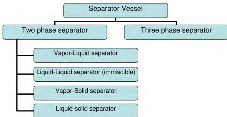
รูปที่ 1 เครื่องกำจัดไอหรืออากาศของไหล 2 สถานะ และของไหล 3 สถานะ
