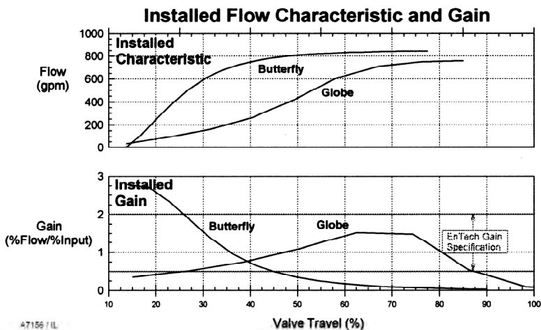
รูปที่ 4-33 ความสัมพันธ์ระหว่าง Installed Flow Characteristic กับ Installed Gain ของ Butterfly Valve และ Globe Valve
