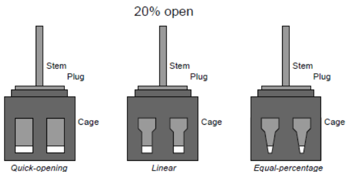
รูปที่ 4-38 ชนิดของตัวนำร่องการเคลื่อนที่หรือตัวประกอบลิ้นวาล์วที่เรียกว่า กรง (Cage) ที่ก่อให้เกิด Flow Characteristic ต่างกันใน Globe Valve
