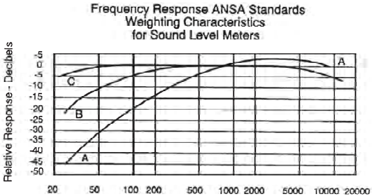
รูปที่ 4-72 กราฟเดซิเบล ในหน่วยวัด dBA, dBB และ dBC
