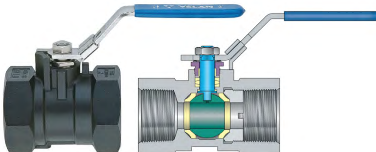
รูปที่ 3-43 One-piece Reduced Port
