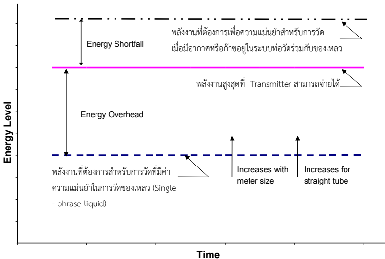
รูปที่ 12 ระดับพลังงานที่จ่ายได้ของตัวถ่ายทอดสัญญาณ (Transmitter) เทียบกับเวลา
