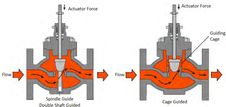
รูปที่ 3-29 การออกแบบการประกอบลิ้นวาล์วที่ใช้แกนที่ความดันสูง
