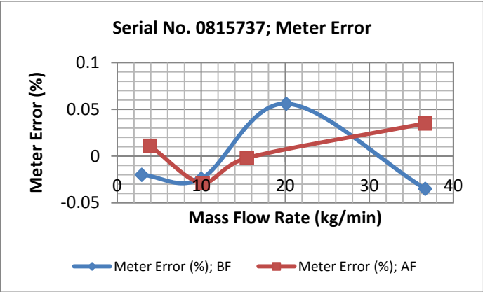
รูปที่ 36 สมรรถนะของมาตรวัดมวลคอริออริสหมายเลข 6680-014-002-51 (SN 0815737)
