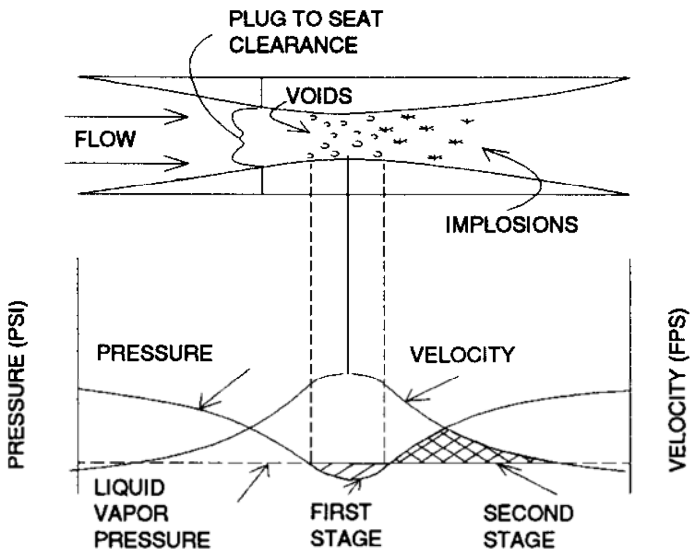
รูปที่ 4-42 ปรากฏการณ์ Cavitation ขั้นตอนที่ 1 (First Stage) และ ขั้นตอนที่ 2 (Second Stage)
