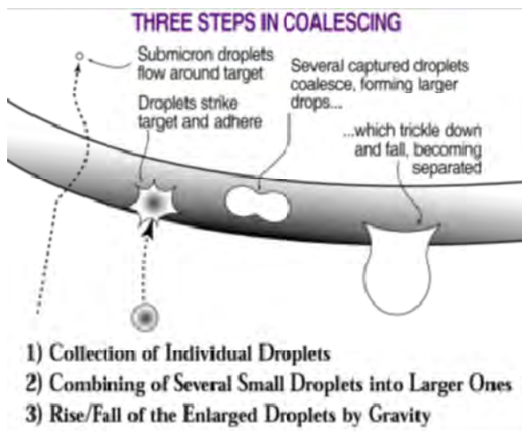
รูปที่ 13 ขั้นตอนการกระทบตามหลักการทำงาน “Impingement”
