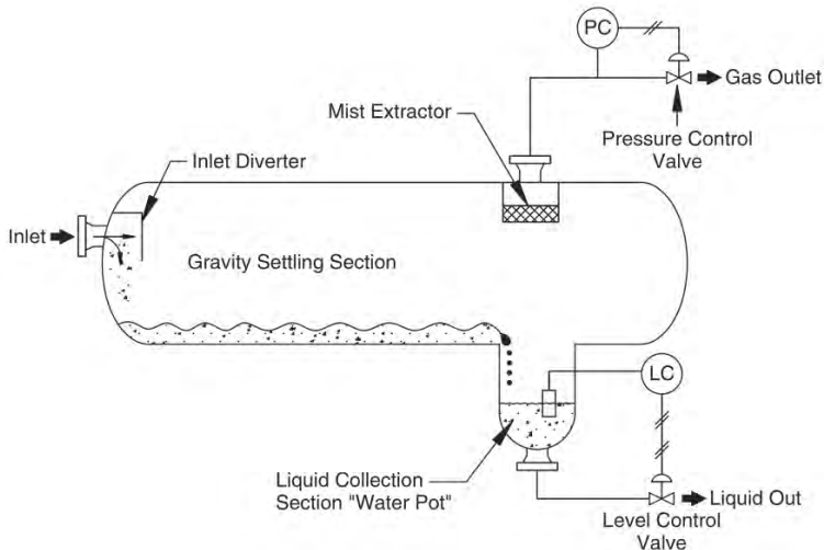
รูปที่ 29 เครื่องกำจัดไอหรืออากาศแบบ Horizontal Separator with a Boot or Water Pot
