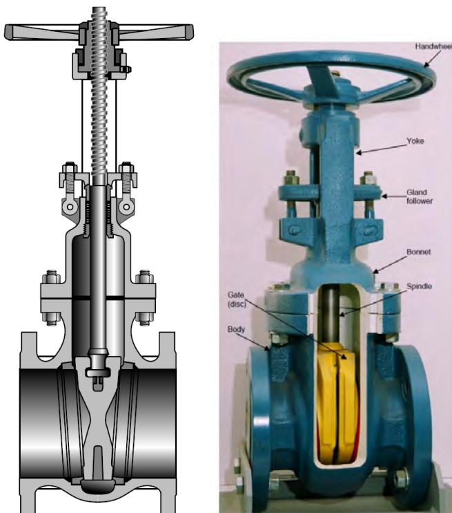
รูปที่ 3-12 วาล์วที่มีลิ้นวาล์วแบบ Flex Wedge,
