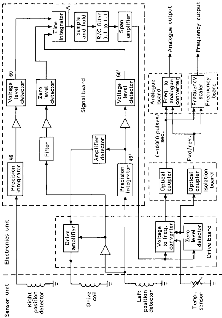
รูปที่ 21-1 Micro Motion Signal Processing System
