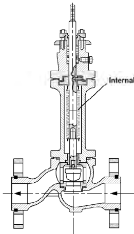
ข. Bellows Seal Bonnet รูปที่ 2-4 ตัวอย่างการออกแบบ Bonnet
