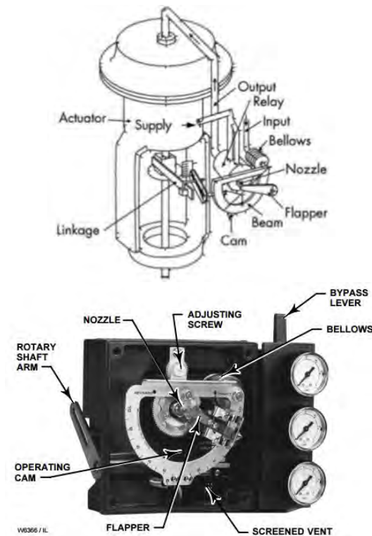
รูปที่ 6-29 ตัวอย่าง Motion Balance Positioner
