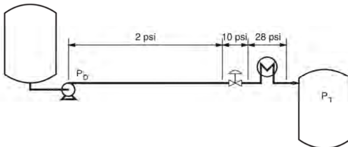
รูปที่ 4-16 ตัวอย่างระบบหรือกระบวนการที่มีสัดส่วนค่าความดันตกคร่อมของทั้งระบบที่ติดตั้งวาล์วมีค่าสูงมากเมื่อเทียบกับค่าความดันตกคร่อมวาล์ว
