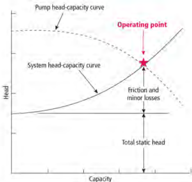
รูปที่ 4-25 “Operating Point” ของระบบท่อในกระบวนการหนึ่ง
