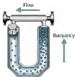
รูปที่ 21 ทิศทางการติดตั้ง มาตรวัดมวลคอโรอริสเพื่อลดการสะสมของ ฟองอากาศ
