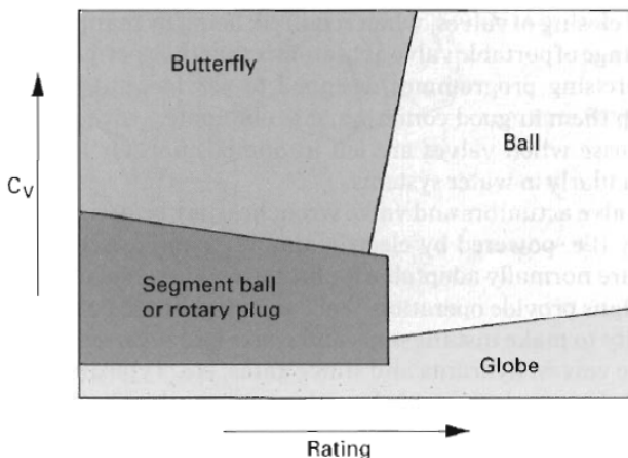
รูปที่ 5-5 ความสัมพันธ์โดยภาพรวมตามชนิดวาล์วควบคุมกับค่า C_v
