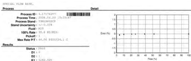
รูปที่ 44 ตัวอย่างการทดสอบมาตรวัดมวลคอริออริสรุ่น CNG050S ผลดัง ในรูปที่ 45
