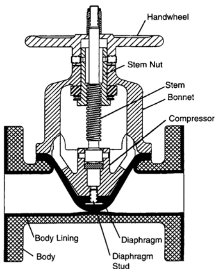
รูปที่ 3-30 ส่วนประกอบหลักๆ ของ Straight-Through Diaphragm Valve
