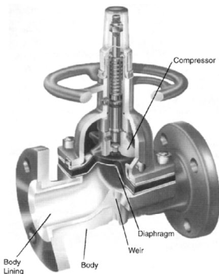
รูปที่ 3-31 ส่วนประกอบหลักๆ ของ Weir Diaphragm Valve
