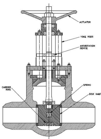
รูปที่ 3-14 ลิ้นวาล์วแบบ Parallel Disk Gate Valve
