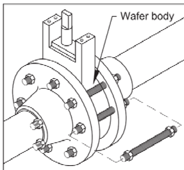
รูปที่ 3-60 Wafer-type Butterfly Valve
