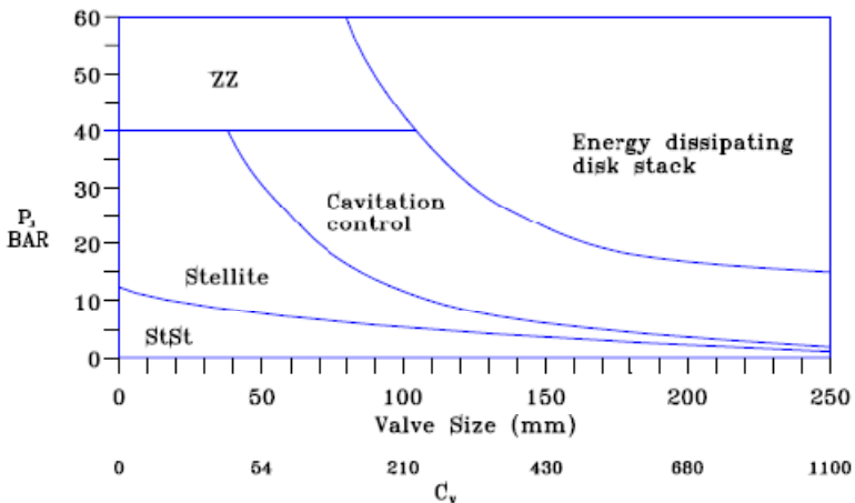
รูปที่ 4-70 แนวการควบคุม Cavitation จากกราฟความสัมพันธ์โดยภาพรวมระหว่าง C_v กับความดันทางเข้าวาล์ว P_1
