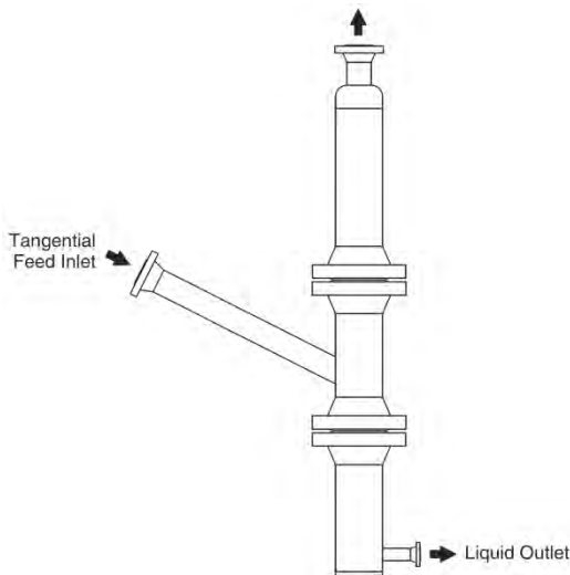
รูปที่ 26 เครื่องกำจัดไอน้ำหรืออากาศแบบใช้แรงหนีศูนย์กลาง
