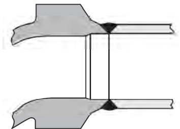
รูปที่ 2-15 ข้อต่อเชื่อมวาล์วแบบ Buttweld Connection
