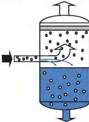
รูปที่ 4 ผลกระทบของความเร็วของไหลของท่อทางเข้าเครื่องกำจัดไอหรือ อากาศต่อการแยกของเหลวออกมาจากของไหล 2 สถานะ
