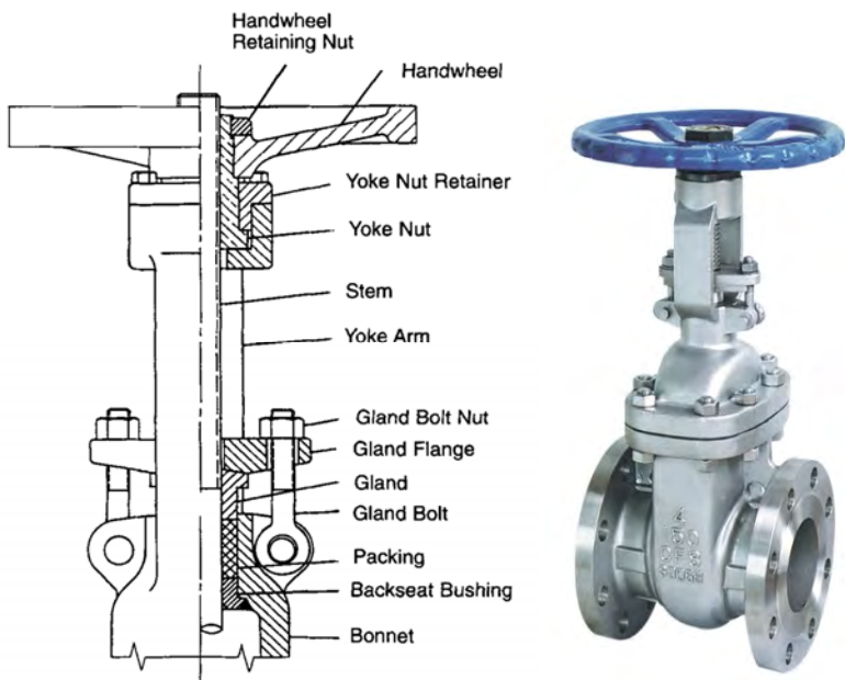
รูปที่ 3-9 Outside Screw and Yoke (OS&Y) Design, บริเวณส่วน Yoke
