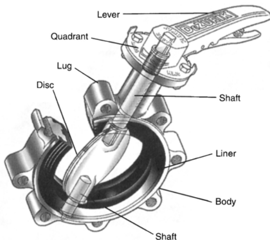
รูปที่ 3-51 Line Butterfly Valve
