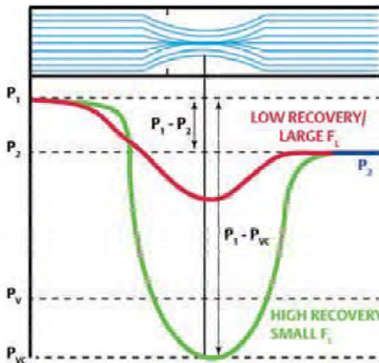
รูปที่ 4-59 เปรียบเทียบการไหลของเหลวของวาล์วฟื้นตัวความดันสูงจะมีค่า F_L ต่ำ, วาล์วฟื้นตัวความดันต่ำจะมีค่า F_L สูง
