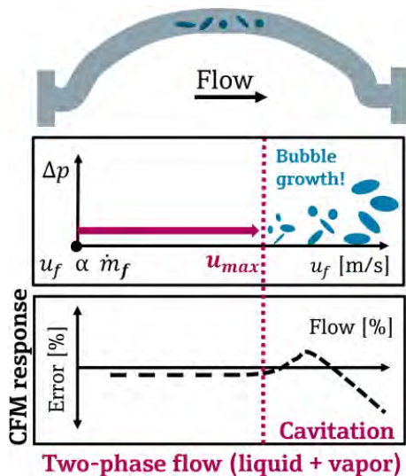
รูปที่ 29 ความเร็วของของเหลวภายในท่อวัดที่สูงมากเกินไปจนความเร็วสูงสุดค่าหนึ่ง ( u_{max} ) จะทำให้ของเหลวเกิดปรากฏการณ์ Cavitation
