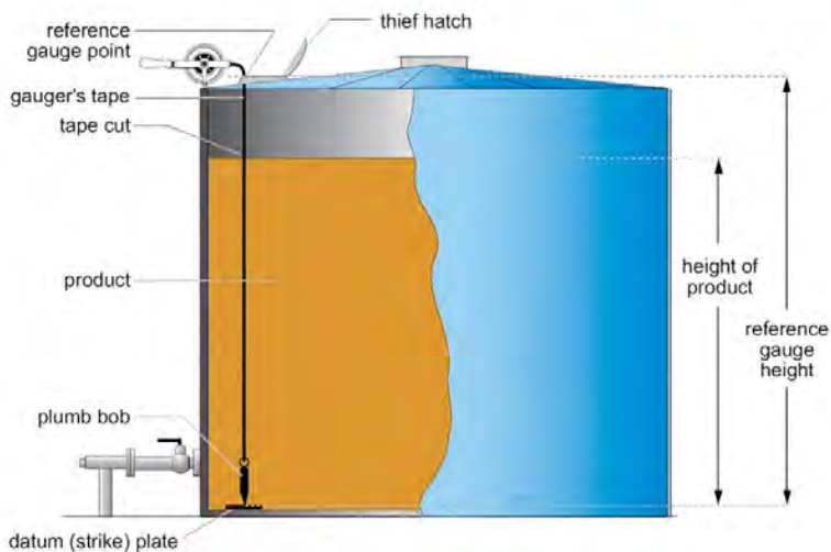
รูปที่ 12 ระยะต่างๆ ของการวัดระดับของเหลวภายในถังสำรองฯแบบ INNAGE Method
