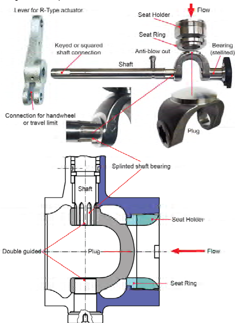
รูปที่ 3-68 Rotary Plug ในรูปแบบของ Eccentric Plug
