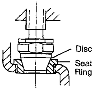
รูปที่ 3-25 ลิ้นวาล์วแบบ Conical Seat
