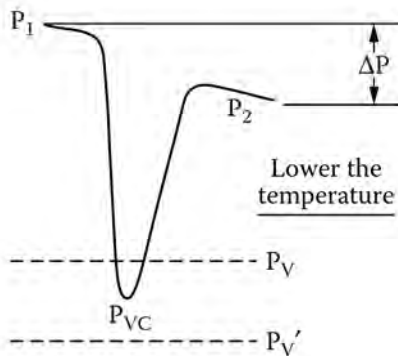
รูปที่ 4-64 ติดตั้งวาล์วหลัง Heat Exchanger ของเหลวด้านทางออกมีอุณหภูมิ ต่ำลง ความดันไอก็ลดต่ำลง
