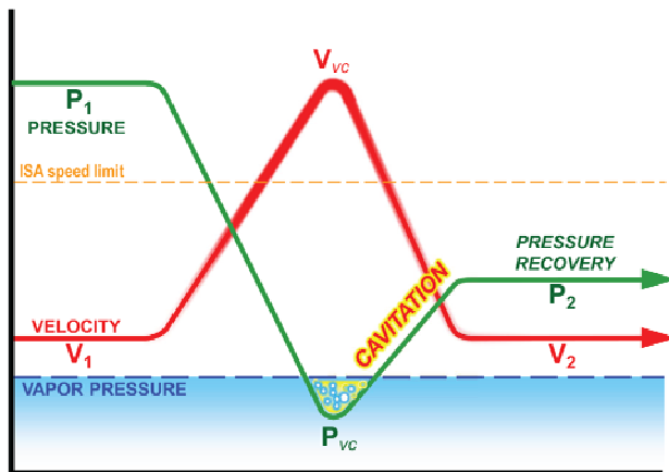
รูปที่ 4-41 ความสัมพันธ์ระหว่างความเร็วของไหลและความดันอธิบายด้วย Bernoulli's Equation ในปรากฏการณ์ Cavitation ตรงตำแหน่ง Vena Contracta
