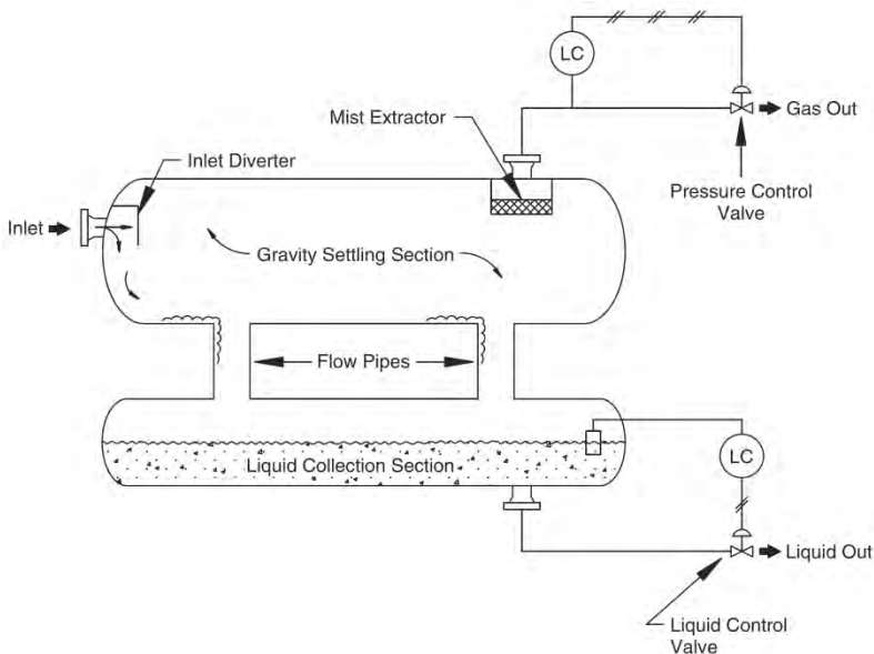
รูปที่ 27 เครื่องกำจัดไอหรืออากาศแบบ Double-Barrel Horizontal Separators
