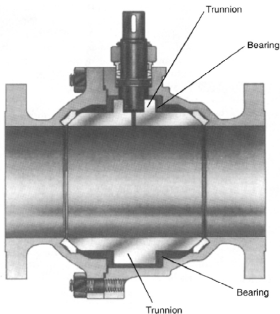
รูปที่ 3-47 Trunnion-mounted Ball Design
