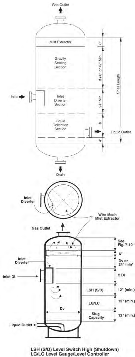
รูปที่ 39 สรุปภาพรวมความสูงและระยะของระดับต่างๆ ในเครื่อง กำจัดไอน้ำหรืออากาศแบบแนวตั้ง (อีกแบบ)
