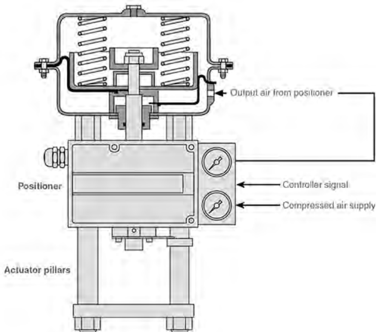
รูปที่ 6-30 สัญญาณความดันอากาศจากตัวควบคุมไปยัง Positioner ซึ่งขยายสัญญาณความดันอากาศแล้วส่งแรงดันอากาศไปขับเคลื่อน Actuator
