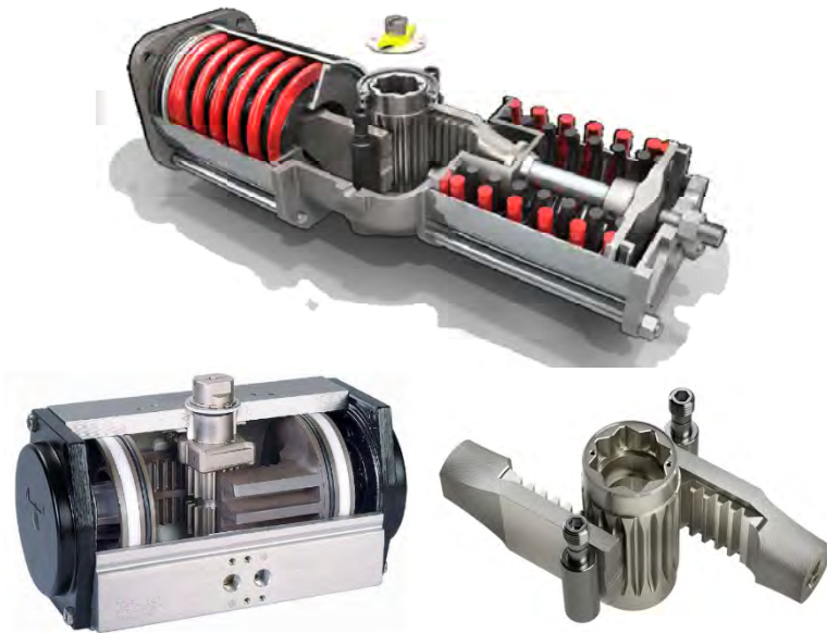
รูปที่ 6-22 ระบบ Rack and Pinion
