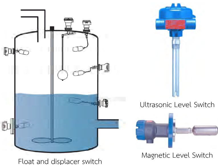
รูปที่ 7 Single-point Level Detection ภายในถังสำรองฯ
