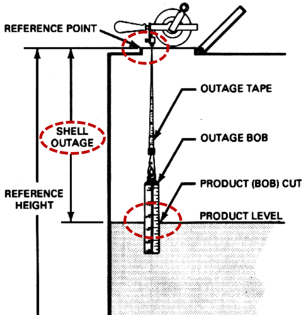
รูปที่ 15 วิธีการวัดแบบ Outage Gauging หรือ Ullage Gauging ด้วย Sounding Tape
