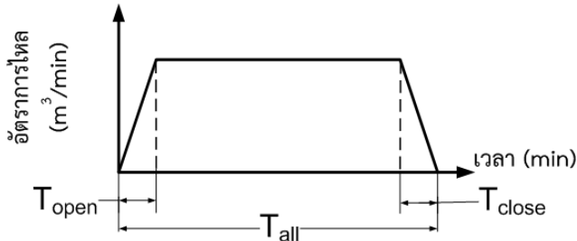
รูปที่ 7 รูปแบบอัตราการไหลเทียบกับเวลาของมาตรวัดแบบมาตรา (ทางปฏิบัติ)
