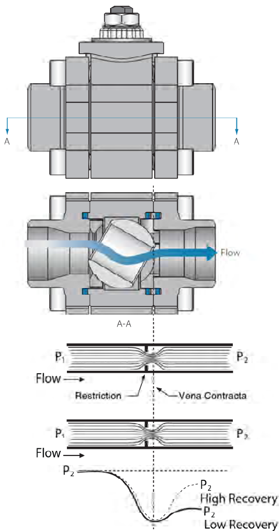
รูปที่ 4-61 ตัวอย่างการฟื้นตัวความดันสูงของ Ball Valve
