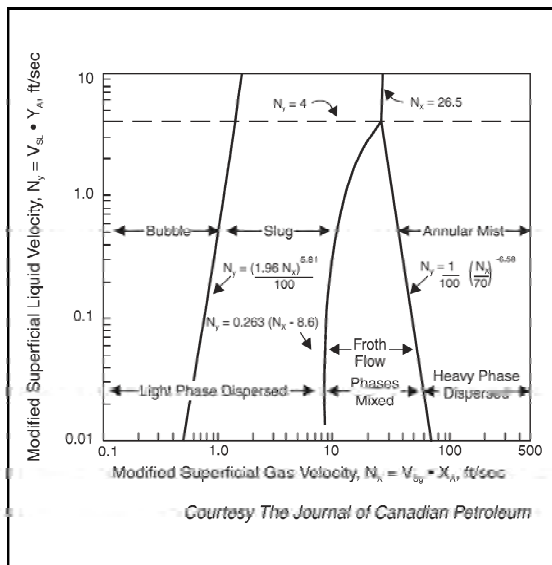
รูปที่ 6 Vertical Flow Pattern Map (Aziz, K 1972)
