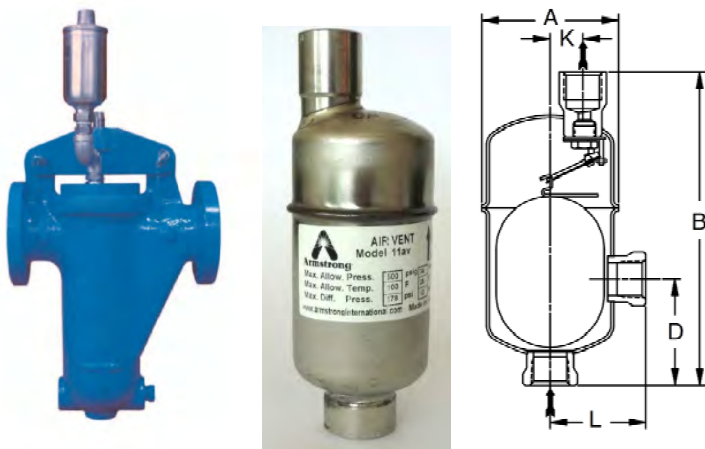
รูปที่ 6 Basket Strainer พร้อมติดตั้ง Automatic Air Vent Valve
