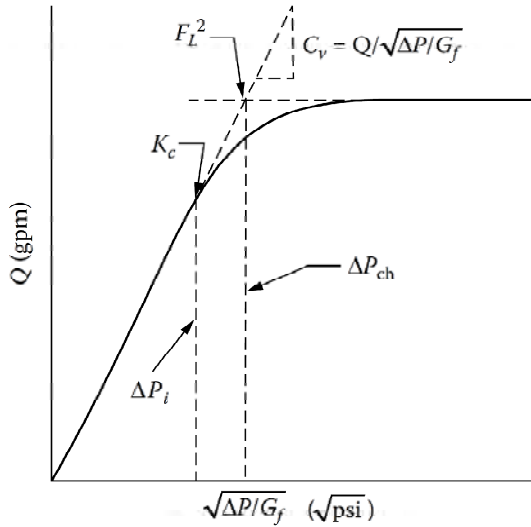
รูปที่ 5-3 Choked Pressure Drop ( \Delta P_{ch} )
