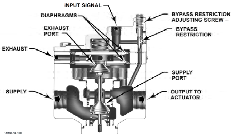
รูปที่ 6-41 Volume Boosters
