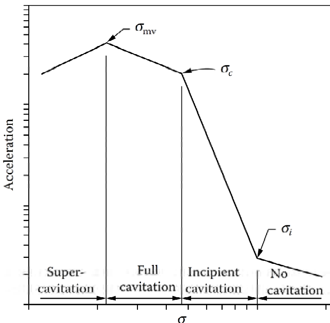
รูปที่ 4-51 การแบ่งปรากฏการณ์การเกิด Cavitation ในวาล์วควบคุม
