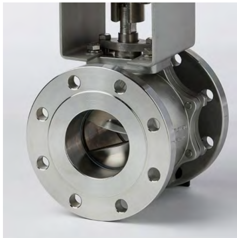
รูปที่ 3-45 V-Port Ball Valve
