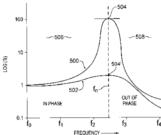
รูปที่ 13 กราฟความสัมพันธ์ระหว่างค่า Transmissivity กับ ความถี่ของการสั้นของท่อวัด เมื่อของเหลวภายในท่อวัดเป็นของเหลวล้นกับของเหลวผสมอากาศหรือก๊าซ
