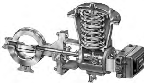
รูปที่ 6-20 Electrical Actuator ติดตั้ง Spring เสริมการทำงาน
