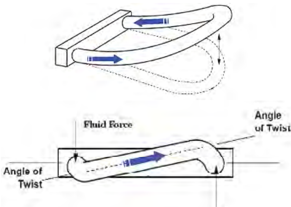
รูปที่ 5 หลักการทำงานของมาตรวัดมวลคอริโอลิส
