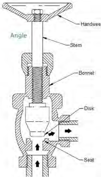
รูปที่ 3-19 Angle Body Design, Globe Valve
