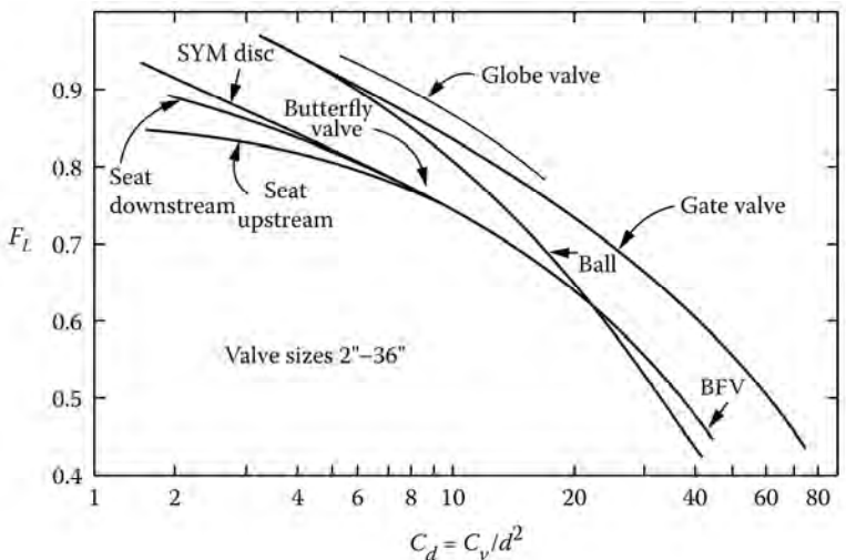
รูปที่ 5-11 F_L มีหลายค่าขึ้นอยู่กับการออกแบบวาล์วในแต่ละชนิด
