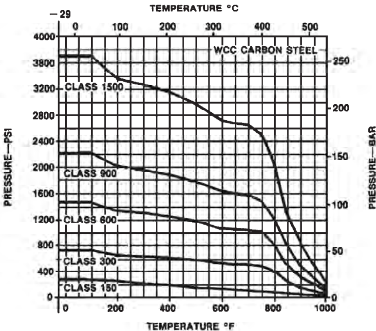
รูปที่ 2-18 Pressure-Temperature Rating สำหรับ Carbon steel (Fisher control instrument, Inc.)
