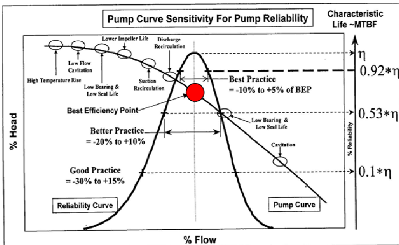
รูปที่ 4-23 Pump Curve Sensitivity For Pump Reliability
