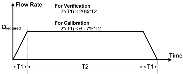
รูปที่ 12 รูปแบบอัตราการไหลเทียบกับเวลาของมาตรวัดแบบมาตรา (ทางปฏิบัติ)
