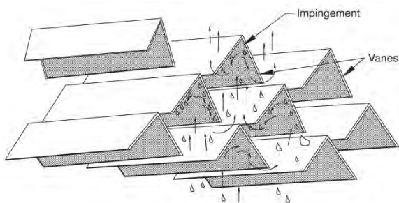
รูปที่ 16 อีกรูปแบบหนึ่งของ Vane-Type Mist Extractor
