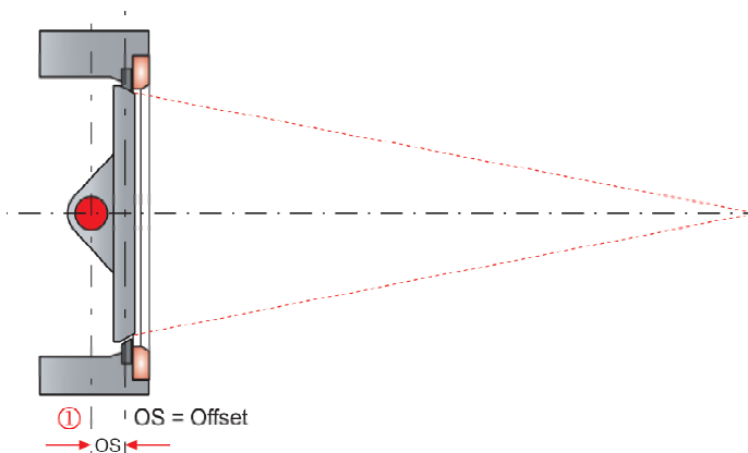
รูปที่ 3-56 การเอียงศูนย์ของลิ้นวาล์ว 1 ระยะเอียง (Single Eccentric Bearing of the Butterfly Disc)
