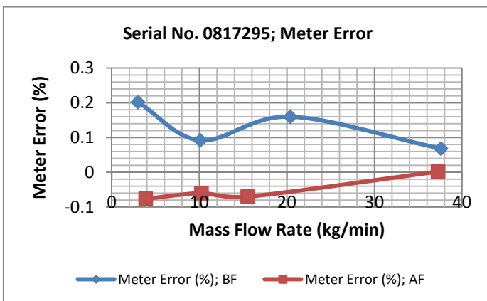
รูปที่ 39 สมรรถนะของมาตรวัดมวลคอริออริสหมายเลข 6680-014-005-51 (SN 0817295)
