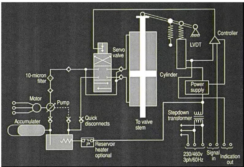
รูปที่ 6-16 Electro- Hydraulic Actuator
