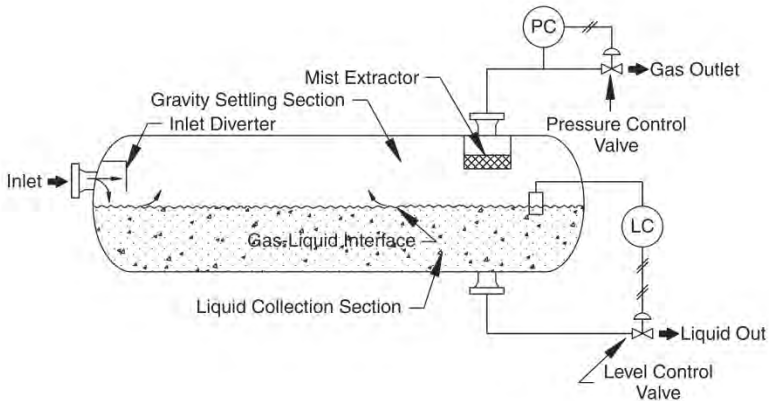
รูปที่ 20 เครื่องกำจัดไอหรืออากาศแบบแนวนอน
