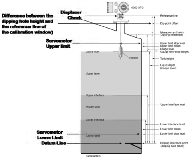
รูปที่ 5 ลักษณะการติดตั้งและค่าระยะของเครื่องวัดระดับของเหลวภายในถัง สำหรับชนิด Servo Operated Displacer Level Gauge
