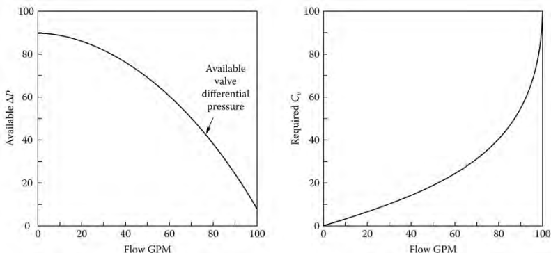
รูปที่ 5-4 ความสัมพันธ์ระหว่าง C_v กับความดันตกคร่อมของวาล์วในระบบ
