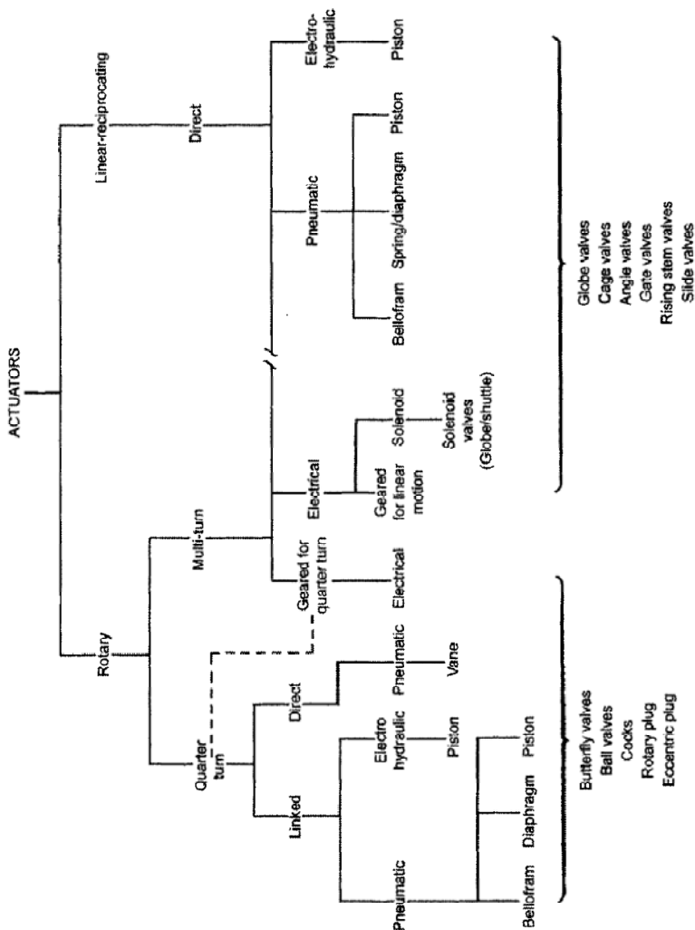
รูปที่ 6-1 ชนิด Actuators หรือ “หัวขับเคลื่อน” และการนำไปใช้งาน
