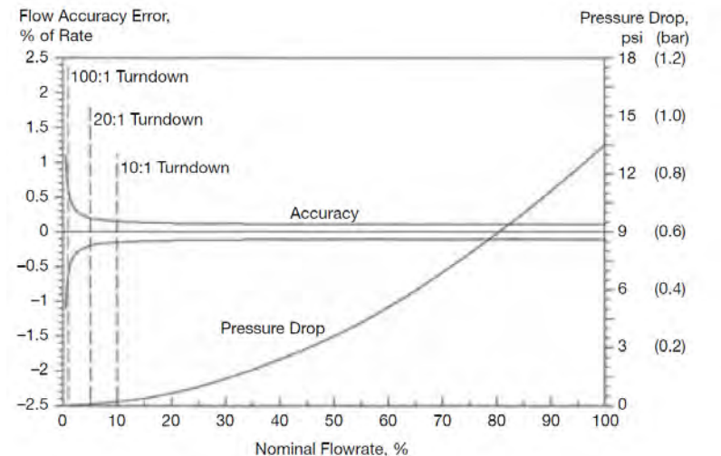
รูปที่ 23 Performance Curve และ Pressure Drop ของมาตรวัดมวลคอริออริส
