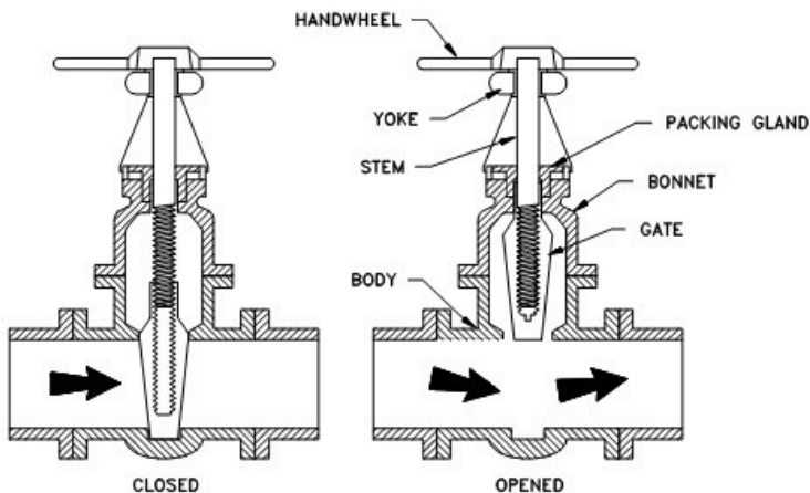
รูปที่ 3-8 ก้านวาล์วแบบ Non-Rising Stem (NRS) Design, Gate Valve
