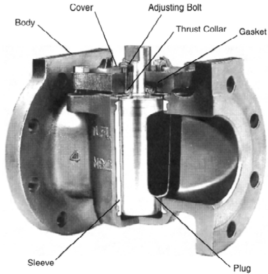
รูปที่ 3-64 Sleeved Plug Valve
