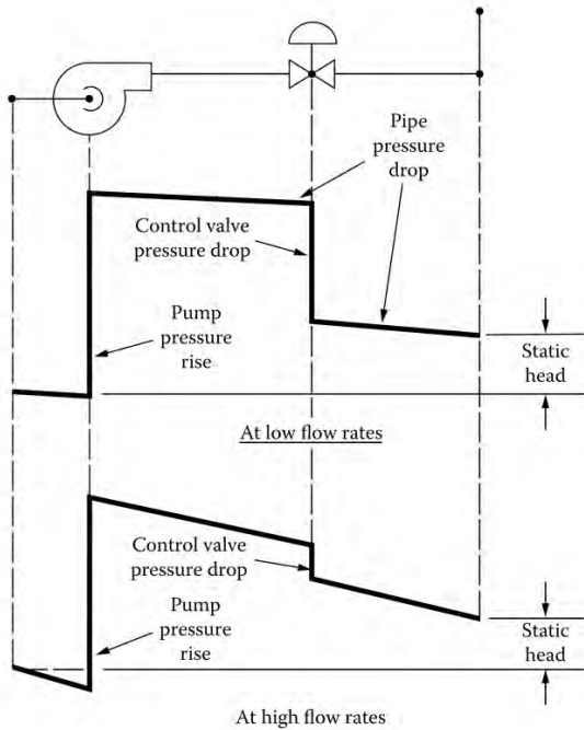
รูปที่ 5-2 ความดันของระบบปั๊มที่อัตราการไหลสูง/อัตราการไหลต่ำซึ่งมีผลต่อการเลือกใช้ค่าความดันตกคร่อมวาล์วในการคำนวณหาขนาดวาล์วควบคุม
