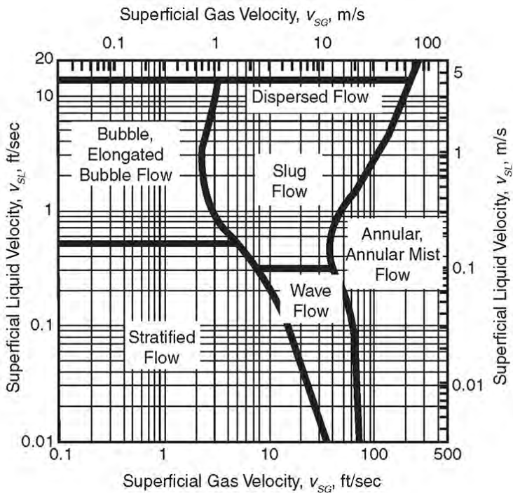
รูปที่ 3 Horizontal Flow Pattern Map (Mandhane 1974)
