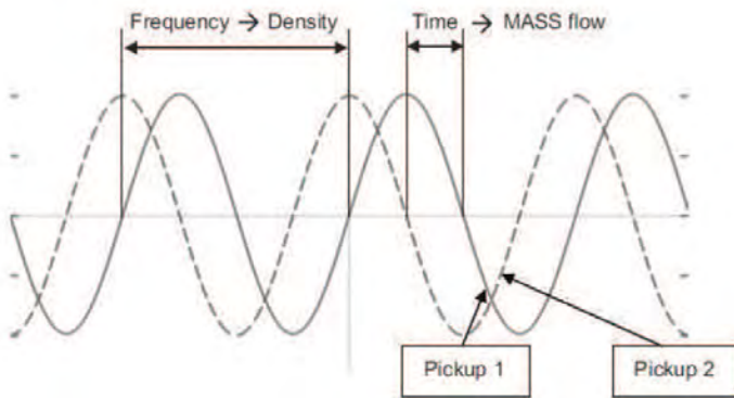
รูปที่ 6 สัญญาณจากตัวตรวจจับการเคลื่อนที่ Sensor's Pickoffs (PO)
