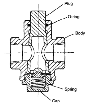
รูปที่ 3-62 ลักษณะ Plug Cock แบบดั้งเดิม
