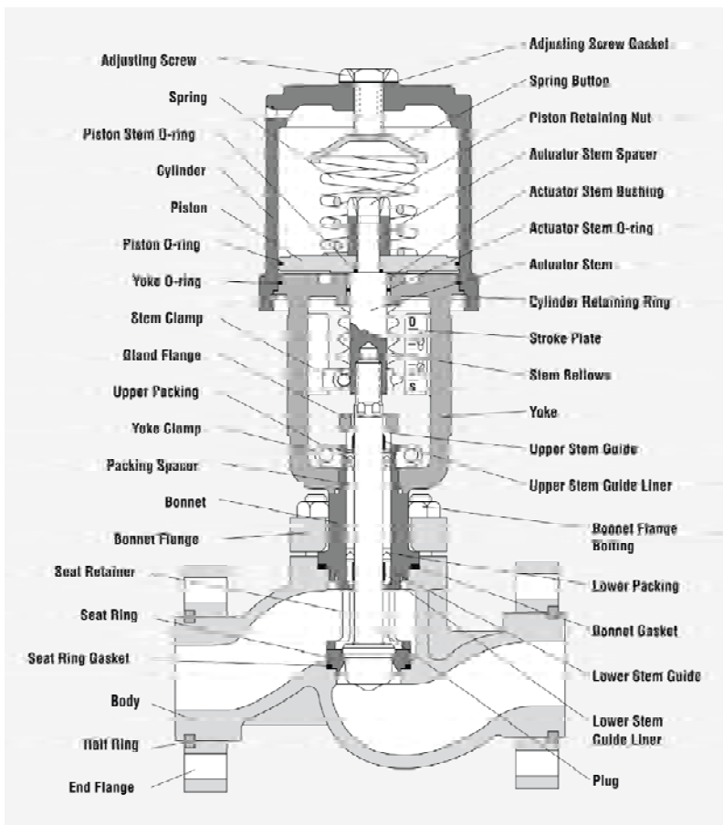
รูปที่ 6-10 ชิ้นส่วน Piston-Cylinder Actuator ที่ติดตั้งเข้ากับ Globe Valve
