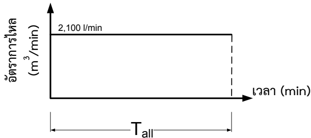
รูปที่ 6 รูปแบบอัตราการไหลเทียบกับเวลาของมาตรวัดแบบมาตรา (ทางทฤษฎี)
