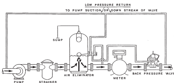
รูปที่ 1 องค์ประกอบที่สำคัญของระบบการวัดปริมาณของเหลว
