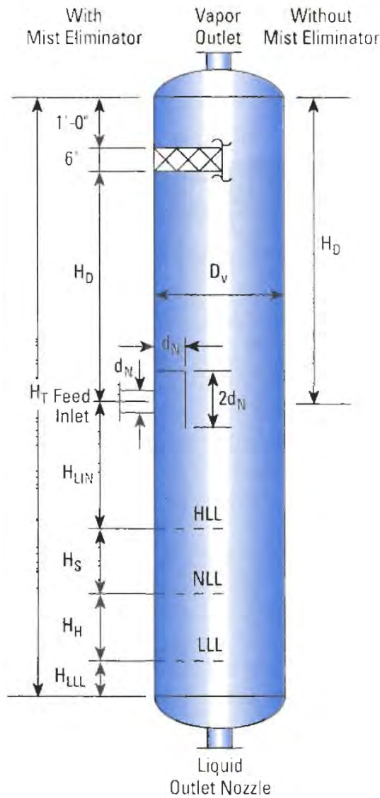
รูปที่ 38 สรุปรวมความสูงและระยะของระดับต่างๆ ในเครื่องกำจัดไอน้ำหรืออากาศแบบแนวตั้ง
