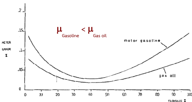
รูปที่ 5 กราฟสมรรถนะของมาตรวัด ชนิด PD Meter
