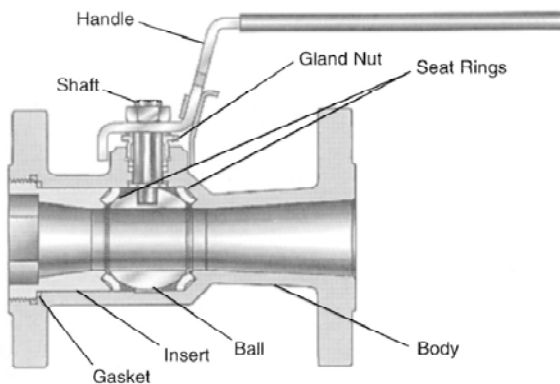
รูปที่ 3-38 End Entry Design ของ Ball Valve
