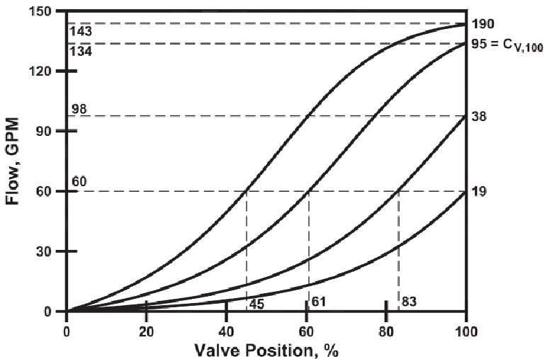
รูปที่ 4-15 ตัวอย่างผลกระทบจากการเลือกใช้วาล์วลักษณะ Equal-Percentage Flow Characteristic ที่มีขนาดเกินพอดีในระบบหรือกระบวนการที่มีสัดส่วนค่าความดันตกคร่อมวาล์วมีค่าสูงมากเมื่อเทียบกับค่าความดันตกคร่อมของทั้งระบบที่ทำการติดตั้ง
