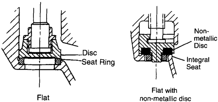
รูปที่ 3-23 ลิ้นวาล์วแบบ Flat seat
