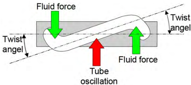
รูปที่ 6 การบิดตัวของท่อดัดอันเนื่องจากโมเมนต์ซึ่งกระทำด้วยแรงคอริออลิสและ ถูกต้านการบิดตัวด้วยโมเมนต์บิดเนื่องจากคุณสมบัติเชิงกลของท่อดัด
