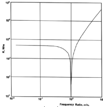
รูปที่ 15 กราฟความสัมพันธ์การสั่นกับ Dynamic Stiffness สมการ (24) ตรงตำแหน่งสุดของกราฟคือค่าความถี่ธรรมชาติของการสั่นระบบมวล
