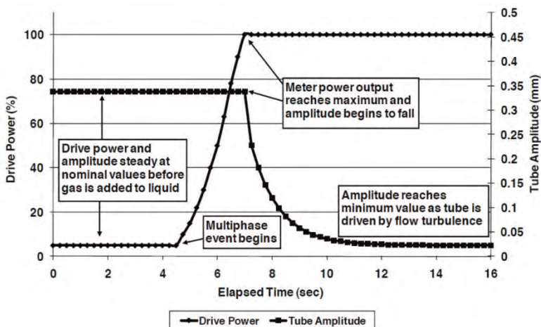
รูปที่ 10 กราฟความสัมพันธ์ระหว่าง Drive Power สูงขึ้นในขณะเดียวกันท่อวัดจะสั่นด้วย Amplitude น้อยลงเมื่อมีอากาศอยู่ในท่อวัดเนื่องจากอากาศจะไปดูดซับการสั่นของท่อวัดให้สั่นน้อยลง
