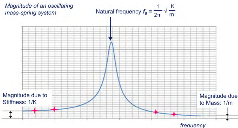
รูปที่ 3 ความถี่ธรรมชาติของการสั่นของท่อดัด (Frequency Response Function; Harmonic Motion)
