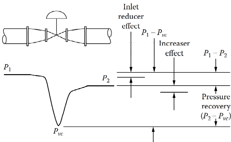
รูปที่ 5-7 รูปแบบความดันของเหลวไหลผ่านวาล์ว
