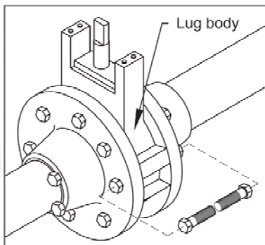
รูปที่ 3-61 Lug-type Butterfly Valve
