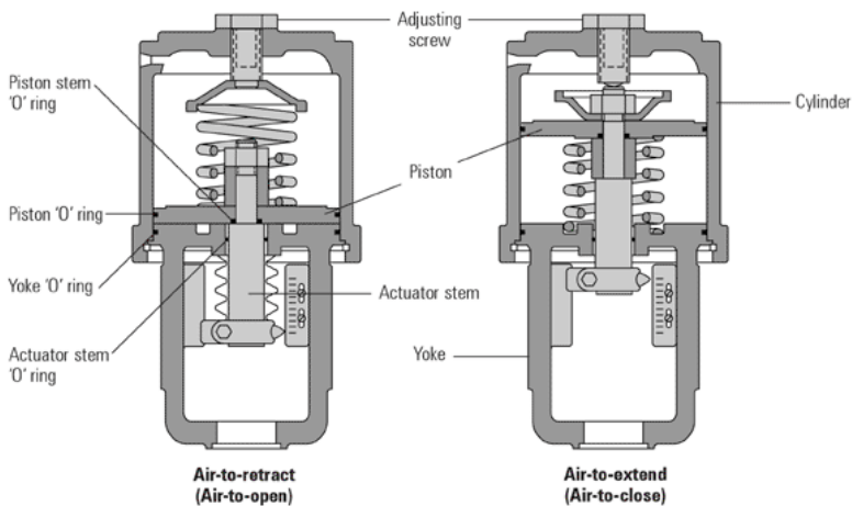
รูปที่ 6-8 รูปแบบโดยทั่วไปของ “Direct-Acting” กับ “Reverse-Acting” ใน Piston-Cylinder Actuator
