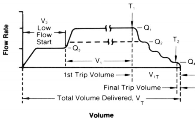
รูปที่ 9 รูปแบบอัตราการไหลเทียบกับเวลาของมาตรวัดที่กำหนดไว้ใน Flow Computer ในการจ่ายน้ำมันทางรถยนต์บรรทุกน้ำมัน
