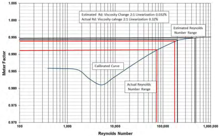
รูปที่ 51 Reynolds Number มีผลต่อ Meter Factor ของมาตรวัดมวลคอริออ- ริสเมื่อสอบเทียบที่ช่วง Reynolds Number หนึ่งแต่กลับไปใช้งานจริง อีกช่วง Reynolds Number หนึ่งซึ่งจะได้ Meter Factor ต่างกัน
