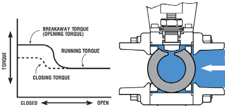
รูปที่ 6-26 แรงบิดที่ต้องใช้ในการปิด-เปิดวาล์วในแต่ละตำแหน่งปิด-เปิด
