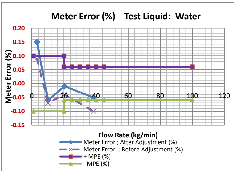
รูปที่ 32 ผลเปรียบเทียบการสอบเทียบมาตรวัดมวลคอริออริส Model CNG050S ด้วยค่า K-Factor 60 pulses/kg (Before Adjustment) กับค่า K-Factor 500 pulses/kg (After Adjustment)
