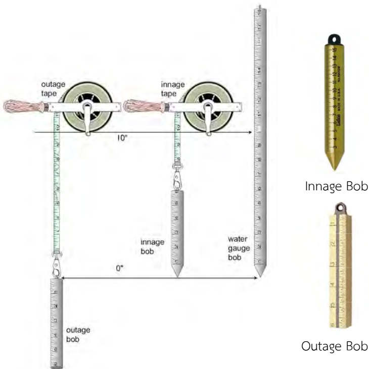
รูปที่ 16 Bob หรือลูกดิ่งแบบ Innage Bob และแบบ Outage Bob
