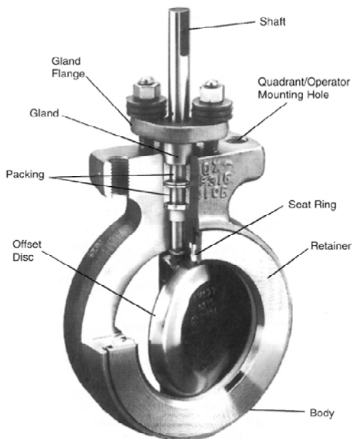
รูปที่ 3-55 High-performance Butterfly Valve
