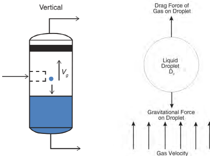
รูปที่ 32 สภาวะแรงกระทำต่อหยดของเหลว (Droplets) ที่ผสมอยู่ในของไหล 2 สถานะในส่วนที่เป็นก๊าซภายในเครื่องกำจัดไอหรืออากาศ
