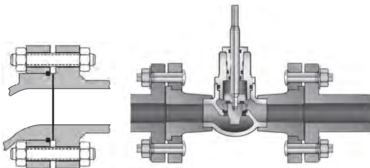
รูปที่ 2-10 ข้อต่อหน้าแปลนแบบ “Separable Flange”
