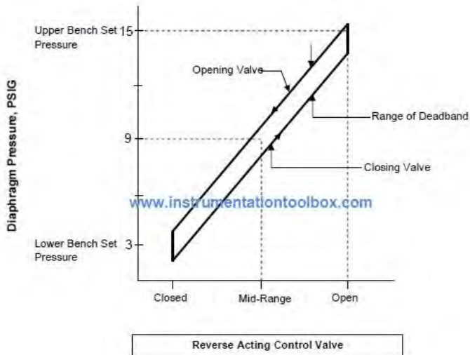
รูปที่ 6-6 Dead Band ของ Actuator
