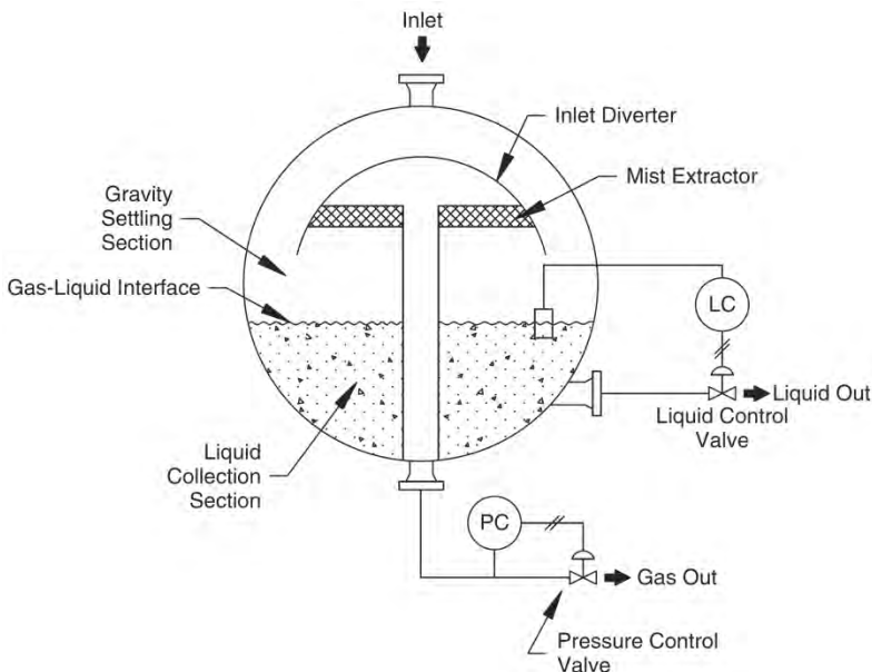
รูปที่ 25 เครื่องกำจัดไอหรืออากาศแบบทรงกลม
