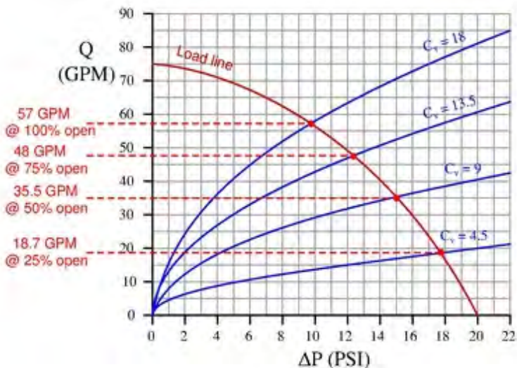
รูปที่ 4-30 ตัวอย่างความดันตกคร่อมวาล์วมีค่าแตกต่างกันเมื่ออัตราการไหลต่างกันด้วยตำแหน่งของลิ้นวาล์วที่แตกต่างกัน
