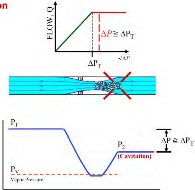
รูปที่ 4-57 การไหลของเหลวเสมือนผ่านวาล์วควบคุม, \Delta P \geq \Delta P_{\text{choked}} (\Delta P_T) , P_{VC} < P_V
