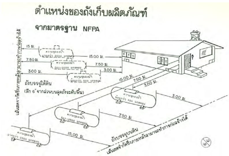
รูปที่ 6 ข้อกำหนด NFPA มาตรฐานความปลอดภัยได้กำหนดการจัดวางถังบรรจุก๊าซความดัน
