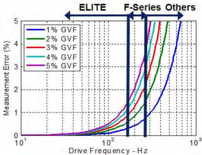
รูปที่ 19 ความสัมพันธ์ Drive Frequency ของท่อวัดกับผลผิดการวัดของมาตรวัดคอโรอริส ขึ้นอยู่กับปริมาณอากาศผสมอยู่ในของเหลว (Gas Void Fraction; GVF) ขณะทำการวัด รุ่น ELITE ถือว่าได้รับผลกระทบน้อยที่สุดจาก GVF
