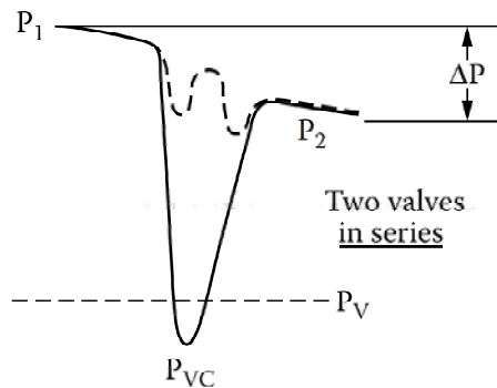
รูปที่ 4-69 ติดตั้งวาล์วที่เหมือนกัน (Identical Valves) 2 ตัวต่อแบบอนุกรม
