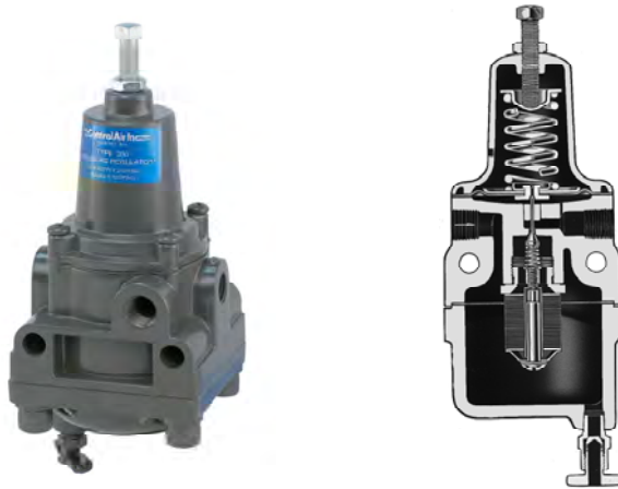
รูปที่ 6-40 Air Regulator
