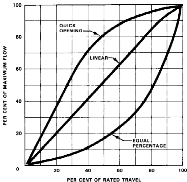
รูปที่ 4-4 Inherent Flow Characteristic
