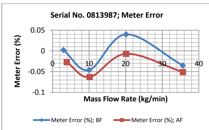
รูปที่ 35 สมรรถนะของมาตรวัดมวลคอริออริสหมายเลข 6680-014-001-51 (SN 0813987)
