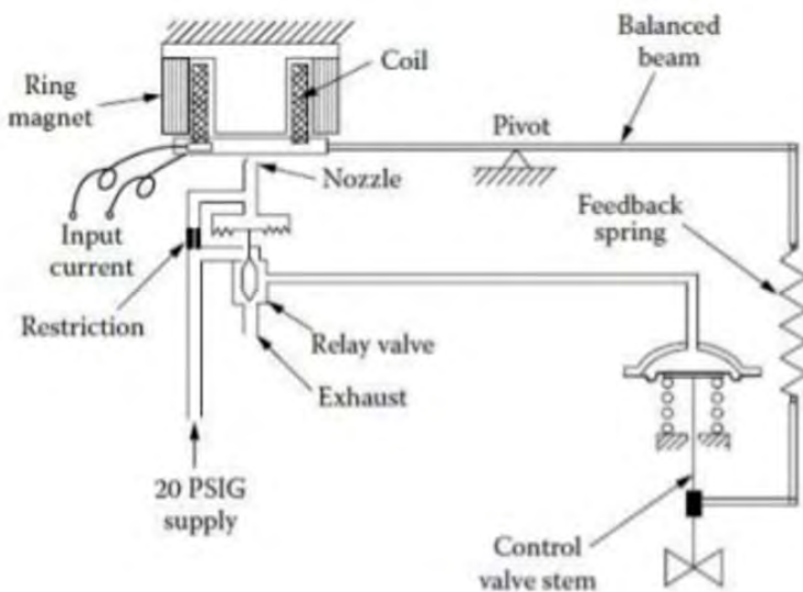
รูปที่ 6-32 หลักการทำงาน Electro-Pneumatic Positioner
