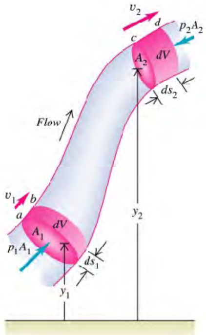
รูปที่ 1 พลังงานที่จุดใดๆในระบบของเหลวภายในท่อตามสมการแบร์นูลลี
