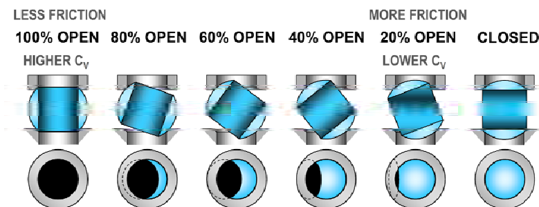
รูปที่ 3-36 รูปแบบการเปิดของลิ้นวาล์วของ Ball Valve
