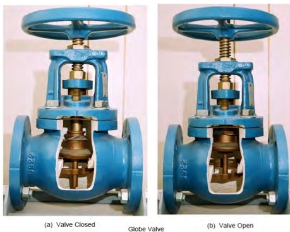
รูปที่ 3-28 ตัวอย่างการประกอบลิ้นวาล์ว (Spindle Guide)
