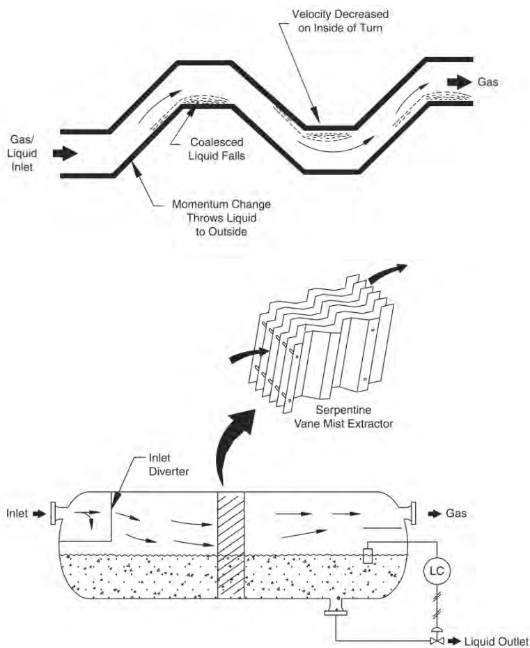
รูปที่ 14 Vane-Type หรือ Chevron-shape mist extractor จับหยดของเหลวได้ขนาด 10-40 \mu\text{m}
