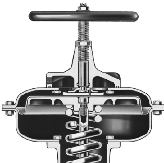
รูปที่ 6-25 การติดตั้ง Top-Mount Handwheel เข้ากับ Diaphragm Actuator
