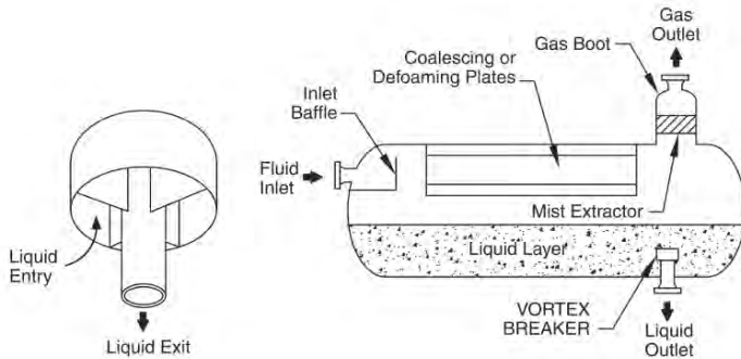
รูปที่ 18 Vortex Breaker
