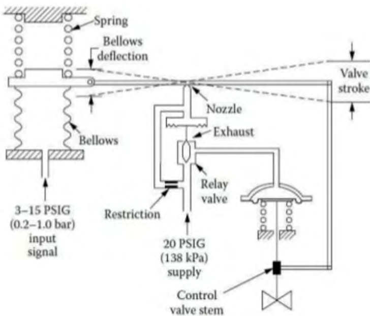
รูปที่ 6-28 หลักการทำงาน Motion Balance Positioner
