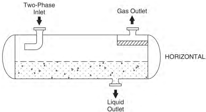
รูปที่ 11 Inlet Device ชนิด Elbow Diverter บางครั้งตัดปลาย Elbow ให้เหลือครึ่งท่อ
