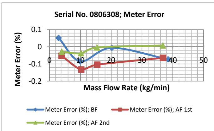
รูปที่ 40 สมรรถนะของมาตรวัดมวลคอริโอลิสหมายเลข 6670-005-001-51 (SN'0806308)
