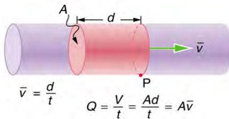
รูปที่ 3 อัตราการไหลของเหลวภายในท่อ
