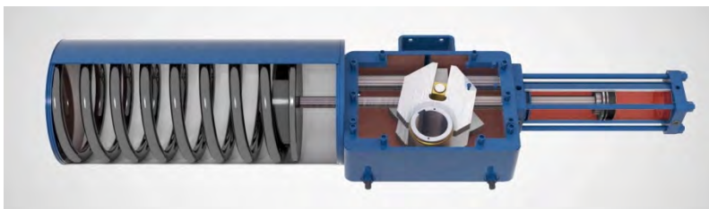
รูปที่ 6-18 รูปตัดขวางแสดงภายใน Hydraulic Actuator
