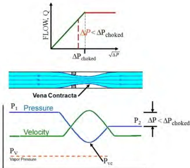
รูปที่ 4-56 การไหลของเหลวเสมือนผ่านวาล์วควบคุม, \Delta P < \Delta P_{\text{choked}} ( \Delta P_T ), P_{VC} > P_v
