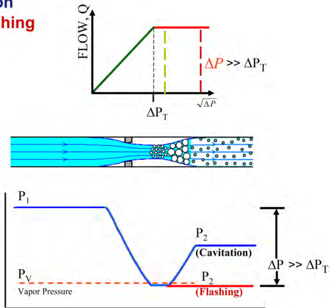
รูปที่ 4-58 การไหลของเหลวเสมือนผ่านวาล์วควบคุม, \Delta P \geq \Delta P_{\text{choked}} (\Delta P_T) ,
