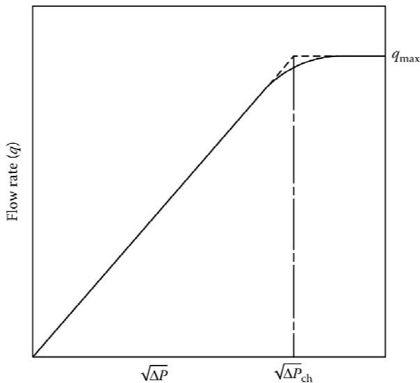
รูปที่ 5-8 อัตราการไหลสูงสุดของเหลวภายใต้ Turbulent Flow, Vaporizing Flow Condition (Choked Flow) ผ่านวาล์ว
