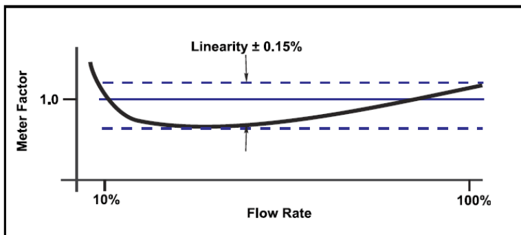
รูปที่ 2 พิจารณาค่า Linearity ของมาตรวัด
