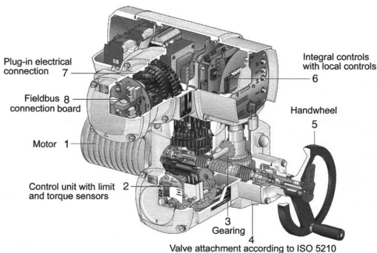
รูปที่ 6-13 Electro-mechanical Actuator แบบหมุนได้หลายรอบ
