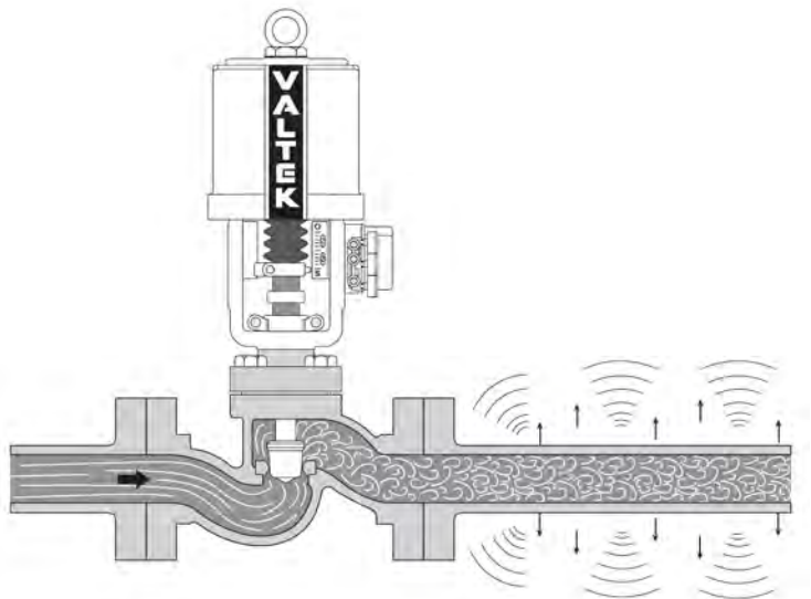
รูปที่ 4-71 ท่อจะสั่นและมีเสียงดังด้านปลายน้ำของวาล์ว
