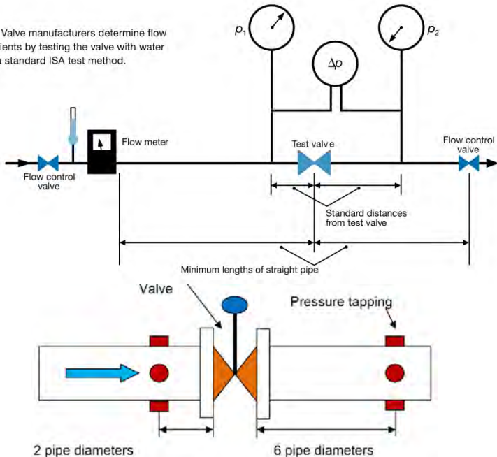
รูปที่ 5-6 ตำแหน่งวัดความดันในการทดสอบหา Valve Flow Coefficient ( C_v )
