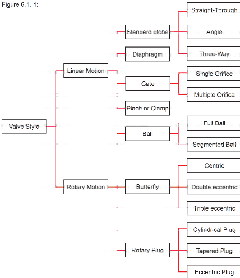
รูปที่ 3-69 การแบ่งรูปแบบของวาล์วที่เราได้เจออีกรูปแบบหนึ่ง
