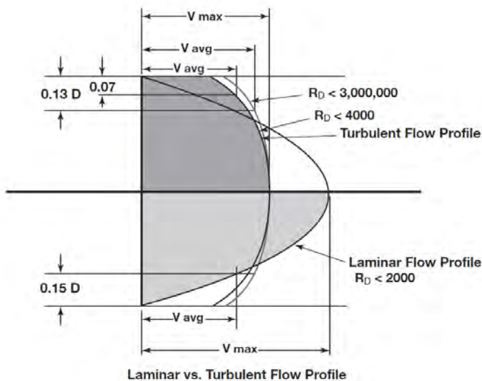
รูปที่ 9 รูปแบบความเร็วของเหลวภายในท่อเทียบกับค่า Reynolds Number
