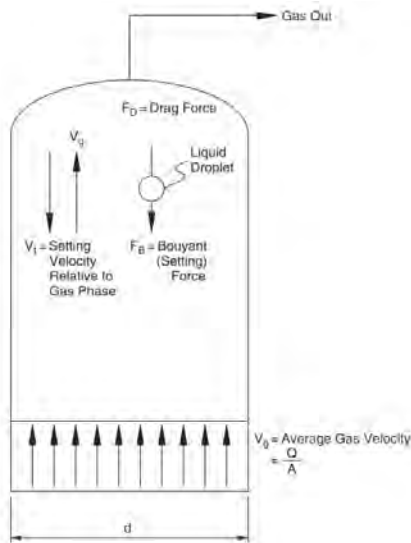
รูปที่ 37 ความสัมพันธ์ของความเร็ว, แรง และพื้นที่หน้าตัดของเครื่อง กำจัดไอหรืออากาศแบบแนวตั้ง
