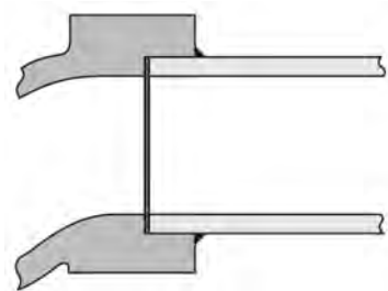
รูปที่ 2-14 ข้อต่อเชื่อมวาล์วแบบ Socketweld End Connection
