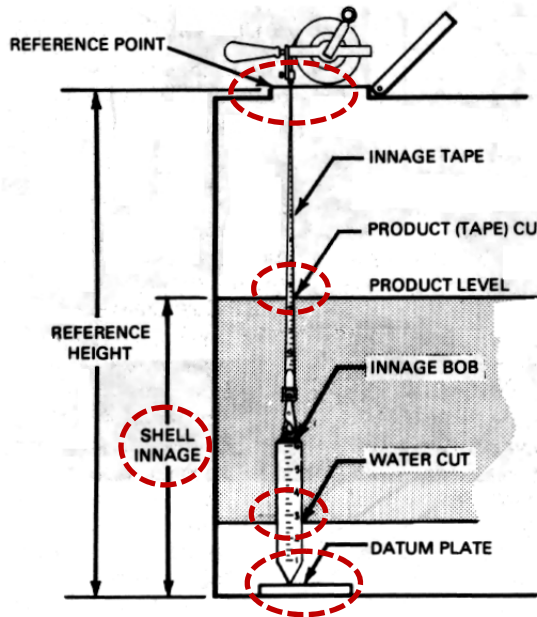
รูปที่ 13 วิธีการวัดแบบ Innage Gauging ด้วย Sounding Tape
