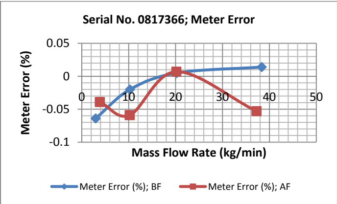
รูปที่ 37 สมรรถนะของมาตรวัดมวลคอริออริสหมายเลข 6680-014-003-51 (SN 0817366)
