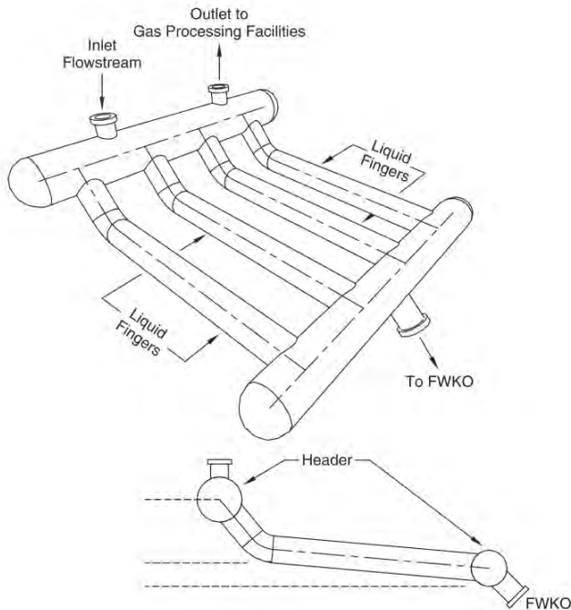
รูปที่ 31 เครื่องกำจัดไอน้ำหรืออากาศแบบ Slug Catchers
