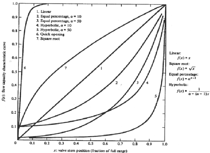
รูปที่ 4-6 Inherent Flow Characteristic ในรูปแบบต่างๆ
