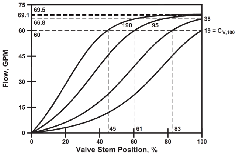
รูปที่ 4-20 ตัวอย่างผลกระทบจากการเลือกใช้วาล์วลักษณะ Equal-Percentage Flow Characteristic ที่มีขนาดเกินพอดีในระบบหรือกระบวนการที่มีสัดส่วนค่าความดันตกคร่อมของทั้งระบบที่ติดตั้งวาล์วมีค่าสูงมากเมื่อเทียบกับค่าความดันตกคร่อมวาล์ว
