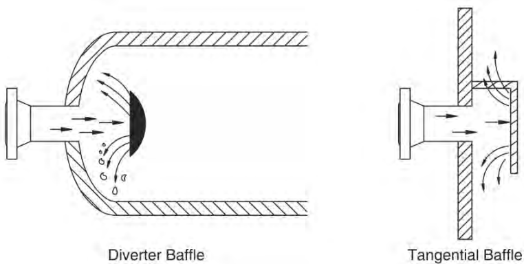
รูปที่ 9 Inlet Device ชนิด Diverter Baffle (Dish head) หรือ Tangential Plate (Diverter Plate)
