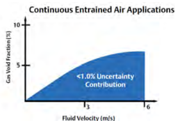
รูปที่ 17 %ปริมาตรของอากาศผสมในของเหลว ที่ยังคงให้ผลการวัดแม่นยำอยู่ ข้อมูลจาก Micro Motion White Paper (WP-00698)
