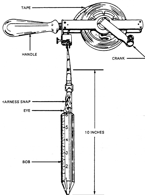
รูปที่ 17 ชื่อชิ้นส่วนประจำสายแถบโลหะประกอบลูกดิ่ง (ต้องเป็นหน่วย IS Unit)
