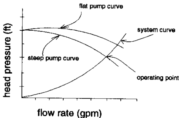
รูปที่ 4-26 จุด System Operating Point ต่างกันหรือเปลี่ยนไปเมื่อเลือกปั๊มต่างชนิดกัน
