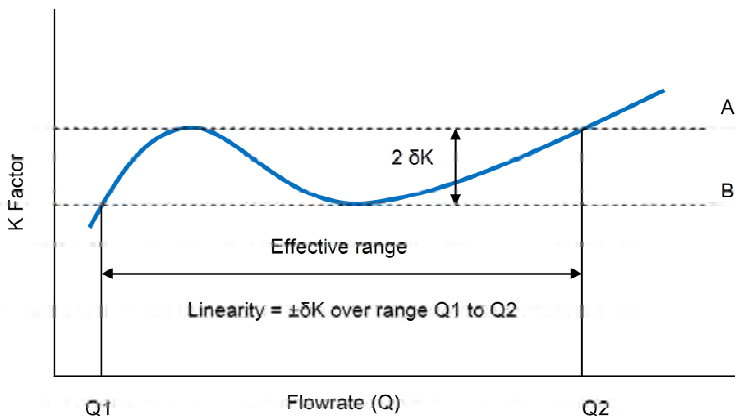
รูปที่ 5 Linearity ของมาตรวัดในเทอมของ K-Factor
