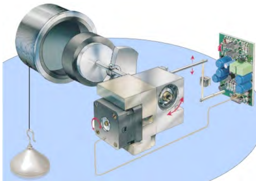
รูปที่ 3 ลูกลอยของเครื่องวัดระดับของเหลวภายในถังสำรองฯ
