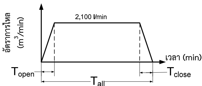
รูปที่ 10 รูปแบบอัตราการไหลเทียบกับเวลาของมาตรวัดแบบมาตรา (ทางปฏิบัติ)
