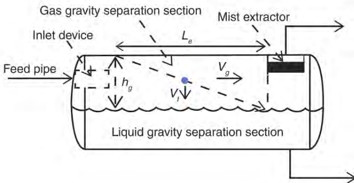
รูปที่ 36 ระยะทางที่เพียงพอให้หยดของเหลวสามารถแยกตัวออกจากก๊าซ เครื่องกำจัดไอหรืออากาศแบบแนวนอนได้ ( L_e ) ก่อนไหลออกจาก เครื่องกำจัดไอหรืออากาศไปพร้อมกับก๊าซ ( H_v = h_g สำหรับใน รูปนี้)
