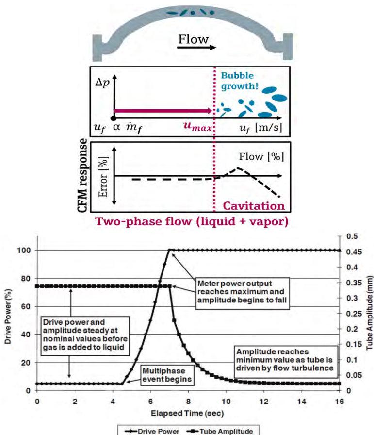
รูปที่ 47 ค่า Drive Gain ของมาตรวัดมวลคอโรริสกับการไหลของเหลวภายในท่อเมื่อเปลี่ยนรูปแบบการไหลจากของเหลวสถานะเดียวเป็นของไหล 2 สถานะคือของเหลวบวกกับไอหรืออากาศ
