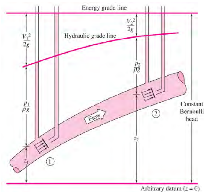
รูปที่ 2 ระดับพลังงานของเหลว (Hydraulic and energy grade lines) ภายในท่อเมื่อเป็นการไหลที่มีแรงเสียดทาน
