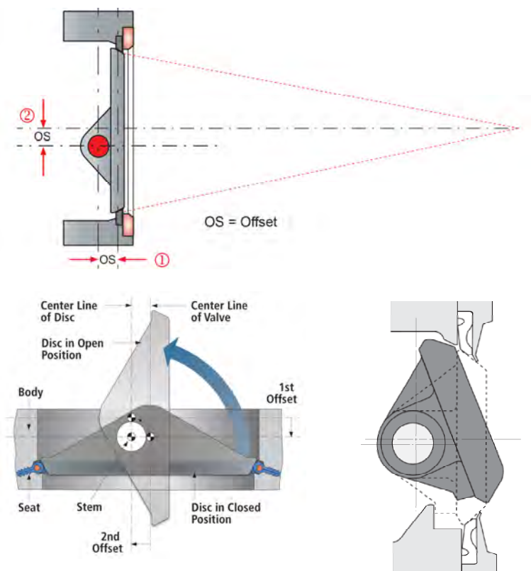
รูปที่ 3-57 การเยื้องศูนย์กลางของลิ้นวาล์ว 2 ระยะเยื้อง (Double Eccentric Bearing of the Butterfly Disc)
