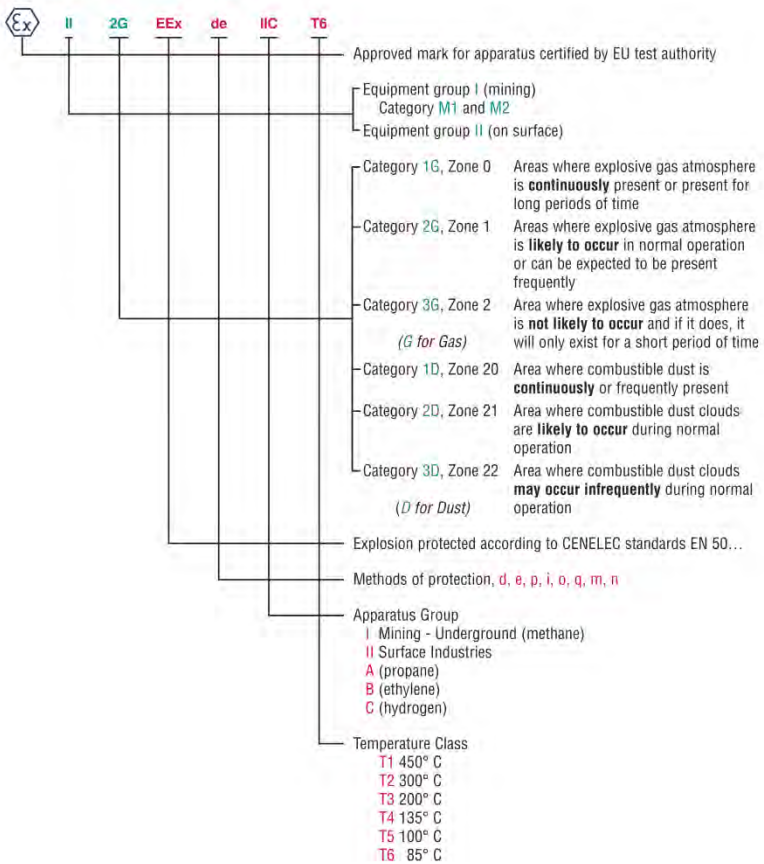
รูปที่ 21-3 ตัวอย่างและความหมายอักษรย่อบนอุปกรณ์ไฟฟ้าที่ใช้ในพื้นที่อันตราย (ต่อ)
