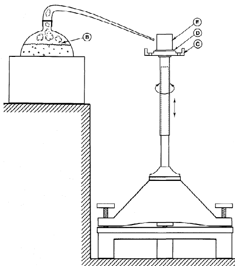
รูปที่ 24 เครื่องมืออุปกรณ์ที่ใช้ล้างตุ้มน้ำหนักแบบมาตรา Platinum-iridium Prototypes (E) ของ BIPM ในยุคหนึ่ง Prototype (E) จะถูกวางไว้บนภาควางตุ้มน้ำหนักแบบมาตราทำด้วย platinum-iridium (D) โดยมีเครื่องผลิตไอน้ำประกอบด้วย Pyrex flask (B) ขนาด 1 ลิตร บรรจุน้ำกลั่น 2 ครั้ง (Bi-Distilled Water) ถูกทำให้ร้อนด้วยเตาไฟฟ้า 350 Watts เพื่อผลิตไอน้ำด้วยอัตรา 0.5 l/h. เมื่อน้ำถูกทำให้ร้อนจนกลายเป็นไอ ไอน้ำจะถูกส่งผ่านท่อที่ปลายท่อทำเป็น Orifice ขนาดเส้นผ่านศูนย์กลางประมาณ 2 มิลลิเมตรพุ่งตรงไปยังตุ้มน้ำหนักแบบมาตรา Platinum-iridium Prototypes (E) โดยระยะห่างระหว่างผิว Prototype (E) กับปลายพ่นไอน้ำห่างกันประมาณ 5 มิลลิเมตรตลอดเวลา น้ำที่กลั่นตัวลงมาจะถูกสะสม ณ ภาควางน้ำ (C) และระบายออกไป ทั้งนี้เราสามารถหมุนภาควางได้ตลอดเวลาและสามารถเลื่อนขึ้นลงได้ 4 ทิศทางด้วยเช่นกัน
