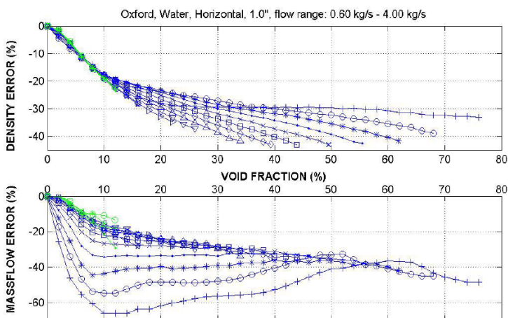
รูปที่ 20 %ปริมาตรของอากาศผสมในของเหลว (% Void Fraction) ที่แตกต่างกันมีผลต่อความแม่นยำในการวัดปริมาณส่งจ่ายและค่าความหนาแน่นที่วัดได้ (Henry M, Duta M, Tombs M, Yeung H, Mattar W, “How a Coriolis Mass Flowmeter Can Operate in Two-Phase (Gas/ Liquid) Flow” ISA EXPO 2004 Technical Conference) (+ อัตราการไหลมวลสูง )
