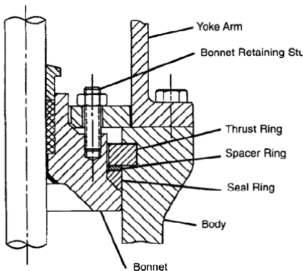
รูปที่ 3-5 Union Body-Bonnet Joint, Gate Valve
