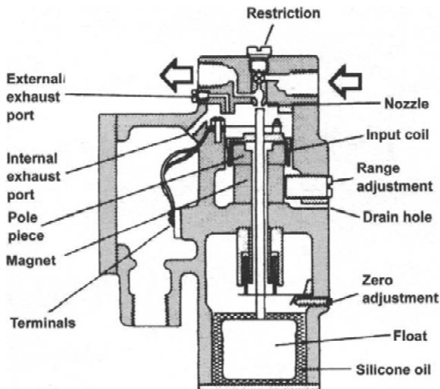
รูปที่ 6-36 I/P Converter
