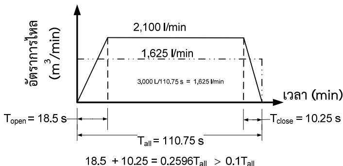
รูปที่ 11 รูปแบบอัตราการไหลเทียบกับเวลาของมาตรวัดแบบมาตราชนิด PD Flowmeter ขนาด \varnothing 4 นิ้ว
