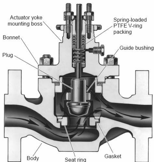
รูปที่ 6-2 โครงสร้างโดยทั่วไปของ Globe Valve
