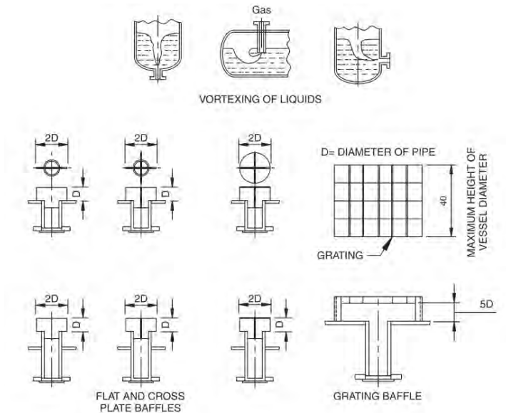
รูปที่ 19 รูปแบบโดยทั่วไปของ Vortex Breaker
