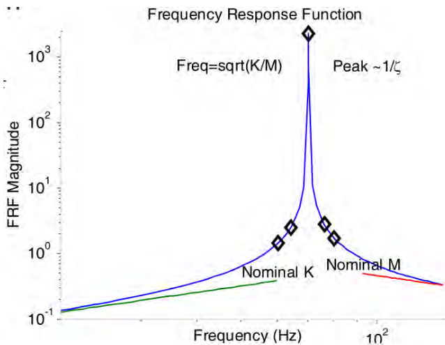
รูปที่ 16 การ Fit Curve ของ Frequency Response Function
