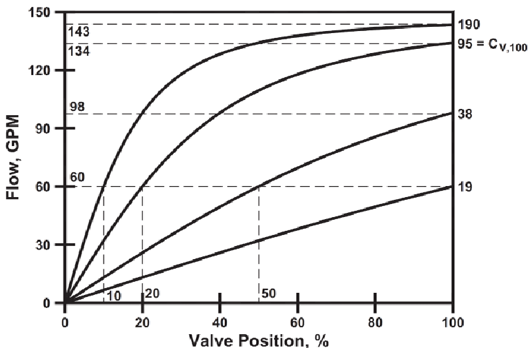
รูปที่ 4-13 ตัวอย่างผลกระทบจากการเลือกใช้วาล์วลักษณะ Linear Flow Characteristic ที่มีขนาดเกินพอดีในระบบหรือกระบวนการที่มีสัดส่วนค่าความดันตกคร่อมวาล์วมีค่าสูงมากเมื่อเทียบกับค่าความดันตกคร่อมของทั้งระบบที่ทำการติดตั้ง
