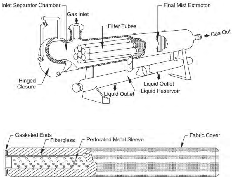
รูปที่ 30 เครื่องกำจัดไอน้ำหรืออากาศแบบ Filter Separator (ด้านบน) และตัว Filters (ด้านล่าง)
