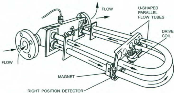
รูปที่ 4 โครงสร้างโดยทั่วไปของมาตรวัดมวลคอริโอลิส (Micro Motion, Inc.)
