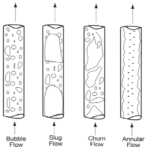
รูปที่ 3 รูปแบบการไหลแบบ 2-Phase ภายในท่อแนวตั้ง
