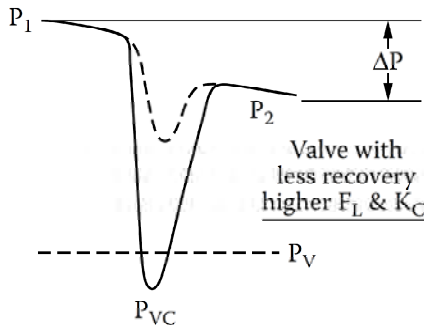
รูปที่ 4-68 เลือกวาล์วที่มีค่าความดันพื้นตัว ( F_L ) มากๆ
