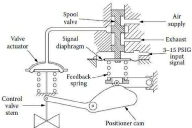
รูปที่ 6-27 หลักการทำงาน Force Balance Positioner
