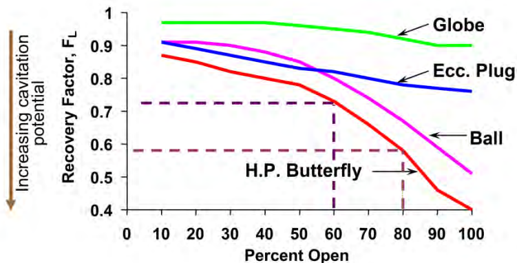
รูปที่ 4-67 Pressure Recovery Factor; F_L ของแต่ละชนิดของวาล์วโดยทั่วไป
