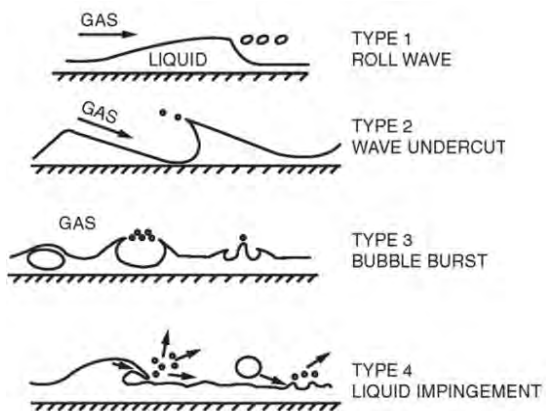
รูปที่ 22 ปรากฏการณ์การแยกตัวของเหลวกับแก๊ส
