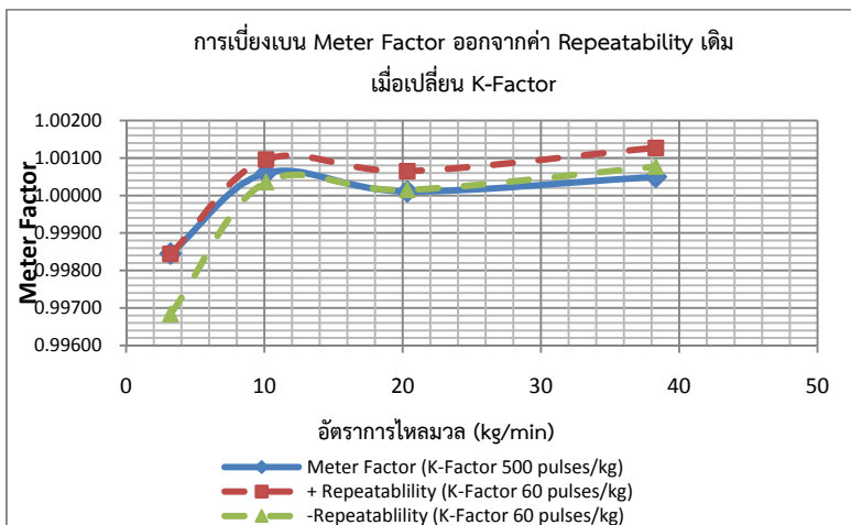
รูปที่ 33 ผลเปรียบเทียบ Meter Factor มาตราวัดมวลคอริออริส CNG050S ด้วย ค่า K-Factor 500 pulses/kg (After Adjustment)
