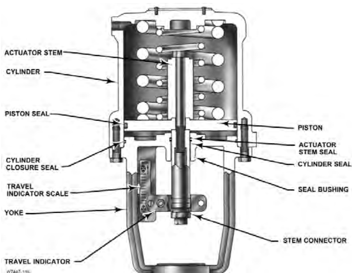
รูปที่ 6-9 รูปแบบโดยทั่วไปของ “Duplex” หรือ “Double Acting” ใน Piston-Cylinder Actuator
