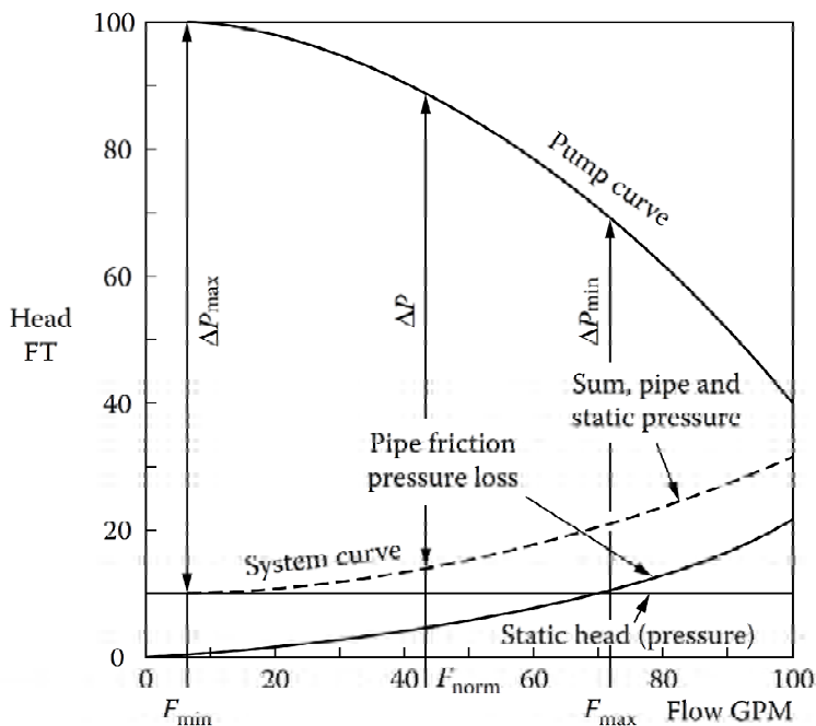
รูปที่ 4-31 ความดันตกคร่อมวาล์วมีค่าแตกต่างกันเมื่ออัตราการไหลต่างกัน
