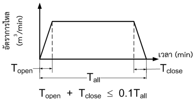
รูปที่ 8 รูปแบบอัตราการไหลเทียบกับเวลาของมาตรวัดแบบมาตรา (ทางปฏิบัติ)
