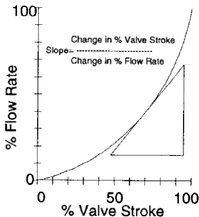
รูปที่ 4-32 Equal Percentage Valve Gain
