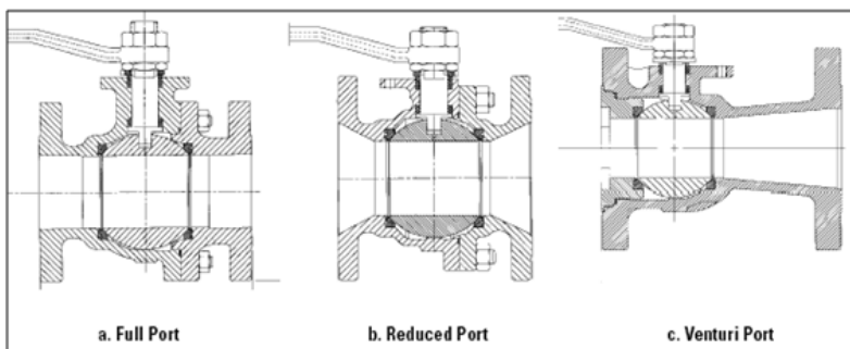
รูปที่ 3-42 ช่องทางการไหล Full Port, Reduced Port และ Venturi Port
