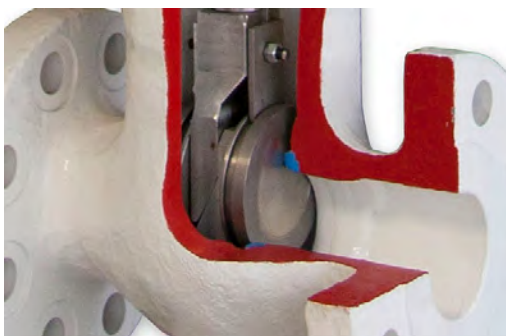
รูปที่ 3-13 ลิ้นวาล์วแบบ Double-Disc Gate Valve
