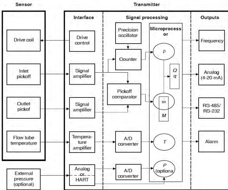
รูปที่ 19 ไตอะแกรมประมวลผลสัญญาณมาตรวัดมวลคอรีออริส
