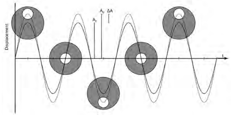
รูปที่ 16 ภาพตัดของของเหลวและฟองก๊าซภายในท่อดึง ก๊าซซึ่งมีความหนาแน่นน้อยกว่าของเหลวจึงมีความเร่งสูงกว่าจึงมีแอมพลิจูดของการสั่นสูงกว่าของเหลว
