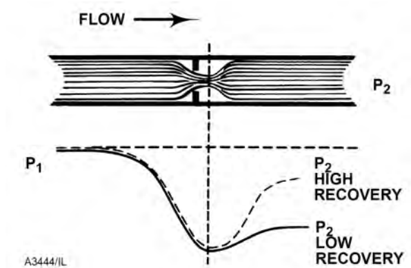
รูปที่ 4-40 การฟื้นตัวของความดันเมื่อผ่านช่องทางแคบๆ (เสมือนวาล์ว)
