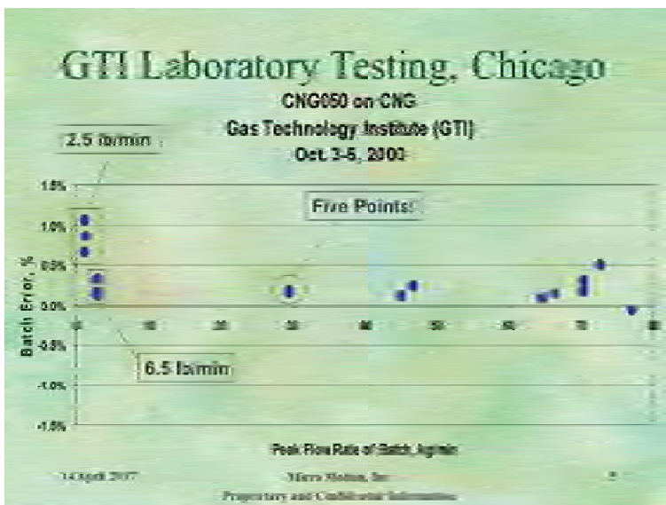
รูปที่ 42 การพิจารณา Repeatability ของมาตรวัดมวลคอริออริสเทียบกับอัตราการไหลสูงสุดของการจ่ายเป็นปริมาณจำนวนหนึ่งต่อครั้ง (Batch) มีค่าน้อยกว่า \pm 0.25\% of Rate
