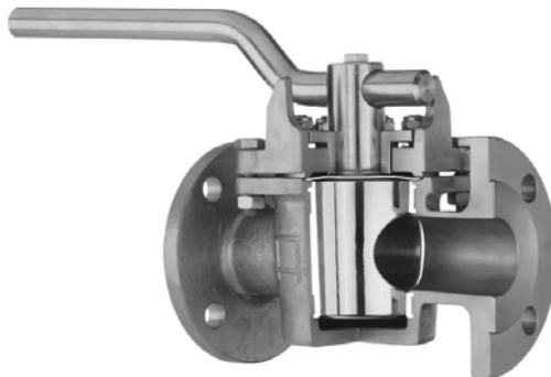
รูปที่ 3-65 Sleeved Plug Valve มีช่องทางเปิดรูปวงกลม 100%
