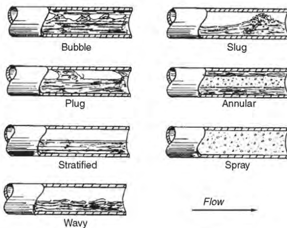
รูปที่ 1 รูปแบบการไหลแบบ 2-Phase ภายในท่อแนวระนาบ
