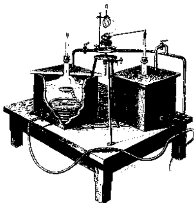
รูปที่ 25 เครื่องมืออุปกรณ์ที่ใช้ล้างตุ้มน้ำหนักแบบมาตรา Platinum-Iridium Prototypes ด้วยไอ Alcohol และไอน้ำพ่นโดยตรงไปยังตุ้มน้ำหนักแบบมาตรา ของ BIPM ในช่วงปี ค.ศ. 1882 -1889
