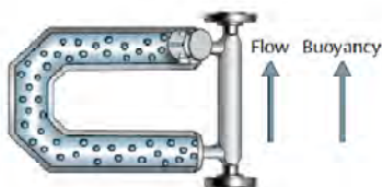
รูปที่ 21 ทิศทางการติดตั้ง มาตรวัดมวลคอโรอริสเพื่อลดการสะสมของ ฟองอากาศ
