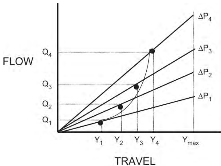
รูปที่ 4-10 ความสัมพันธ์ระหว่างอัตราการไหลผ่านวาล์วเทียบกับระยะยกตัวเคลื่อนที่ของก้านวาล์วที่มีค่าความดันตกคร่อมคงที่แต่แตกต่างกัน เมื่ออยู่ภายใต้สภาวะการทำงานจริง
