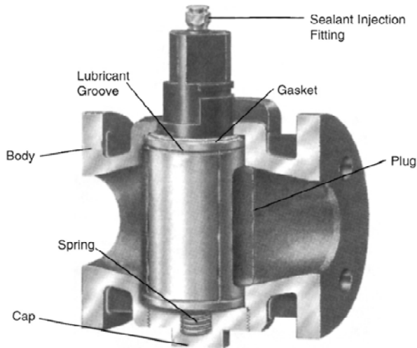
รูปที่ 3-63 Lubricate Plug Valve
