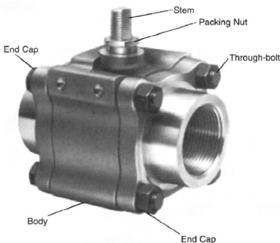
รูปที่ 3-40 ชนิด 3-Piece Design ของ Ball Valve
