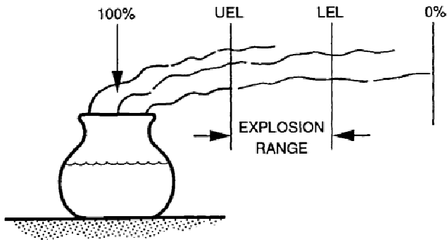
รูปที่ 2 ความเข้มข้นของไอสารไวไฟในเทอมของปริมาณเปอร์เซ็นต์ของสารไวไฟหรือส่วนที่เป็นไอระเหยผสมอยู่ในอากาศ
