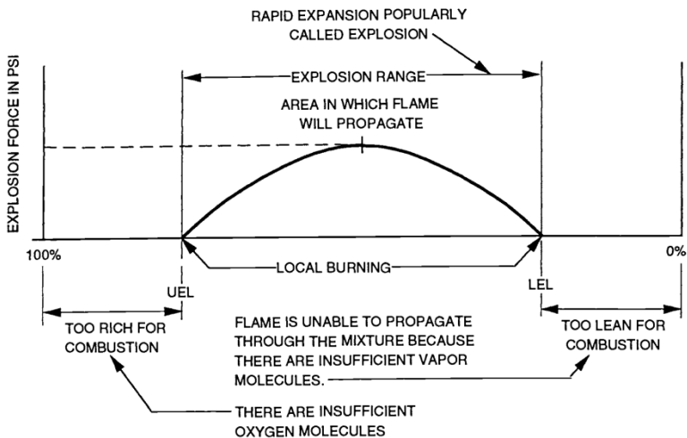
รูปที่ 3 ขอบเขตการการจุดติดไฟของสารไวไฟ
