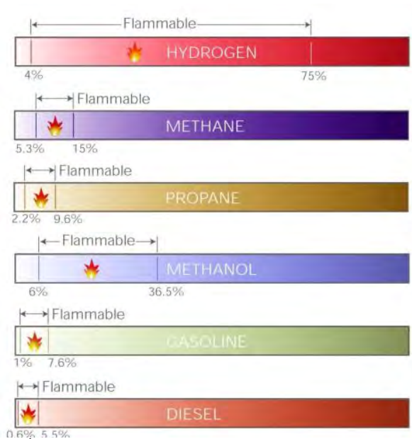
รูปที่ 3 ตัวอย่างขอบเขตการจุดติดไฟของสารไวไฟ
