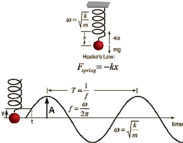
รูปที่ 2 การเคลื่อนที่ของมวลบนปลายสปริง (Harmonic Motion)
