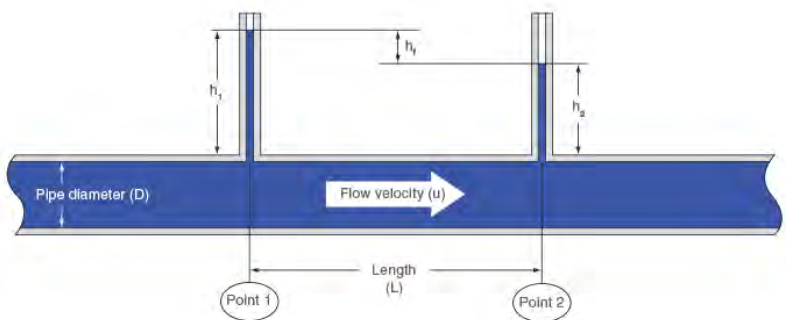
รูปที่ 4-24 ความเสียดทานสูญเสียภายในท่อ (Head Loss)
