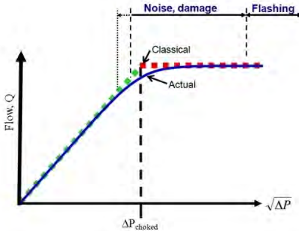
รูปที่ 4-60 ปรากฏการณ์จากสภาวะ Non-Choked Flow เป็น Choked Flow
