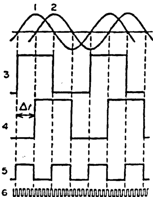
รูปที่ 20 โดอะแกรมการทำงานของส่วนอิเล็กทรอนิกส์และส่วนประมวลผล โดยกราฟหมายเลข 5 และ หมายเลข 6 (สัญญาณนาฬิกามาตรฐาน) เป็นการทำงานภายในตัว Counter 1 (รูปบน)
