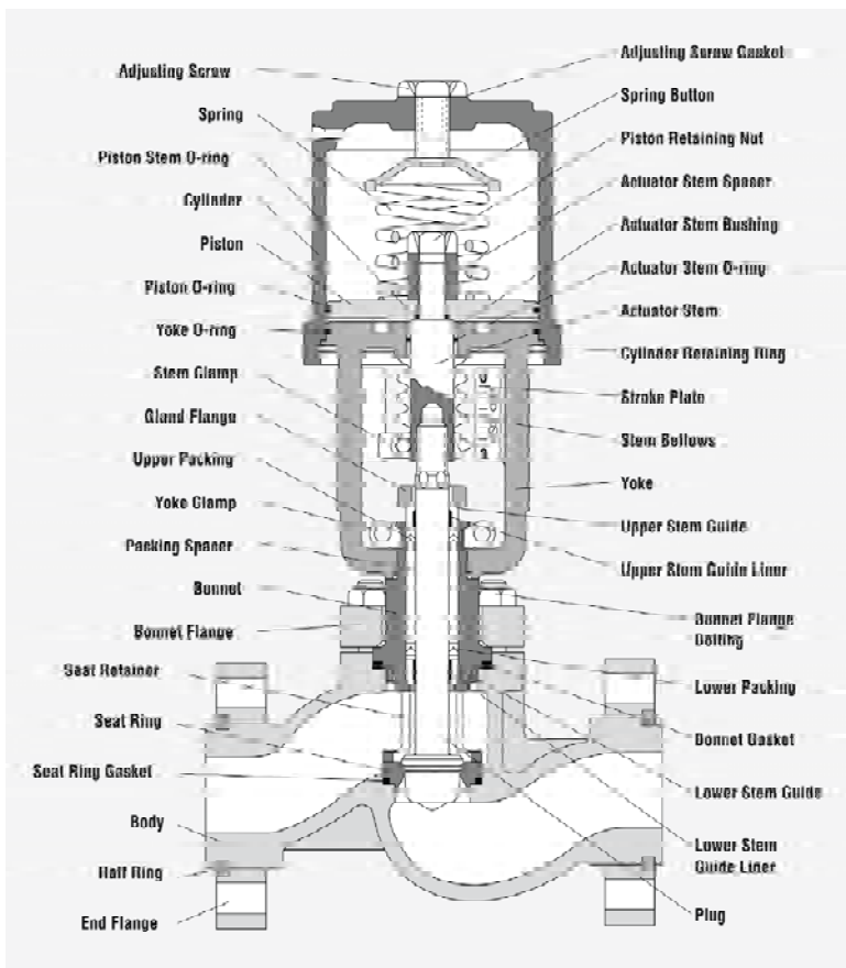
รูปที่ 2-3 ชิ้นส่วนของวาล์วควบคุม
