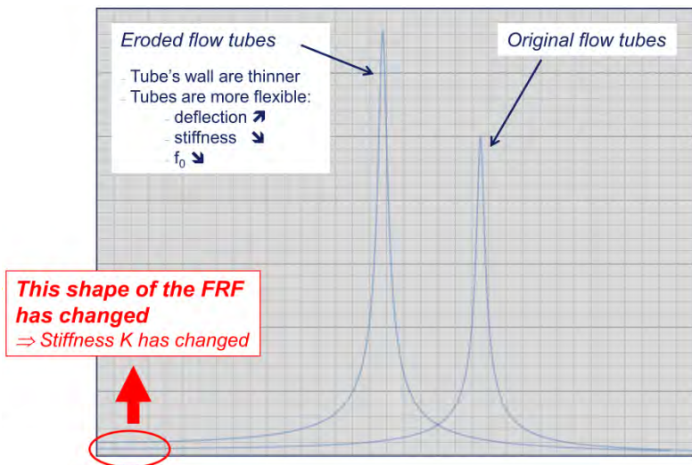
รูปที่ 13 เปรียบเทียบความถี่ธรรมชาติในการสั่นของท่อน้ำเปลี่ยนไปเมื่อทดสอบที่อัตราการไหลเดียวกัน
