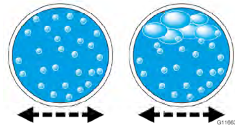
รูปที่ 11 รูปแบบอากาศที่เข้าไปหรือเกิดขึ้นในระบบท่อแบบ Gas Bubbles และ Slug Flow
