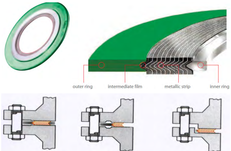
รูปที่ 3-4 Filled Spiral-Wound Gasket และตัวอย่างการติดตั้งเข้ากับหน้าแปลนในรูปแบบต่างๆ
