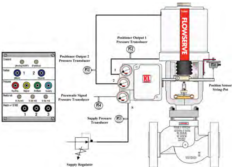
รูปที่ 6-33 Electro-Pneumatic Positioner
