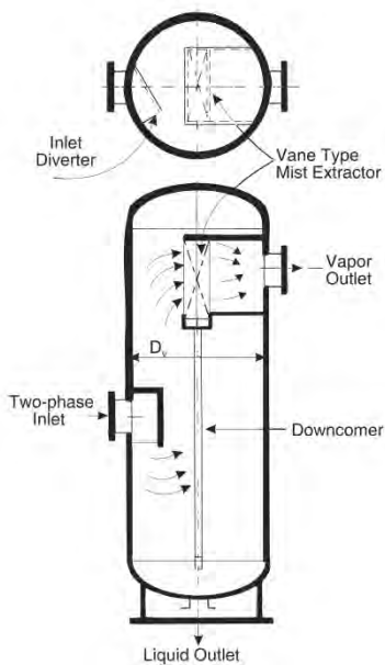
รูปที่ 15 Vane-Type พร้อมด้วย Corrugated plates และภาตรองรับภายในตัว
