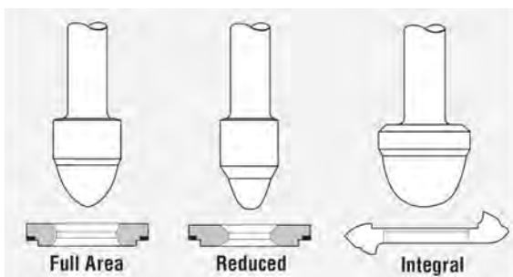
รูปที่ 4-37 ชนิดของ Seat Ring กับลิ้นวาล์วในช่องทางการไหล (Port) บางครั้งเรียกรวมกันว่า “Trim” ของ Globe Valve
