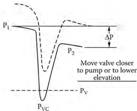
รูปที่ 4-65 ติดตั้งวาล์วในตำแหน่งต่ำกว่าระบบเพื่อเพิ่ม Static Head ทางเข้า วาล์ว
