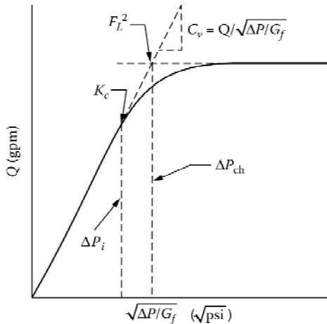
รูปที่ 4-44 นำสมการ (4-11) เขียนกราฟความสัมพันธ์อัตราการไหลกับรากที่สองของความดันตกคร่อมวาล์วเมื่อเกิด Choked Flow และ Cavitation
