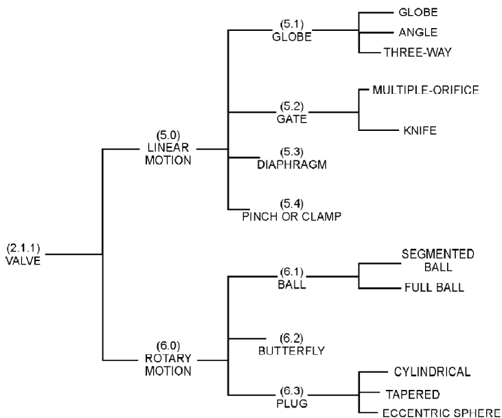
รูปที่ 1-2 การแบ่งกลุ่มวาล์วควบคุม (Control Valve) ตาม ISA-S75.05-1983
