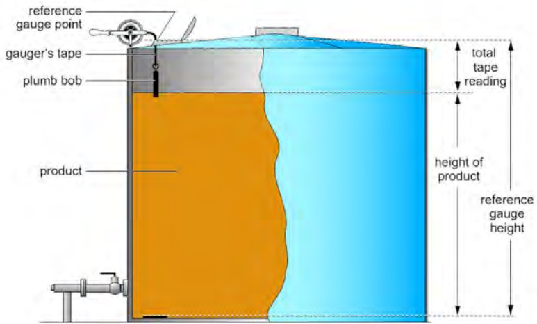
รูปที่ 14 ระยะต่างๆ ของการวัดระดับของเหลวภายในถังสำรองแบบ OUTAGE or ULLAGE Method
