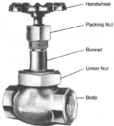
รูปที่ 3-3 Union Body-Bonnet Joint, Gate Valve
