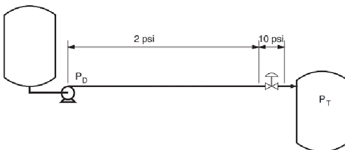
รูปที่ 4-11 ตัวอย่างระบบหรือกระบวนการที่มีสัดส่วนค่าความดันตกคร่อมวาล์วมีค่าสูงมากเมื่อเทียบกับค่าความดันตกคร่อมของทั้งระบบที่ทำการติดตั้ง
