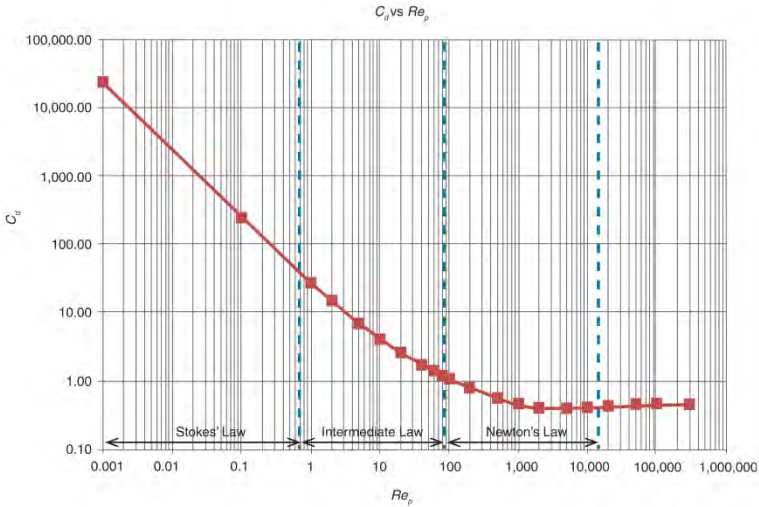
รูปที่ 34 ความสัมพันธ์ของ C_D กับ Reynold Number สำหรับวัตถุทรงกลม
