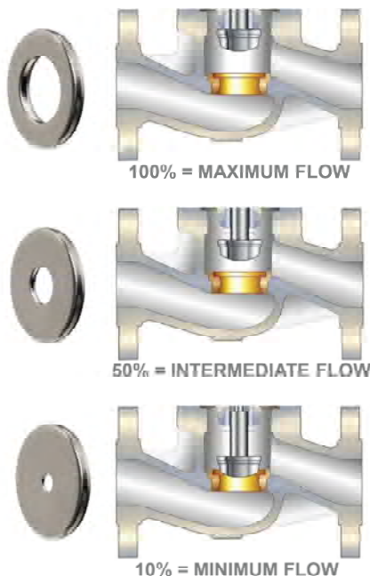
รูปที่ 3-16 พื้นที่ช่องเปิดในรูปแบบของวงกลม (Annular Space) ของ Globe Valve
