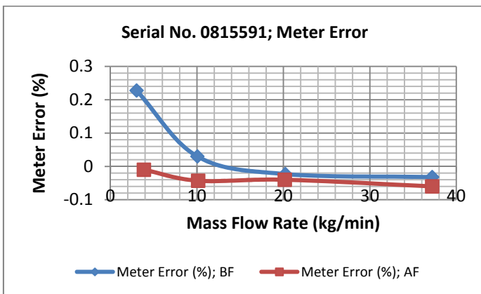
รูปที่ 38 สมรรถนะของมาตรวัดมวลคอริออริสหมายเลข 6680-014-004-51 (SN 0815591)
