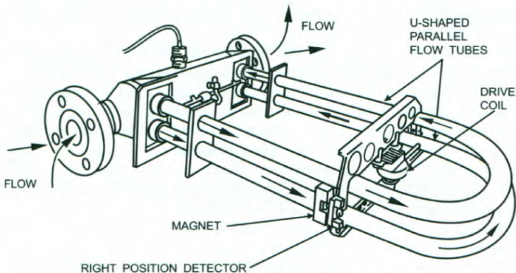
รูปที่ 1 โครงสร้างโดยทั่วไปของมาตรวัดมวลคอริออริส (Micro Motion, Inc.)
