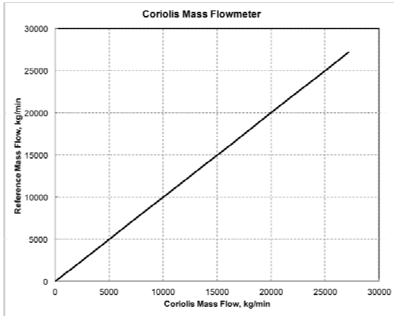
รูปที่ 11 กราฟความสัมพันธ์อัตราการไหลมวลที่วัดได้จากมาตรวัดมวลคอริสอริสเทียบกับอัตราไหลมวลของแบบมาตรา ตามสมการ (18)
