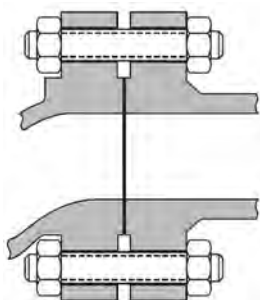
ข. หน้าแปลนชนิดหน้ายก
