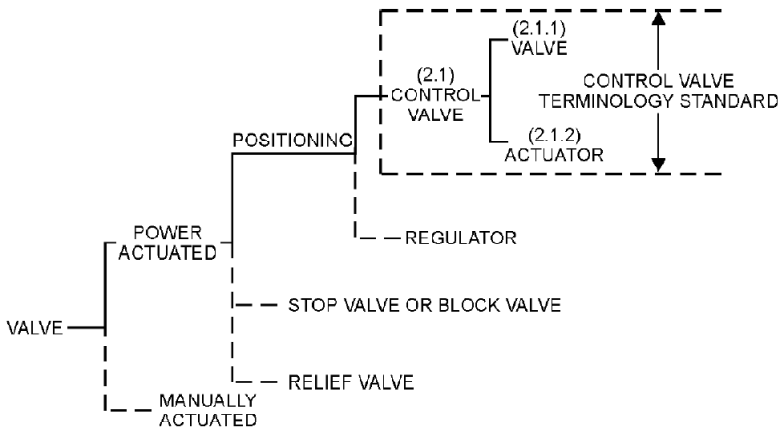
รูปที่ 1-1 การแบ่งกลุ่มวาล์ว ตาม ISA-S75.05-1983
