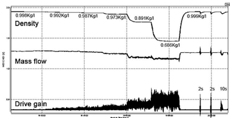
รูปที่ 18 ความสัมพันธ์ระหว่าง Drive Gain อัตราการไหลมวล (Mass Flow) และค่าความหนาแน่นของเหลวที่วัดได้ของมาตรวัดมวลคอโรอริส
