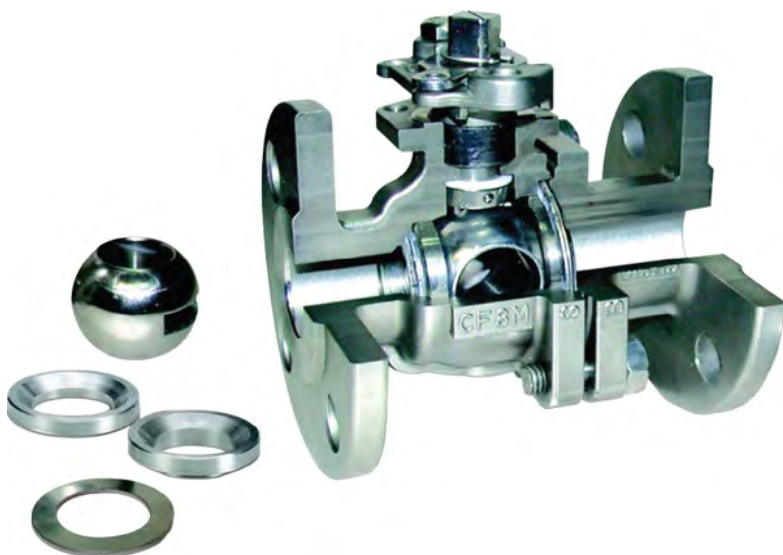
รูปที่ 3-50 Metal Seat ใน Ball Valve
