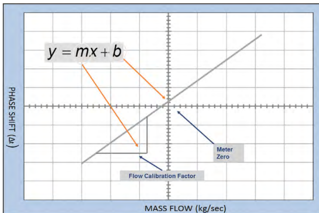
รูปที่ 12 กราฟแสดง Meter Zero เมื่อค่าความชันกราฟ m = F.C.F และค่าตัดแกน Y หรือ b = \text{Zero Offset}
