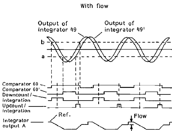
รูปที่ 21-2 Micro Motion Signal Processing System (บน) ณ สภาวะไม่มีการไหล, (ล่าง) ณ สภาวะที่มีการไหลผ่านท่อวัด
