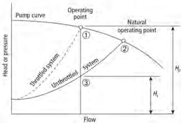
รูปที่ 4-28 การหรีวาล์วจะสร้างเส้นกราฟความดันสูญเสียของระบบใหม่เมื่อหรีวาล์ว (Throttled System)
