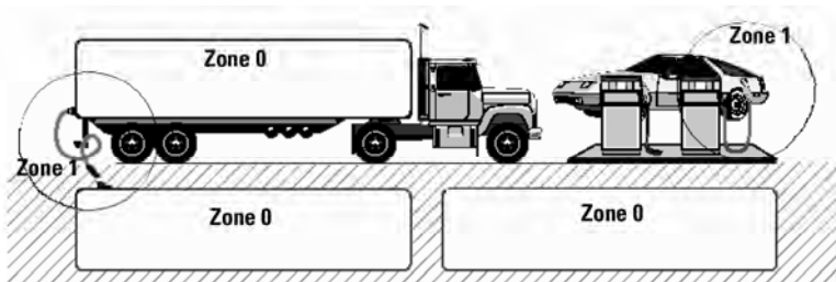
รูปที่ 3 แนวความคิดการแบ่งโซน ตาม IEC
