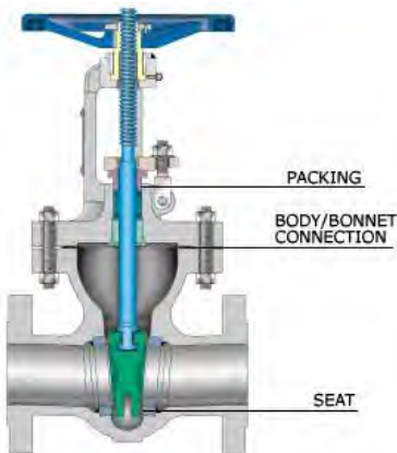
รูปที่ 1-6 On/Off หรือ Block Valve
