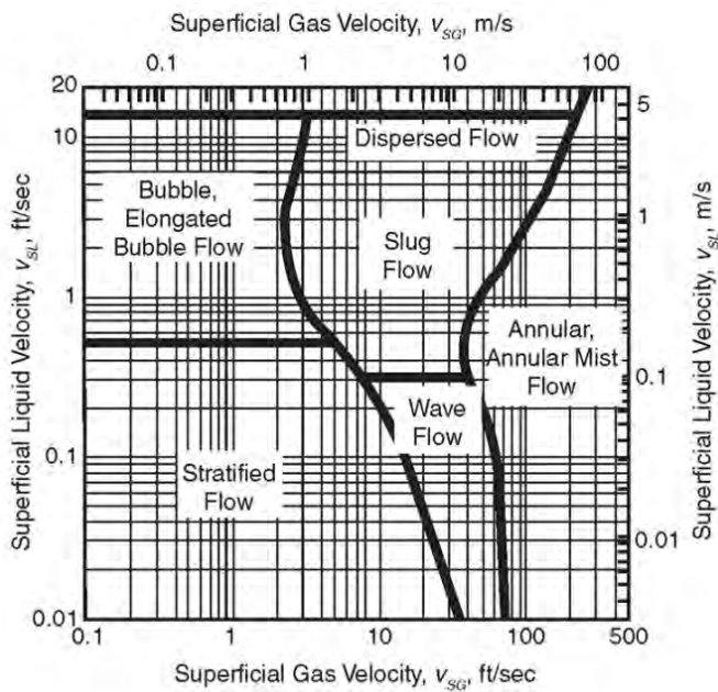
รูปที่ 2 Horizontal Flow Pattern Map (Mandhane 1974)
