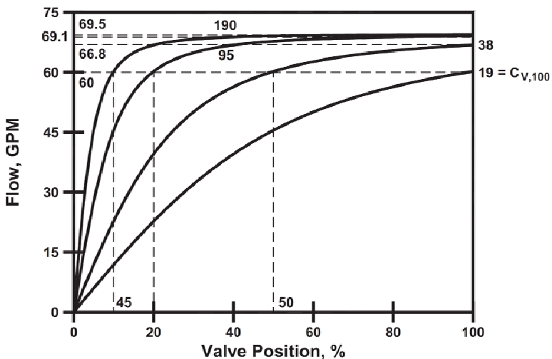
รูปที่ 4-18 ตัวอย่างผลกระทบจากการเลือกใช้วาล์วลักษณะ Linear Flow Characteristic ที่มีขนาดเกินพอดีในระบบหรือกระบวนการที่มีสัดส่วนค่าความดันตกคร่อมของทั้งระบบที่ติดตั้งวาล์วมีค่าสูงมากเมื่อเทียบกับค่าความดันตกคร่อมวาล์ว
