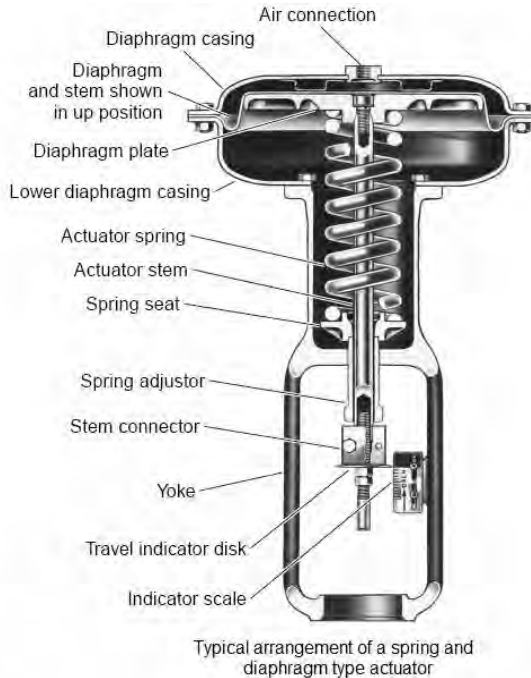
รูปที่ 6-3 โครงสร้างโดยทั่วไปของ Actuator ซึ่งติดตั้งเข้ากับ Globe Valve
