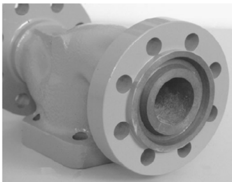
รูปที่ 2-11 ข้อต่อหน้าแปลนหน้าสัมผัสชนิด Ring-type Joint (RTJ)
