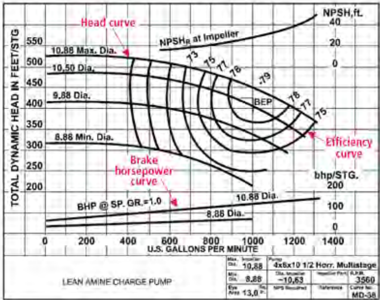
รูปที่ 4-22 ตัวอย่างกราฟแสดงสมรรถนะของปั๊ม (Pump Performance)
