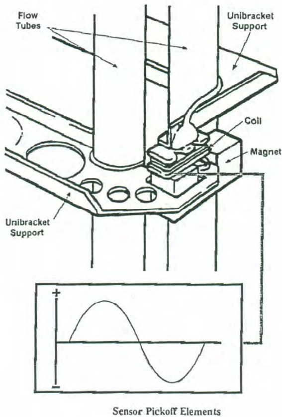
รูปที่ 8 การเหนี่ยวนำไฟฟ้ากระแสสลับขึ้นภายใน Coil เขียนกราฟความสัมพันธ์ระหว่างความต่างศักย์ไฟฟ้าที่เหนี่ยวนำขึ้นภายใน Coil เทียบกับคาบเวลา
