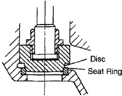
รูปที่ 3-24 ลิ้นวาล์วแบบ Spherical Seat
