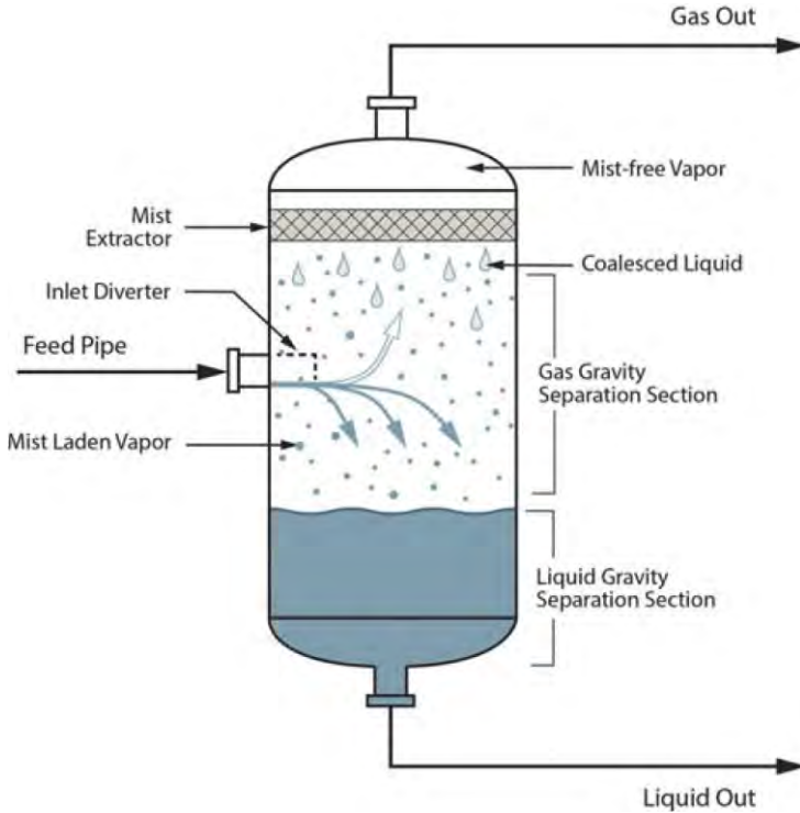
รูปที่ 33 หยดของเหลว (Droplets) ที่ผสมอยู่ในของไหล 2 สถานะ ในส่วนที่เป็นก๊าซภายในเครื่องกำจัดไอหรืออากาศ
