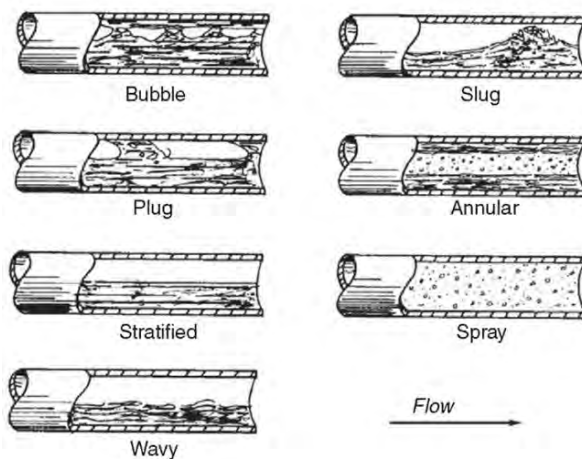
รูปที่ 2 รูปแบบการไหลแบบ 2-Phase ภายในท่อแนวระนาบ
