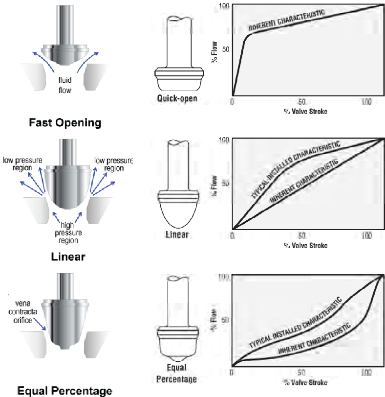
รูปที่ 4-36 ชนิดของลิ้นวาล์วของ Globe Valve กับ Flow Characteristic
