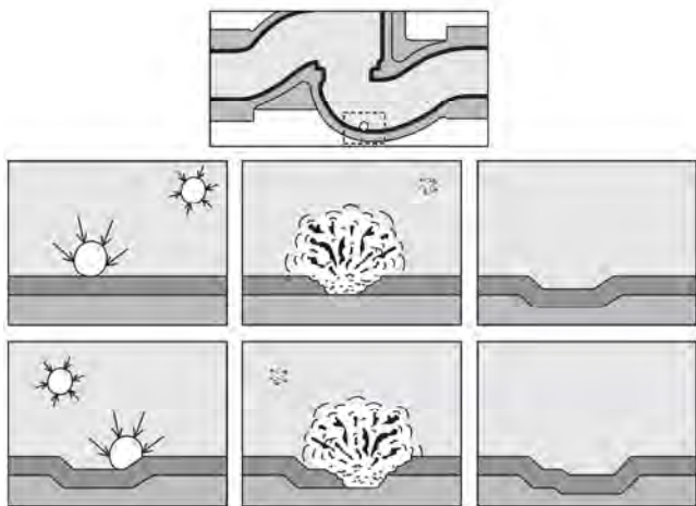
รูปที่ 4-45 ตัวอย่างการเกิด Cavitation ภายในตัวเรือนวาล์ว
