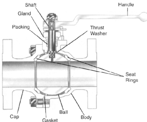
รูปที่ 3-35 ส่วนประกอบหลักๆ ของ Ball Valve
