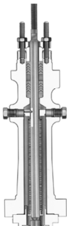
ข. Bellows Seal Bonnet รูปที่ 2-4 ตัวอย่างการออกแบบ Bonnet
