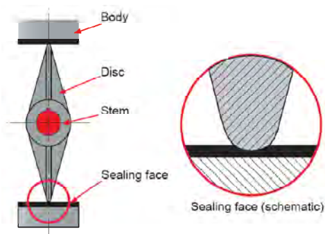
รูปที่ 3-53 Sealing structure of centered seal butterfly valve
