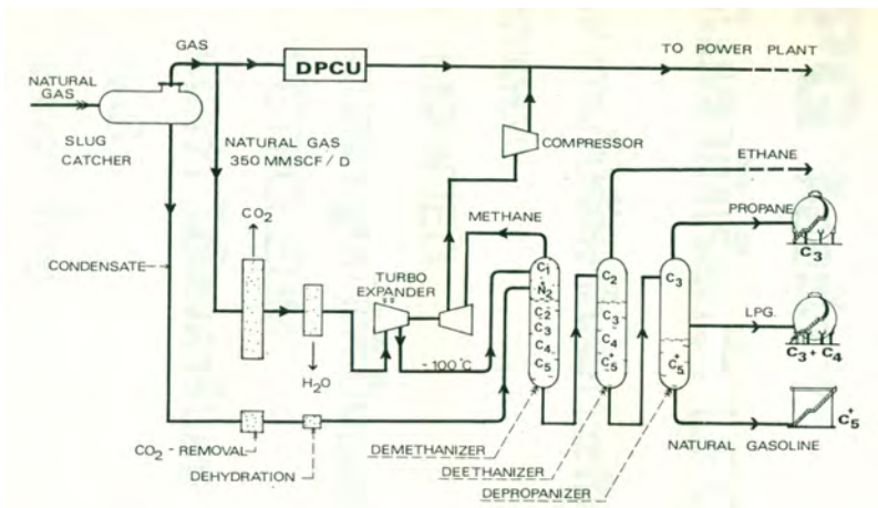
รูปที่ 1 ขั้นตอนการแยกก๊าซธรรมชาติ เพื่อให้ได้ก๊าซ LPG
