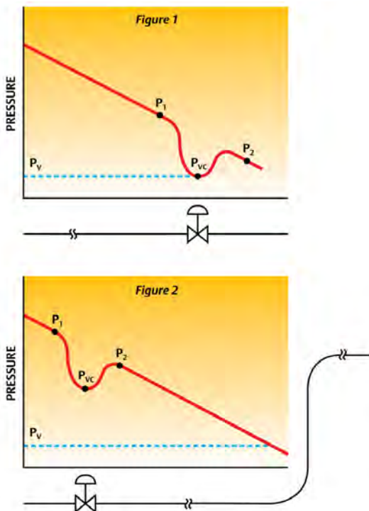
รูปที่ 4-63 เปลี่ยนตำแหน่งติดตั้งวาล์วให้อยู่ต้นน้ำเพื่อเพิ่มความดันทางเข้าวาล์ว
