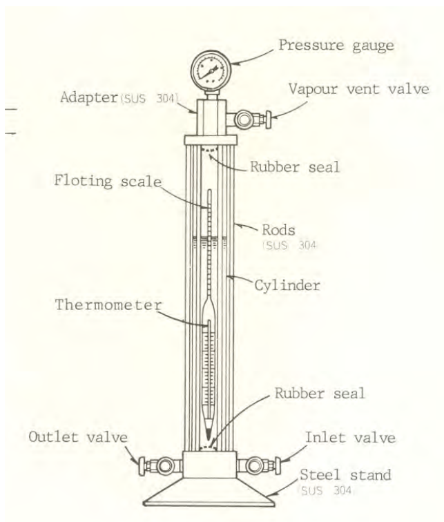
รูปที่ 1 เครื่องวัดความถ่วงจำเพาะ LPG ประกอบด้วย Hydrometer พร้อมเครื่องวัดอุณหภูมิและเกจวัดความดัน
