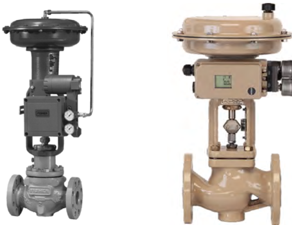
รูปที่ 6-38 Electro-Pneumatic Positioner ใช้ I/P Converter
