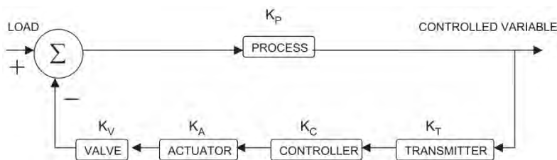
รูปที่ 4-34 การทำงานร่วมของส่วนทำงานของระบบ Control Loop
