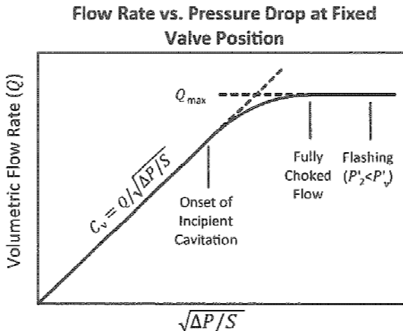
รูปที่ 4-54 พัฒนาการของการเกิด Cavitation
