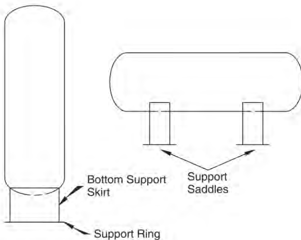
รูปที่ 24 เปรียบเทียบโครงสร้างรองรับสำหรับเครื่องกำจัดไอน้ำหรืออากาศแบบแนวตั้งและแบบแนวนอน
