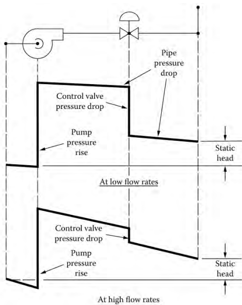
รูปที่ 4-29 ความดันของปั๊มและความดันตกคร่อมวาล์วมีค่าแตกต่างกันเมื่ออัตราการไหลต่างกัน
