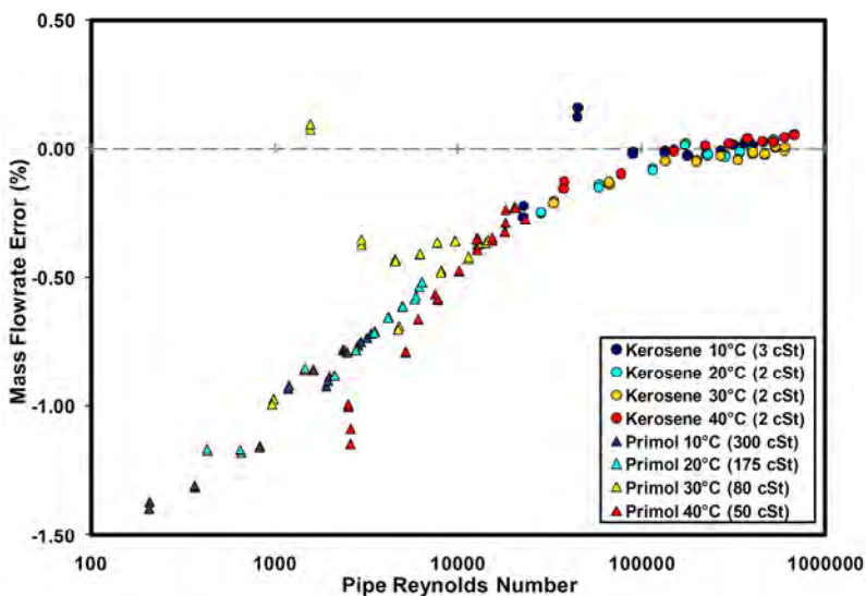
รูปที่ 50 Reynolds Number มีผลต่อผลผิดอัตราการไหลมวลของมาตรวัดมวลคอรีออริสเมื่อใช้กับของเหลวที่มีค่าความหนืดต่างกัน
