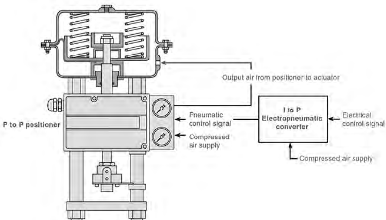
รูปที่ 6-37 สัญญาณไฟฟ้าจากตัวควบคุมถูกแปรความหมายด้วย I/P Converter แล้วส่งสัญญาณความดันอากาศไปยัง Positioner ซึ่งขยายสัญญาณความดันอากาศแล้วส่งแรงดันอากาศไปขับเคลื่อน Actuator
