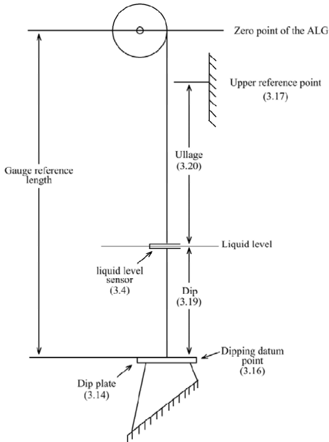
รูปที่ 9 ระยะและตำแหน่งการวัดระดับของเหลวภายในถังฯ (OIML R85-1,2008)
