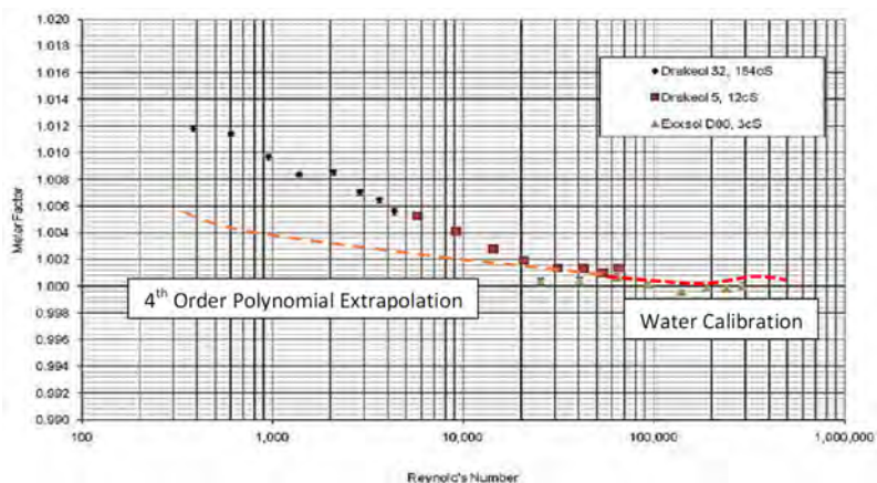
รูปที่ 49 ค่า Meter Factor ของการสอบเทียบ Ø 4" Coriolis Meter
