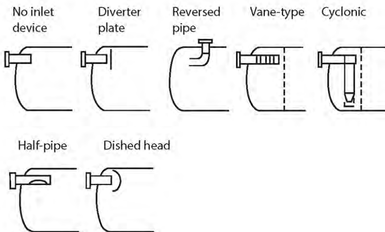
รูปที่ 8 ชนิดของ Inlet Device ของเครื่องกำจัดไอหรืออากาศ
