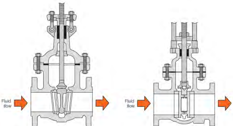
รูปที่ 3-15 เปรียบเทียบวาล์วที่มีลิ้นวาล์วแบบ Wedge กับแบบ Parallel
