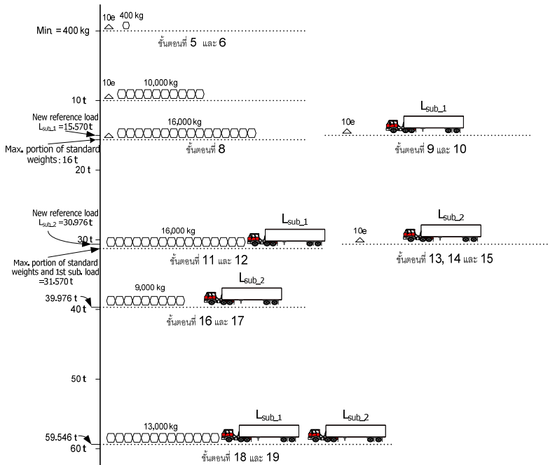
ภาพแสดงตัวอย่าง การซึ่งน้ำหนักอื่นแทนค่าน้ำหนักของสินค้าหนักแบบมาตรฐาน
