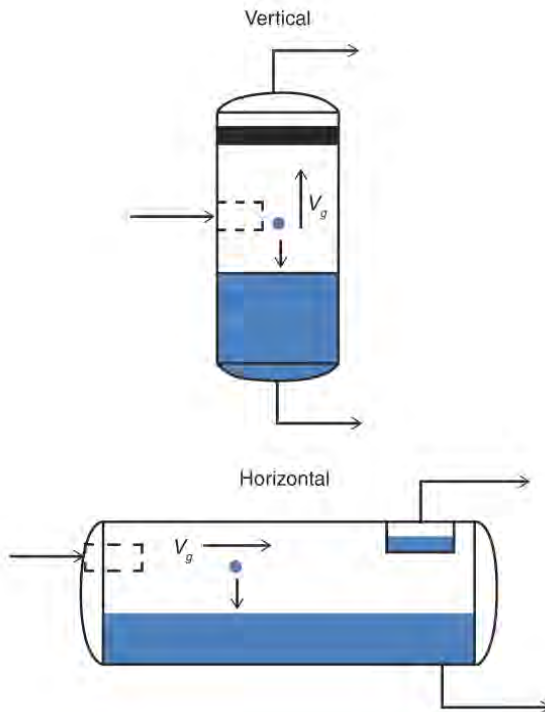
รูปที่ 21 ทิศทางการไหลของก๊าซออกจากเครื่องกำเนิดไอหรืออากาศและ ทิศทางการหยดของเหลวซึ่งแยกตัวออกจากก๊าซ
