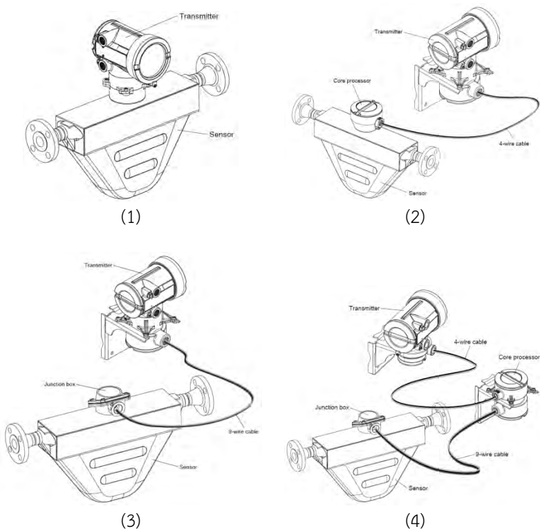
รูปที่ 23 รูปแบบการติดตั้งของมาตรวัดมวลคอโรอริส (1) Integral installation (2) 4-wire remote installation (3) 9-wire remote installation type (4) Remote core processor with remote sensor installation type (Micro Motion)
