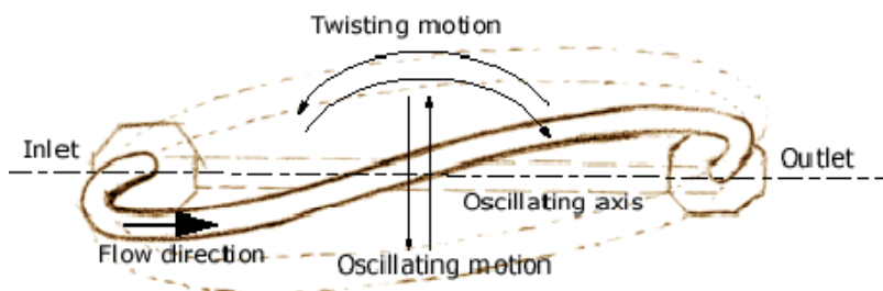
รูปที่ 8 การหมุนเชิงมุมและการบิดตัวของท่อวัดใน “Superimposed Mode” หรือ “Coriolis Mode”
