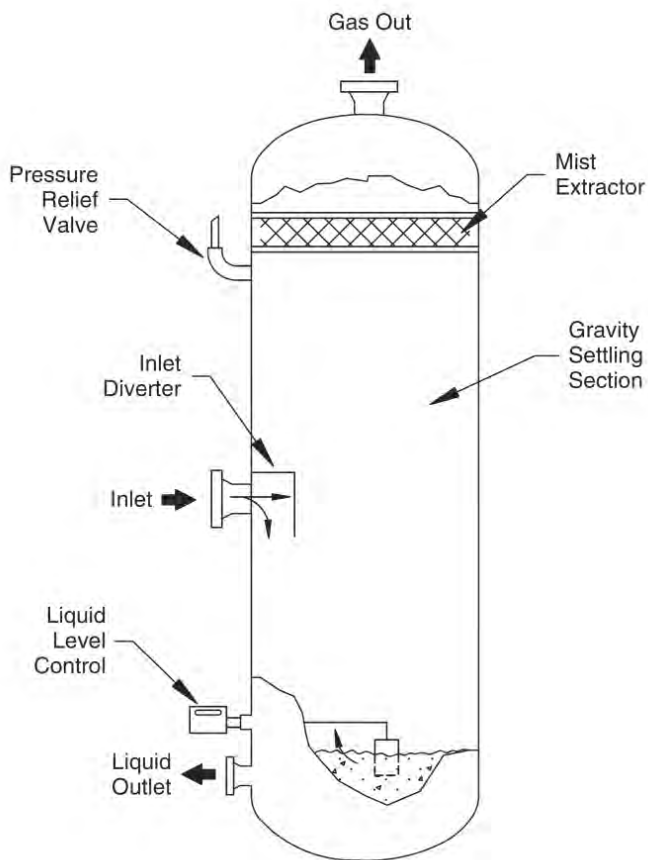
รูปที่ 23 เครื่องกำจัดไอน้ำหรืออากาศแบบแนวตั้ง
