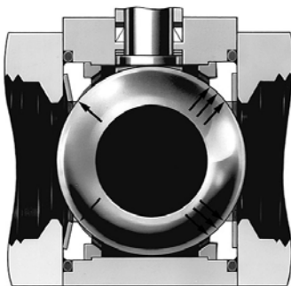
รูปที่ 3-46 แรงกระทำต่อลิ้นวาล์วลูกบอลที่ติดตั้งในรูปแบบ Floating-Ball Design ใน One-Piece Reduced Port (ของไหลความดันสูงอยู่ทางซ้ายมือ)
