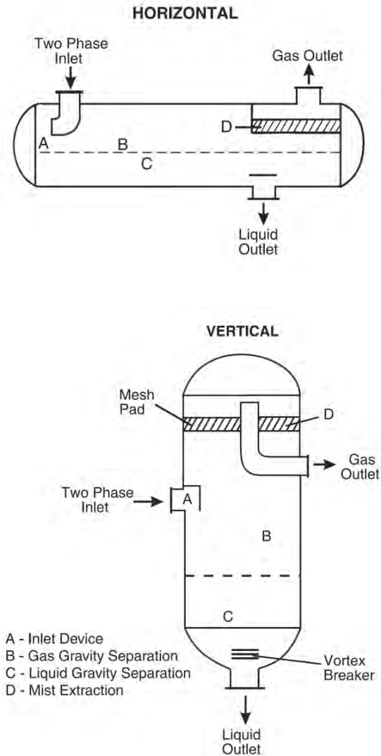
รูปที่ 7 ชนิดของ Gas - Liquid Separators
