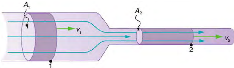
รูปที่ 4 สมการความต่อเนื่อง
