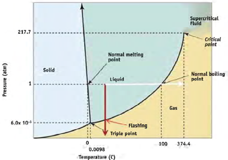
รูปที่ 4-48 Phase diagram แสดงการเปลี่ยนสถานะของเหลวกลายเป็นไอน้ำด้วยวิธีการ Boiling (อุณหภูมิเปลี่ยน ความดันคงที่) และ Flashing (อุณหภูมิคงที่ ความดันเปลี่ยน); (Machado, 2009)
