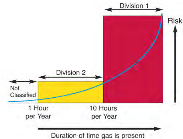
รูปที่ 2 การจำแนกพื้นที่อันตรายตามมาตรฐาน NEC เป็น Class และ Division ในเทอมของระยะเวลาของการปรากฏของสารไวไฟใน 1 ปี
