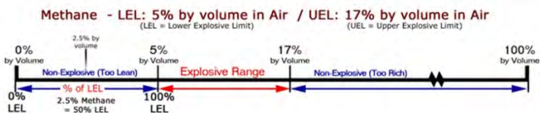
รูปที่ 4 ตัวอย่างขอบเขตการการจุดติดไฟของก๊าซ Methane
