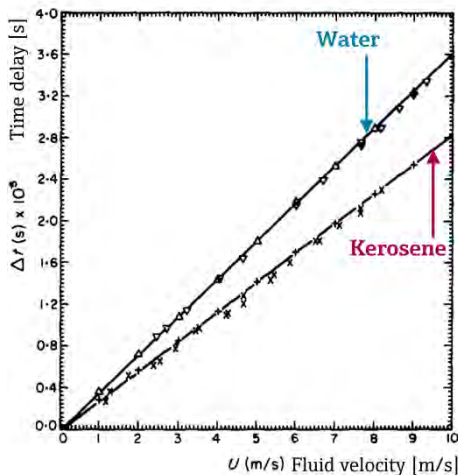
รูปที่ 10 ความสัมพันธ์ระหว่างความเร็วของไหลภายในท่อกับผลต่างการ Shift ของกราฟการเคลื่อนที่ของท่อวัดสันคิดเป็นเวลา \Delta T ขณะมีของเหลวไหลผ่านท่อ (FLOW) ต่างชนิด (ความหนาแน่นต่างกัน)
