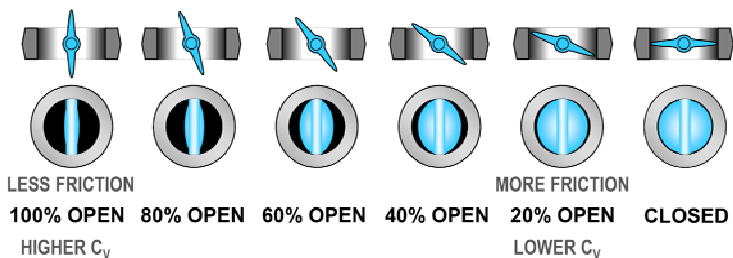
รูปที่ 3-52 รูปแบบการปิด-เปิดของล้นวาล์วชนิด Butterfly Valve
