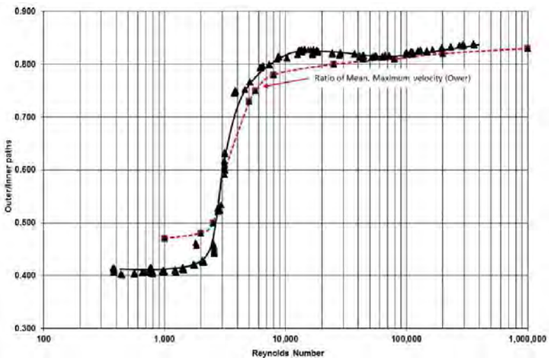
รูปที่ 10 การเปลี่ยนแปลงในอัตราส่วน Flow Profile Velocity (บริเวณใกล้ผิวท่อเทียบกับใจกลางท่อ) เมื่อเทียบกับ Reynolds Number
