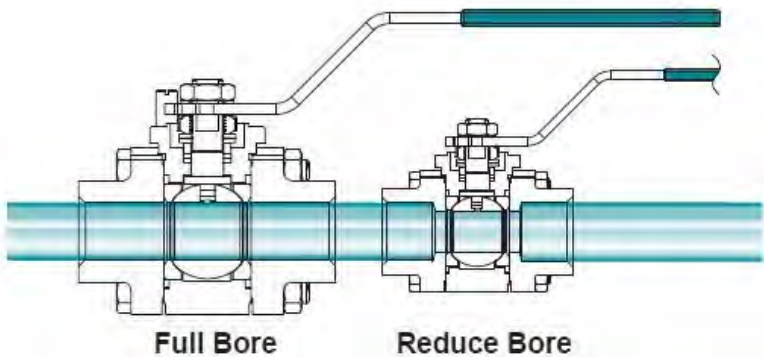
รูปที่ 3-41 เปรียบเทียบขนาดช่องทางการไหล Full Port กับ Reduced Port
