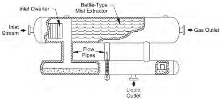
รูปที่ 28 เครื่องกำจัดไอหรืออากาศแบบ Double-Barrel Horizontal Separators ประกอบด้วย baffle-Type mist extractor
