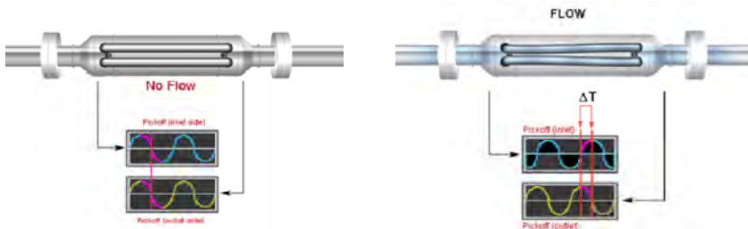
รูปที่ 9 ผลต่าง Phase Shift ของท่อวัดสันคิดเป็นเวลา \Delta T ขณะมีของเหลวไหลผ่านท่อ (FLOW: ขวามือ) กับไม่มีของเหลวไหลผ่านท่อ (NO FLOW: ซ้ายมือ) เป็นสัดส่วนโดยตรงกับอัตราการไหลมวลของเหลว
