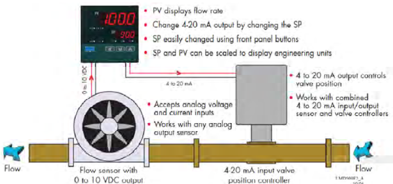
รูปที่ 1-10 ตัวอย่าง Flow Control ควบคุมด้วย Digital Controller
