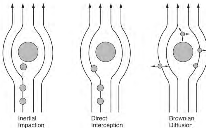
รูปที่ 12 3 กลไกหลักการทำงาน “Impingement” ในการดักจับหยดของเหลวผสมในก๊าซ
