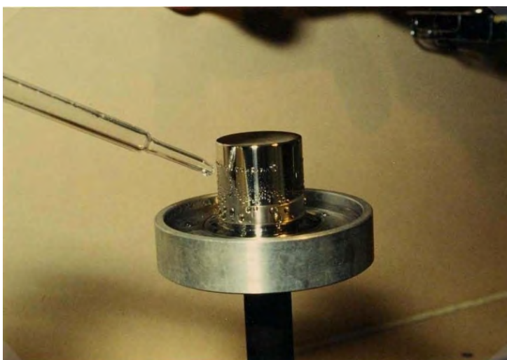
รูปที่ 32 ปลอ่ยไอน้ำพ่นให้ทั่วบริเวณส่วนผิวทรงกระบอกของ Prototype พร้อมหมุนฐานให้ Prototype เคลื่อนที่ขึ้นลง เมื่อครบ 15 -20 นาที ให้ใช้ขอบกระดาษซับตะเหยदनน้ำที่จับตัวบริเวณผิวให้หยदनน้ำถูกดึงออกจากผิวด้วย Capillary Action เท่านั้น
