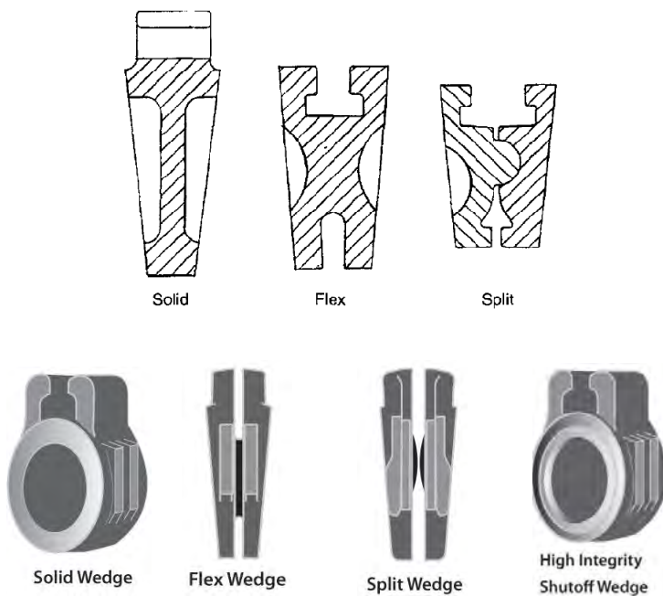
รูปที่ 3-11 ลิ้นวาล์วแบบ Solid Wedge, Flex Wedge, Split Wedge และ High Integrity Shutoff Wedge
