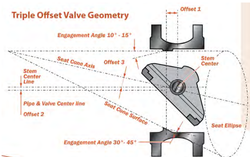
รูปที่ 3-58 การเอียงศูนย์ของลิ้นวาล์ว 3 ระยะเอียง (Triple Eccentric Bearing of the Butterfly Disc)
