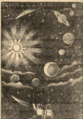
ดวงอาทิตย์และดาวฤกษ์
