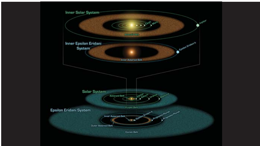
รูปที่ 2 แผนภาพแสดงแหล่งที่มาของดาวหางทั้ง 2 แหล่ง ได้แก่ แถบไคเปอร์และเมฆออร์ต (ภาพโดย www.cfa.harvard.edu )
