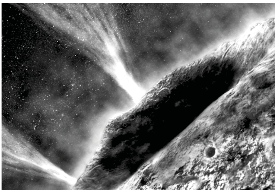
รูปที่ 12 ดาวหางโบห์แอ้เคลื่อนที่ปะทะกับบรรยากาศ ที่บีก้าชี่พวยพุ่งจากดาวหาง หรือโบห์แอ้เพียงแต่ไฮโดรคาร์บอนที่เกินคาด แต่พวกมันยังมีโมเลกุลของน้ำด้วย (ภาพโดย NASA/JPL-Caltech)
