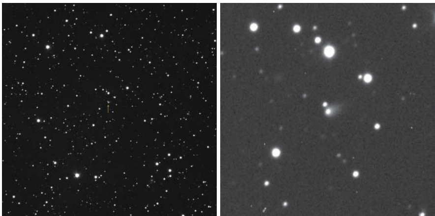
รูปที่ 9 ดาวหางไอซอน (ison C/2012 S1) ใช้วิธีเปรียบเทียบความสว่างกับดาวใกล้เคียงโดยภาพด้านซ้าย คือ ภาพดาวหางปกติ ส่วนภาพขวา คือ ทำการปรับไฟฟ้ให้ดาวใกล้เคียงมีขนาดใกล้เคียงกับดาวหางแล้วทำการวัดความสว่างก่อนนำมาเปรียบเทียบกับ ดาวหาง (ภาพโดย http://ssonblog.sierrastars.com/?cat=1 )
