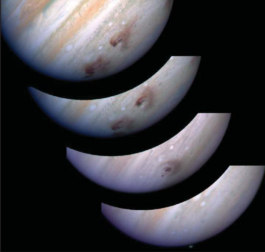
รูปที่ 28 ร่องรอยที่เกิดจากการพุ่งชนของดาวหางชูเมกเกอร์-เลวี-9 ปรากฏเป็นรอยสีดำนบนผิวดาวพฤหัสบดี ซึ่งรอยดังกล่าว มีเส้นผ่านศูนย์กลาง ใกล้เคียงกับเส้นผ่านศูนย์กลางของโลก (ภาพโดย http://commons.wikimedia.org/ )
