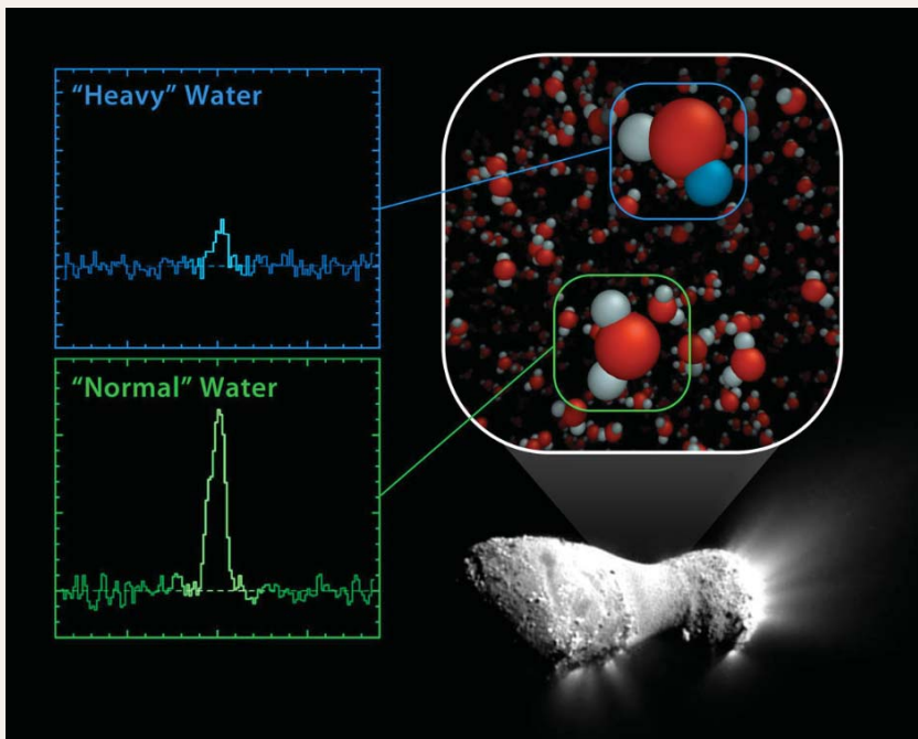
รูปที่ 13 ภาพจากการกิจ EPOXI แสดงถึงนิวเคลียสของดาวหาง ฮาร์ดลีย์-2 แสดงถึงสเปกตรัมของน้ำปกติ และน้ำแบบหนัก ซึ่งถูกวัดด้วยเครื่องมือ Heterodyne Instrument ที่ติดตั้งอยู่บนกล้องอวกาศ เฮอร์เชล (Herschel Space Observatory)
