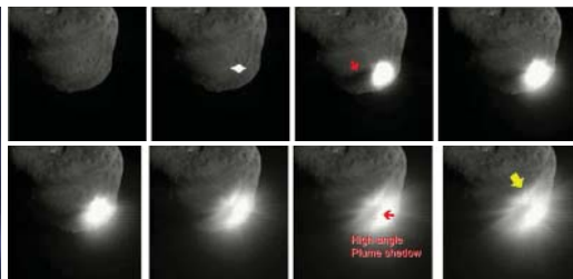
รูปที่ 21 (ซ้าย) ภาพจำลองการกีดฟอิมแพ็ค (ขวา) ภาพลำดับเหตุการณ์หลังจากยานกระแทกกับผิวของดาวหาง (ภาพโดย www.discovery.nasa.gov/SmallWorlds )
