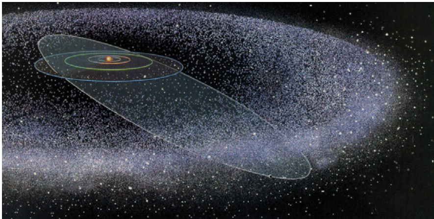
รูปที่ 25 เปรียบเทียบวงโคจรของดาวเคราะห์ กับตำแหน่งของแถบไคเปอร์และกลุ่มเมฆออร์ต ซึ่งมีขนาดแตกต่างกันอย่างมาก ( www.abysss.uoregon.edu )
