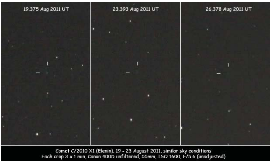
รูปที่ 15 ดาวหางเอูลิน (C/2010 X1 Elenin) เคลื่อนที่เปลี่ยนตำแหน่งเพื่อเทียบกับดาวฤกษ์เป็นหลัง
