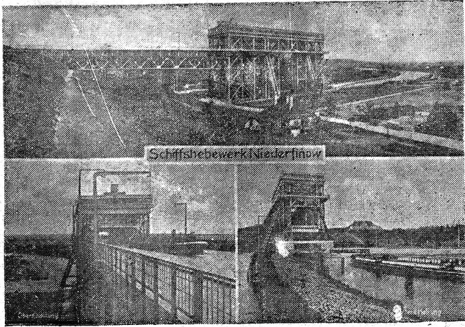
อีกภาพหนึ่งแสดงให้เห็นคานยกเรือขึ้นที่หน้าเวลา และทันสมัยที่สุดของเยอรมัน ในภาพนี้จะเห็นเรือกำลังถูกยกขึ้น และวิ่งเข้าสู่รางน้ำต่อไป และมองเห็นภาพแม่น้ำเบื้องล่าง
