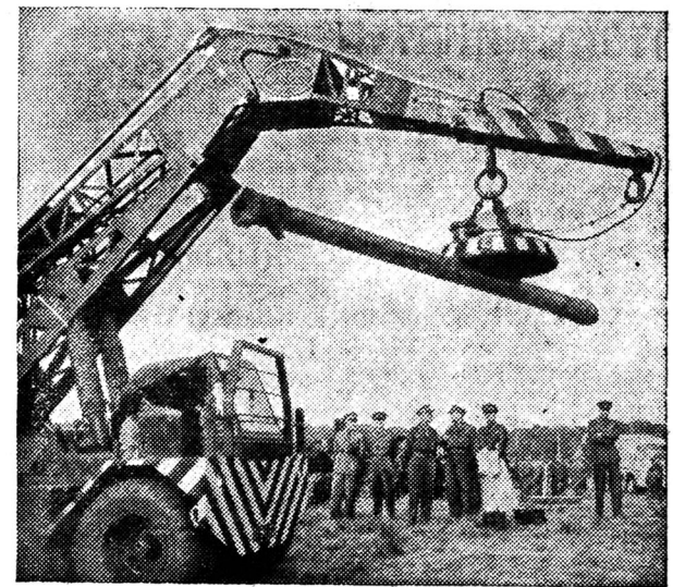
เครื่องกว้านแบบใหม่ ใช้ยกของหนักได้หลายตัน
