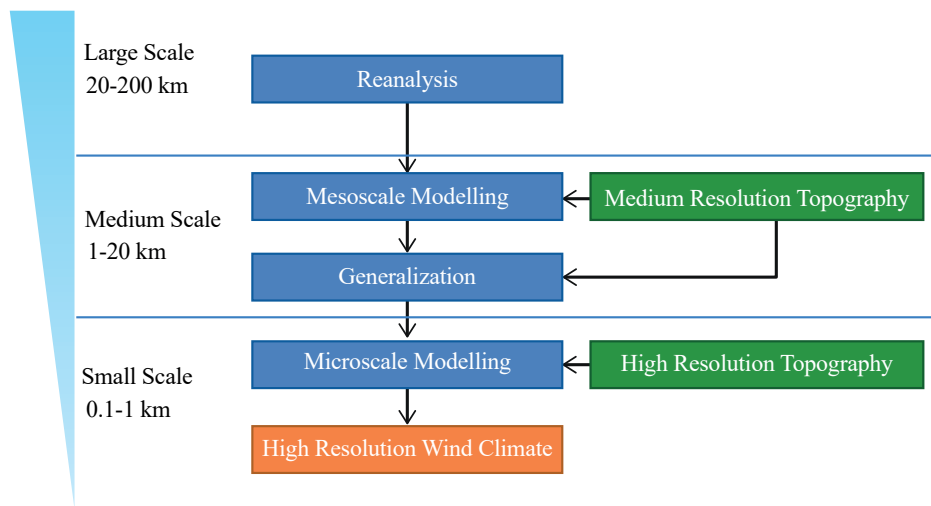
ภาพที่ 3 ระเบียบวิธีแผนที่ลมระดับมหภาค (GWA)
