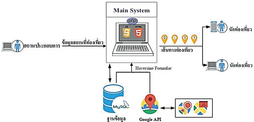
ภาพที่ 1 สถาปัตยกรรมของระบบ
