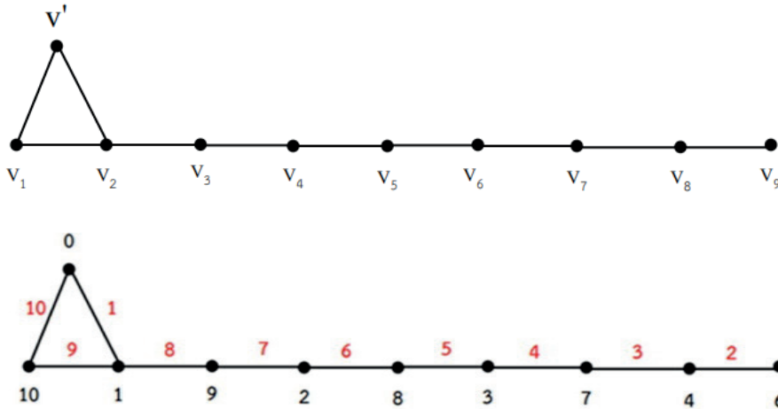
ภาพที่ 2 กราฟกราฟซึ่งเป็นกราฟที่ได้จากการทำซ้ำเส้นเชื่อมด้วยจุดยอดใหม่
