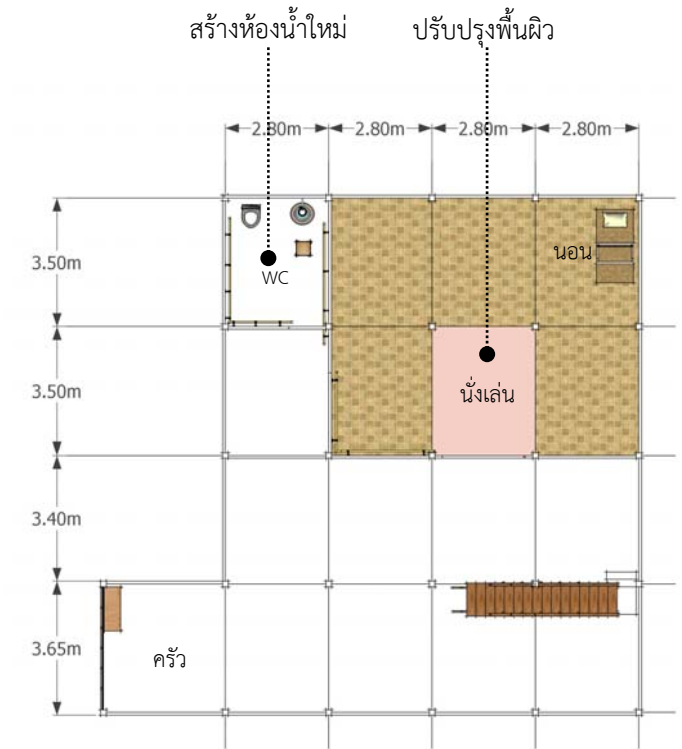
ผังพื้นที่ 1 หลังการปรับปรุง
