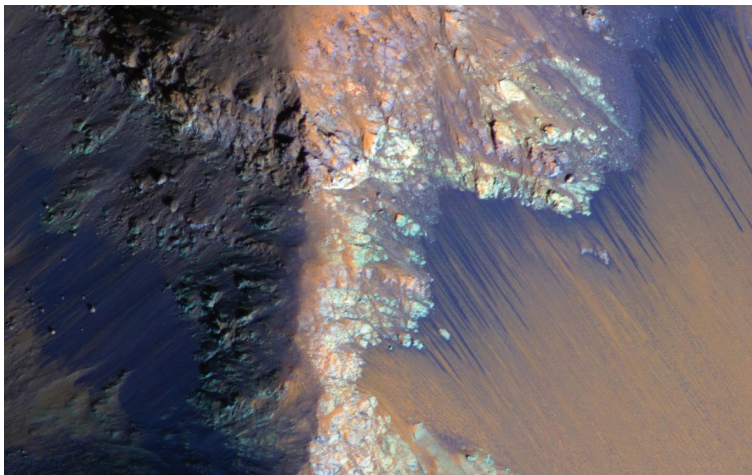
ภาพแสดงพื้นผิวของดาวอังคารบริเวณพื้นที่ Coprates Chasma มีร่องรอยที่เชื่อว่าการไหลของน้ำ
