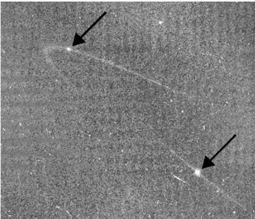
ภาพถ่ายจากยานแคสสินีแสดง Ring Arc ของดวงจันทร์แอนธี (ลูกกลมๆ) และของดวงจันทร์มีโธนี (ลูกทรงรี) [Credit ภาพ: NASA/JPL/SSI]
