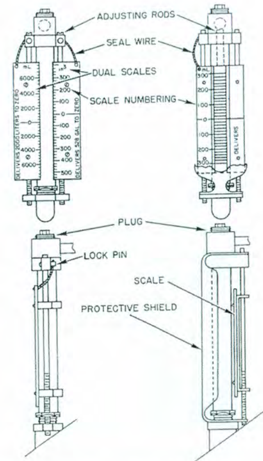
รูปที่ 3 ส่วนวัดระดับของเหลวภายในเครื่องดวงแบบมาตรา (Gage assembly)
