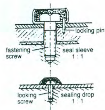
รูปที่ 6 ลักษณะทั่วไปส่วนวัดระดับแบบแผ่นปะกับ
