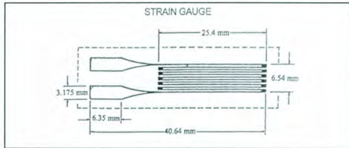
รูปที่ 1 รูปร่างและขนาดของ Strain gauge โดยทั่วไปที่ใช้กับเครื่องชั่งไม่อัตโนมัติ
