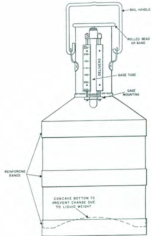
รูปที่ 1 เครื่องตวงแบบมาตราขนาดเล็ก (Standard test measures)
