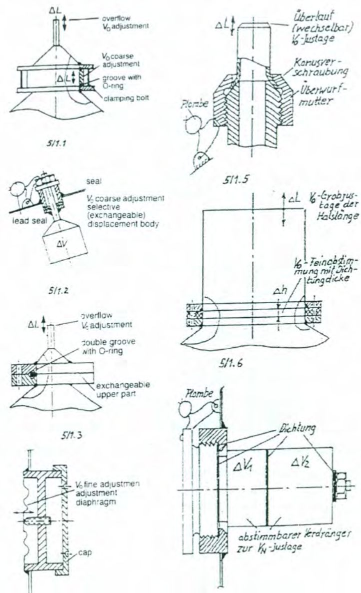
รูปที่ 8 ลักษณะทั่วไปของส่วนปรับแต่งปริมาตรของเครื่องตวงแบบมาตร
