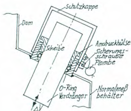
รูปที่ 8 (ต่อ) ลักษณะทั่วไปของส่วนปรับแต่งปริมาตรของเครื่องตวงแบบมาตร
