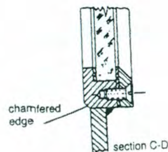
รูปที่ 6 ลักษณะทั่วไปส่วนวัดระดับแบบแผ่นปะกับ
