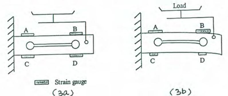
รูปที่ 3 หลักการทำงานของโหลดเซลล์เปรียบเทียบระหว่างสภาวะไม่มีน้ำหนักกระทำกับสภาวะเมื่อมีภาระน้ำหนักกระทำ
