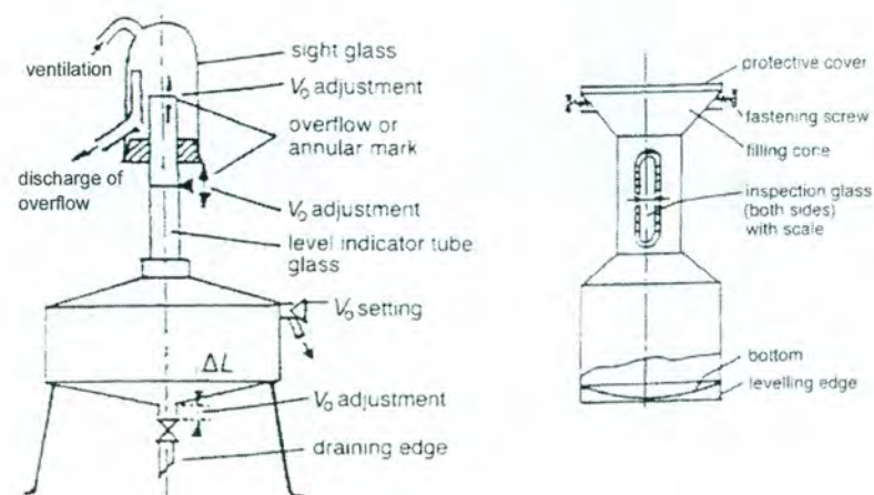
รูปที่ 5 ลักษณะทั่วไปของเครื่องตวงแบบมาตรฐาน
