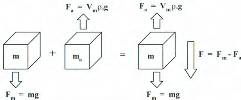
รูปที่ 1 แสดงผลรวมของแรงกระทำต่อมวล m
