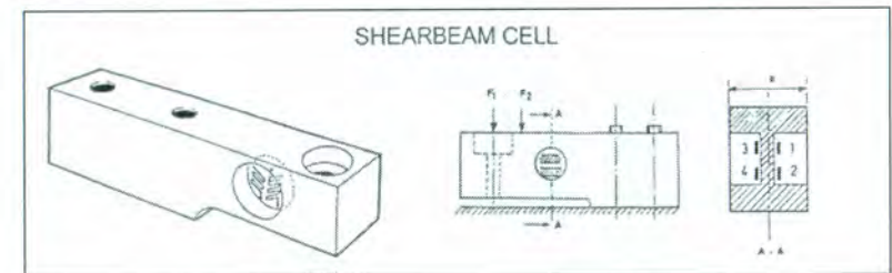
รูปที่ 2 ลักษณะการติดตั้ง Strain gauges บนโหลดเซลล์แบบ Beam cell และ Shearbeam cell
