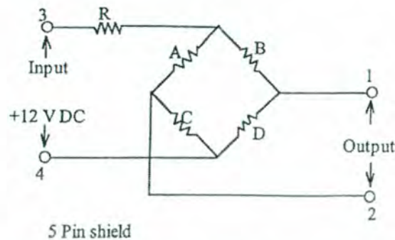
รูปที่ 4 การต่อเชื่อมเป็นวงจรไฟฟ้าวีทสโตนบริด (Wheatstone Bridge Circuit) ของ Stain gauges
