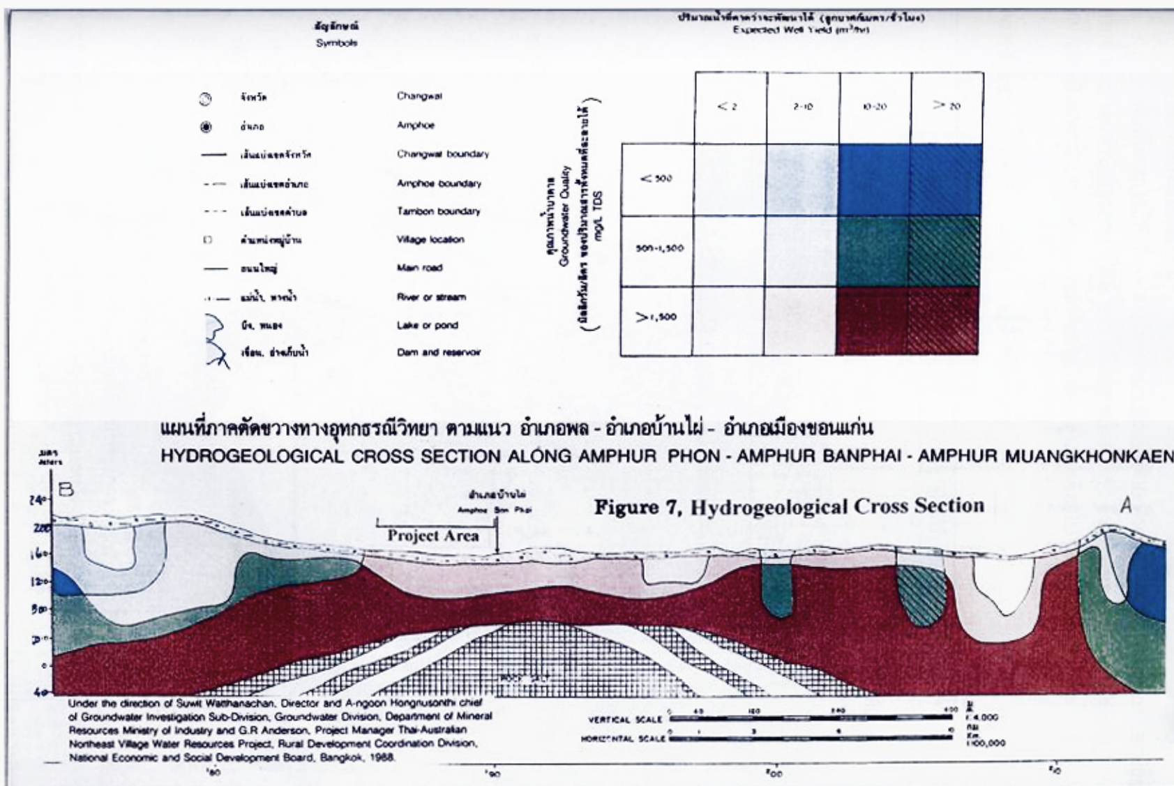
ภาพที่ ๒.๗ แผนที่ภาคตัดขวางทางอุทกวิทยา ตามแนวอำเภอพล-อำเภอบ้านไผ่-อำเภอเมืองขอนแก่น
