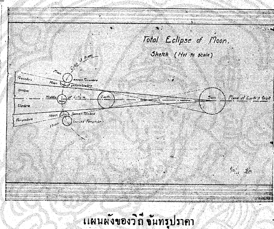
แผนผังของวิถีจันทร์ปรากฏ
