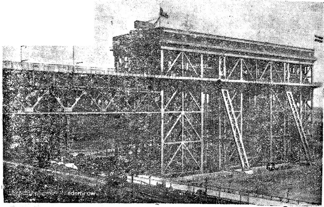
ภาพของคานยกเรือที่ นั้เตรฟโฟ
