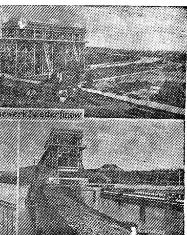
อีกภาพหนึ่งที่แสดงให้เห็น คานยกเรือที่นั้เตรฟโฟ และทันสมัยที่สุดของเยอรมัน ในภาพนี้จะเห็นเรือกำลัง ถูกยกขึ้น และวิ่งเข้าสู่น้ำที่คลอง และเรือที่เกย แม่น้ำเบื้องล่าง
