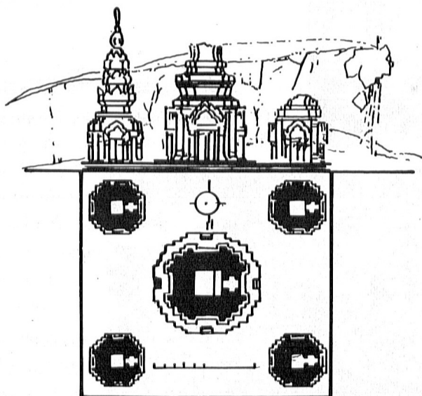
แผนผังปราสาทศรีขรภูมิ
