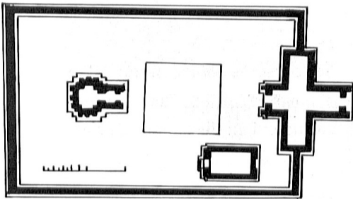
แผนผังปราสาทสระกำแพงน้อย
