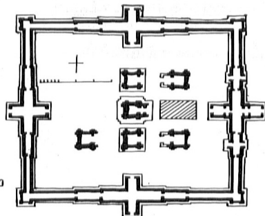
แผนผังปราสาทสระกำแพงใหญ่
