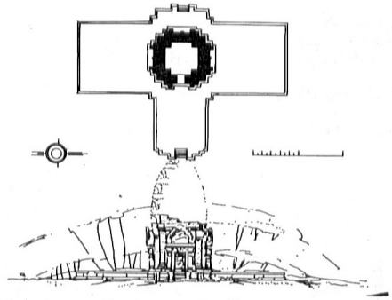
แผนผังปราสาทหินบ้านพลวง
