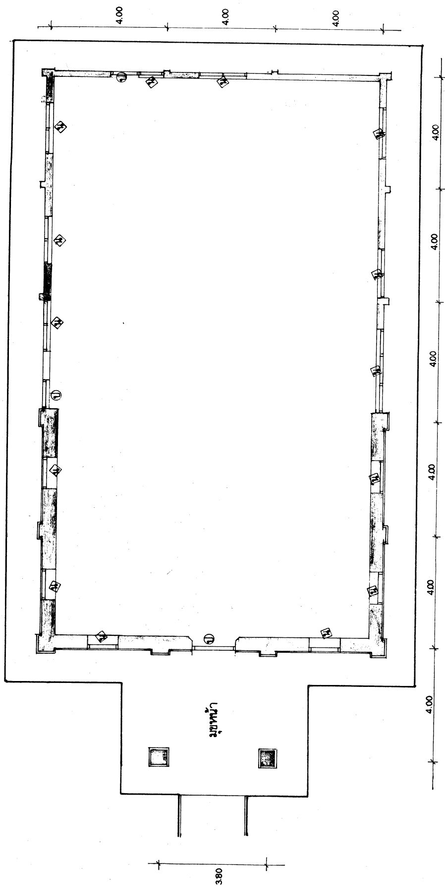
แปลนชั้นล่าง บ้านเลขที่ 179 ถนนเยาวราช
