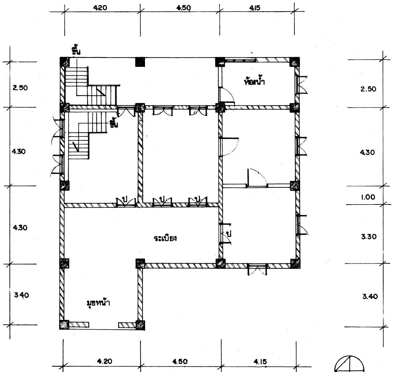
แปลนชั้นล่าง สำนักงานอัยการ
