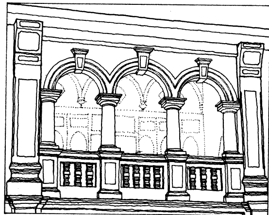
รูปด้านชั้นบน ชุ่มระเบียงโค้งครึ่งวงกลม
