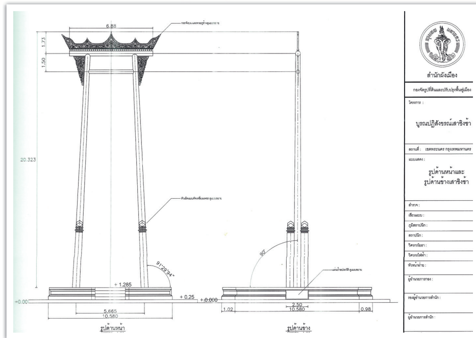
แบบผังการบูรณปฏิสังขรณ์เสาชิงช้ารูปด้านหน้าและด้านข้าง
