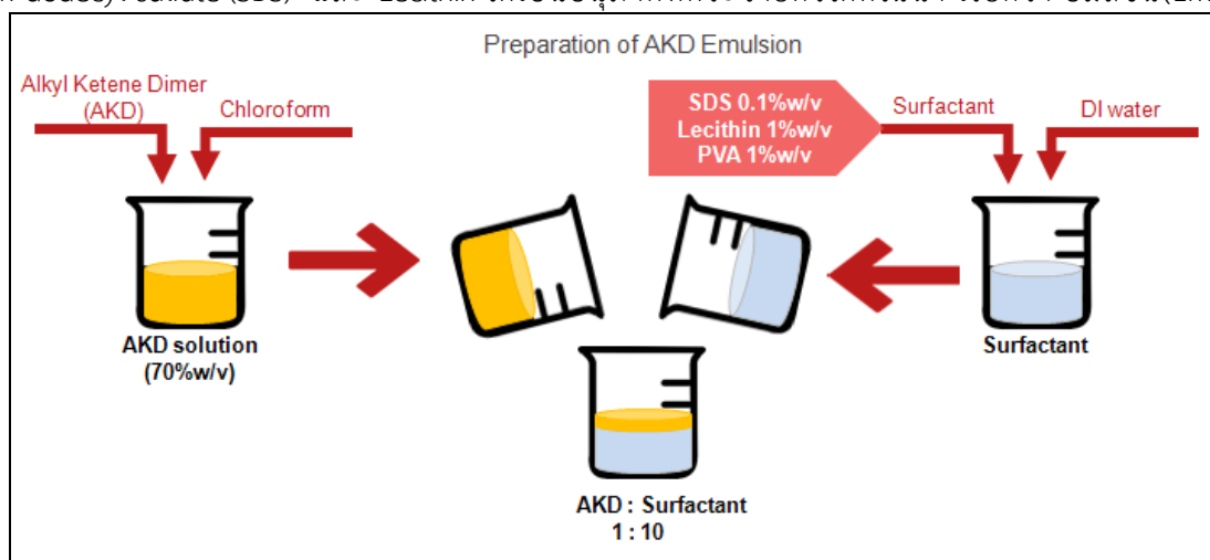
รูปที่ 1 แสดงการเตรียมอนุภาคระดับนาโนของ AKD โดยการห่อหุ้มอนุภาคด้วยสารที่มีขี้ดสูง 3 ชนิด คือ Poly(vinyl alcohol) (PVA), Sodium dodecyl sulfate (SDS) และ Lecithin
