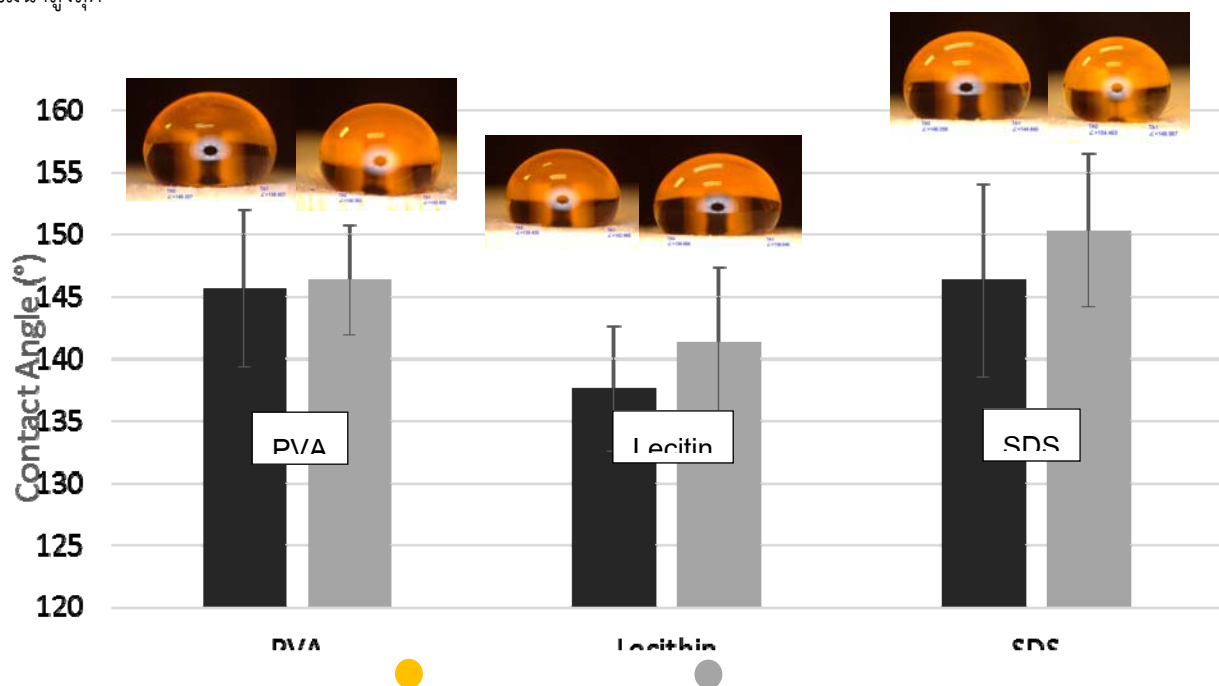
รูปที่ 3 แสดงค่าการต้านการซึมผ่านของเนื้อไม้ที่ผ่านกรรมวิธีปรับปรุงคุณสมบัติจากการเคลือบของอนุภาคระดับนาโนของ AKD โดยการหุ้มผิวอนุภาคด้วยสารที่มีขั้วสูง 3 ชนิด คือ Poly(vinyl alcohol) (PVA),
