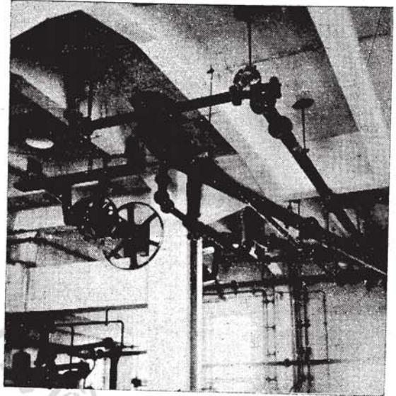
การติดตั้งเครื่องจักรในโรงทำเยื่อ
