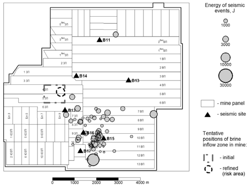
รูป ที่ 6.6.2 แสดงจุดเสี่ยงที่น้ำรั่วเข้าสู่เหมืองใต้ดิน Berezniki-1 จากผลการตรวจวัดความไหวสะเทือน (seismological observations) ในปี ค.ศ. 2006
