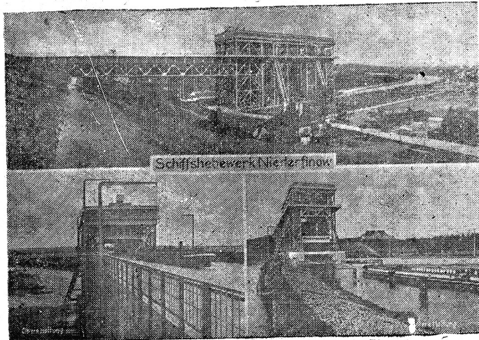
ออกภาพหนึ่งทีแสดงให้เห็นคานยกเรือขึ้นท่าเวลา และทันสมัยที่สุดของเยอรมัน ในภาพนี้จะเห็นเรือกำลังถูกยกขึ้น และวิ่งเข้าสู่วางน้ำที่ทอดไว้ และมองเห็นภาพแม่น้ำเบื้องล่าง.
