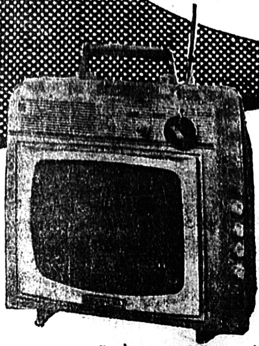
แบบ 12 V.5 กระเป๋าทรงกลมกระทัดรัดเคลื่อนย้ายสะดวก จอภาพ 12 นิ้ว 110 องศา มีหลอด 15 หลอด ใช้ไฟ 110-220V.
