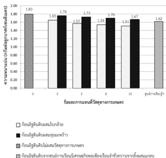
รูปที่ 3 ความหนาแน่นของก้อนอัดดิน
