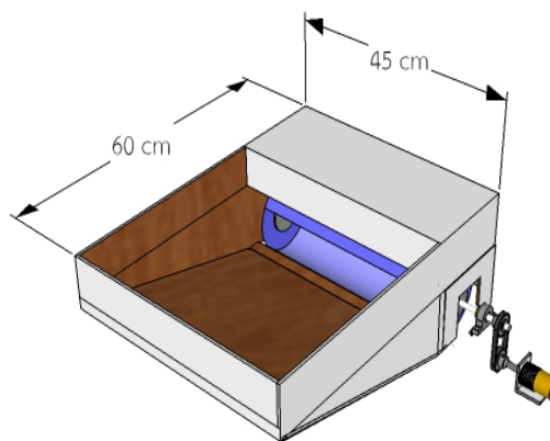
รูปที่ 2 โครงสร้างส่วนช่องใส่ลูกมะนาว
