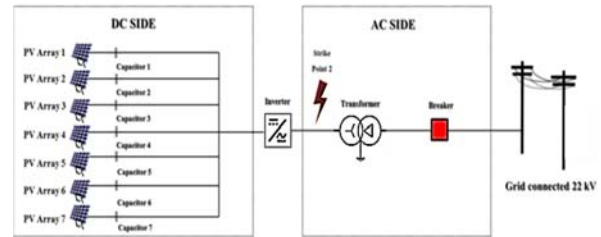
รูปที่ 8 ฟ้าผ่าด้าน AC กรณีไม่มีอุปกรณ์ป้องกันฟ้าผ่า
