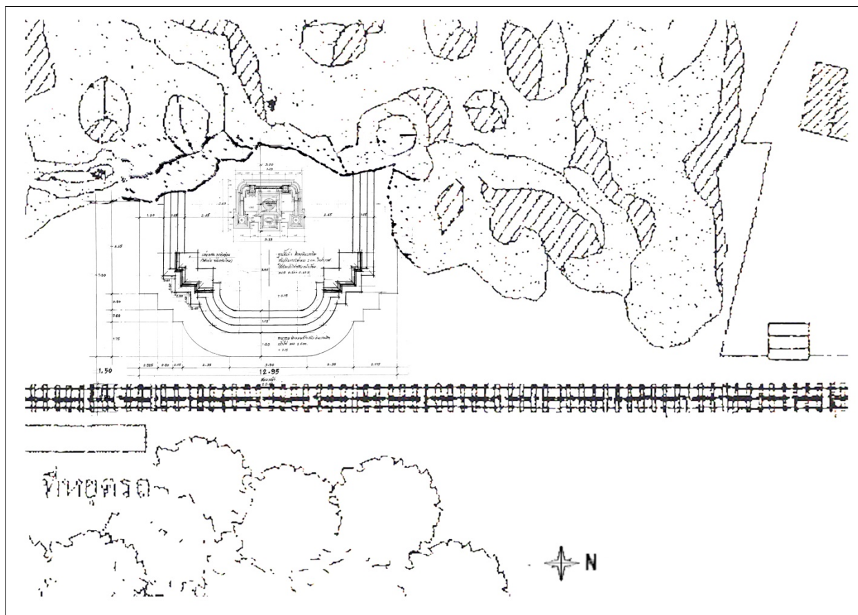
แบบผังบริเวณ พระบรมราชานุสาวรีย์ฯ เห็นข้อจำกัดของพื้นที่ ซึ่งมีขนาดเล็ก และติดกับรางรถไฟ อีกทั้งตั้งอยู่ลึกเข้าไปจากทางเข้าหลักด้านขวาของภาพ ซึ่งจะถูกชะง่อนผาจารึกบังมุมมองอยู่
