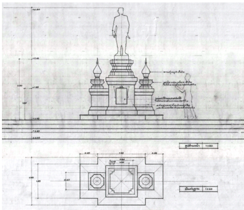
แบบผัง และรูปด้านหน้าพระบรมราชานุสาวรีย์สมเด็จพระนเรศวรมหาราช
