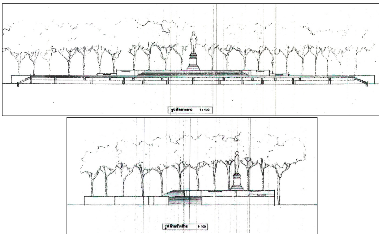
แบบรูปด้านพระบรมราชานุสาวรีย์ฯ
