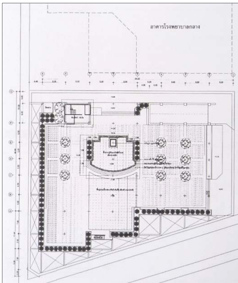
แบบผังพื้นลานประดิษฐานพระบรมราชานุสาวรีย์ฯ
