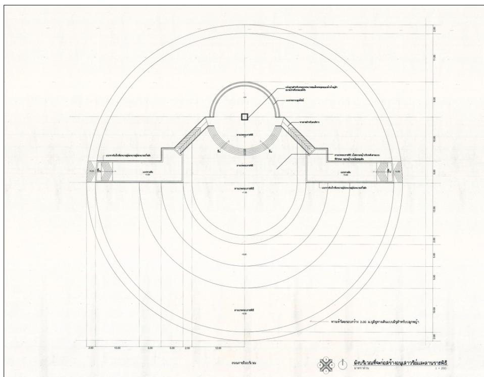
แบบผังบริเวณ แสดงการใช้ประโยชน์พื้นที่ในสถานที่ก่อสร้างฯ
