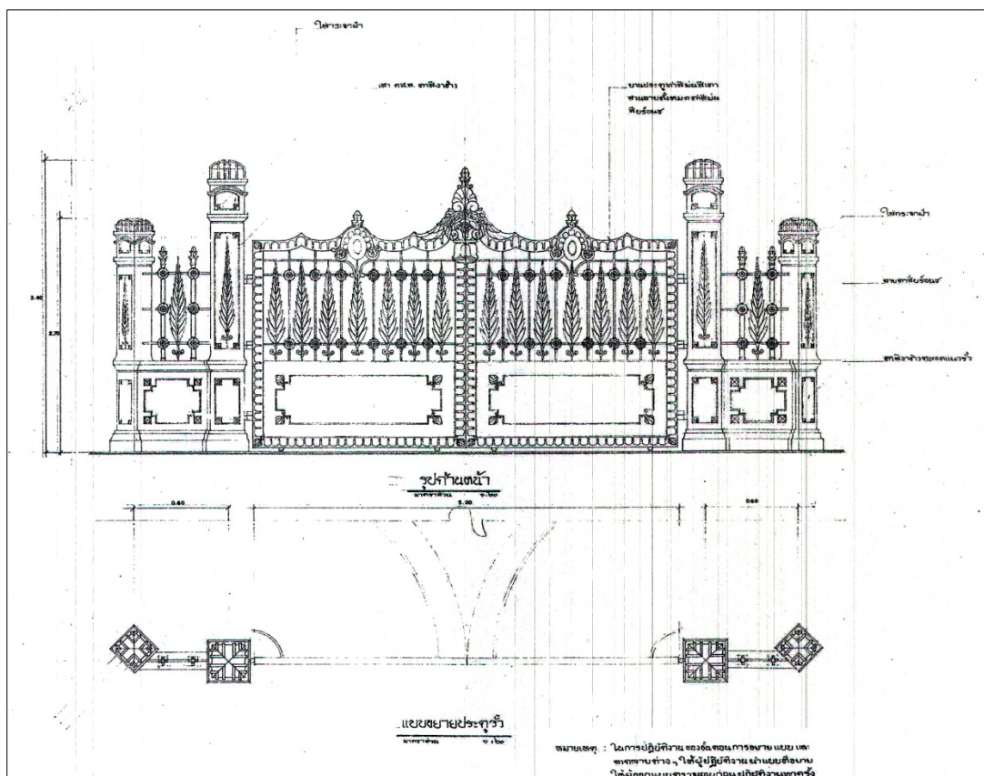
แบบรั้วด้านหน้าพร้อมประตูทางเข้า ได้แนวคิดในการออกแบบมาจากรั้ววังศุโขทัย
