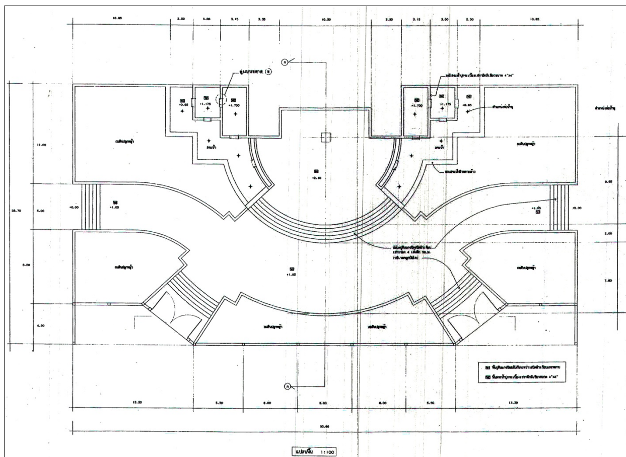
แบบผังพระบรมราชานุสาวรีย์พระบาทสมเด็จพระปกเกล้าเจ้าอยู่หัว แสดงอาณาบริเวณด้านหน้าอาคารประชาธิปกศักดิ์เดช ซึ่งเป็นจุดที่ตั้งพระบรมราชานุสาวรีย์ฯ อันเป็นมุมมองที่เห็นได้ชัดเจน สง่างาม โดยใช้อาคารเป็นฉากหลัง
