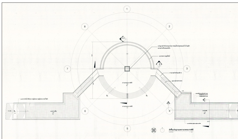
แบบผังพระบรมราชานุสาวรีย์ฯ แสดงการเข้าถึงแท่นประดิษฐาน
