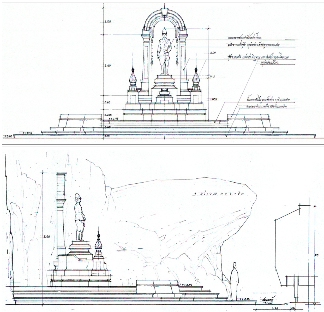
แบบรูปด้านแท่นฐานพระบรมราชานุสาวรีย์ฯ
