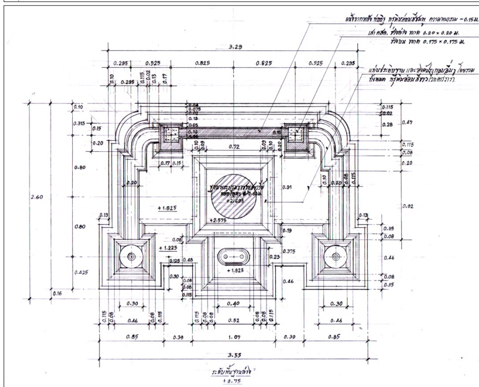
แบบผังแท่นฐานพระบรมราชานุสาวรีย์ฯ
