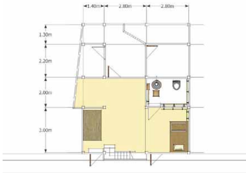
แปลนชั้น 1
