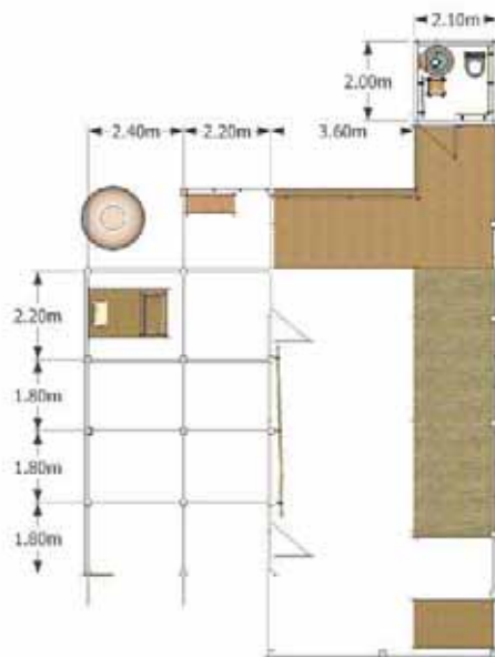
แปลนชั้น 1
