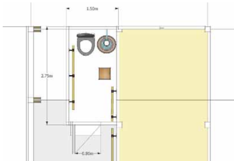
แปลนขยายห้องน้ำ
