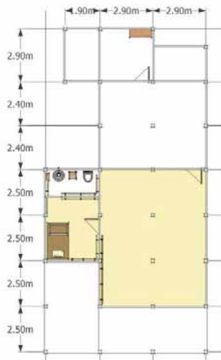
แปลนชั้น 1
