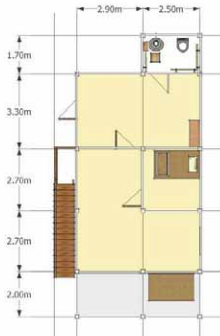
แปลนชั้น 1
