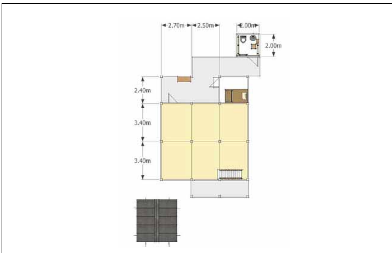
แปลนชั้น 1
