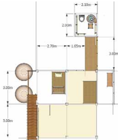
แปลนชั้น 1
