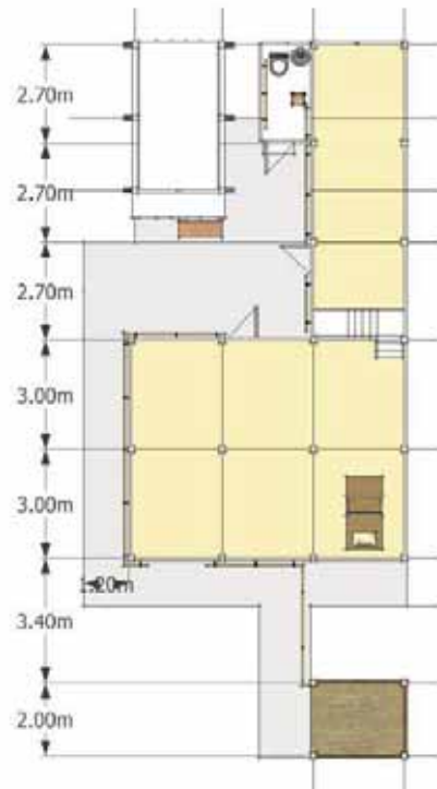
แปลนชั้น 1
