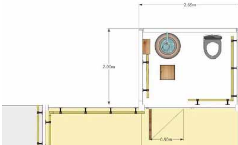
แปลนขยายห้องน้ำ
