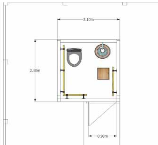
แปลนขยายห้องน้ำ
