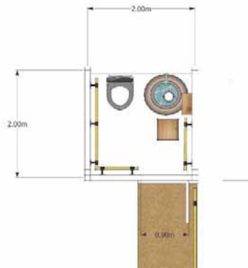
แปลนขยายห้องน้ำ
