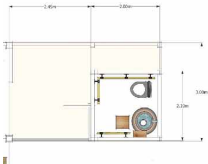
แปลนขยายห้องน้ำ
