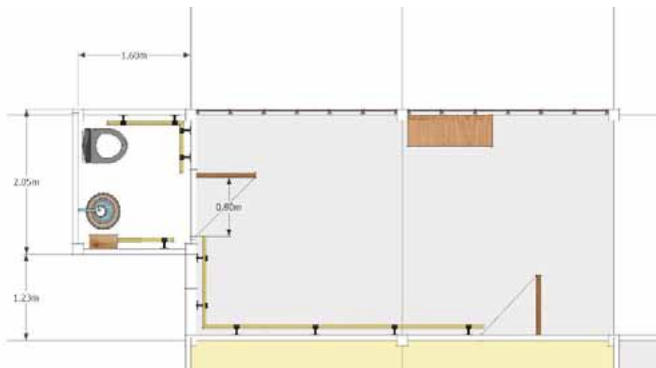
แผนขยายห้องน้ำ
