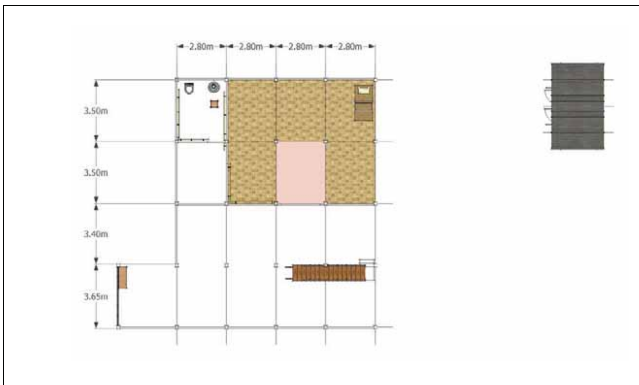
แปลนชั้น 1
