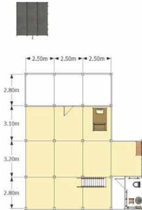
แปลนชั้น 1
