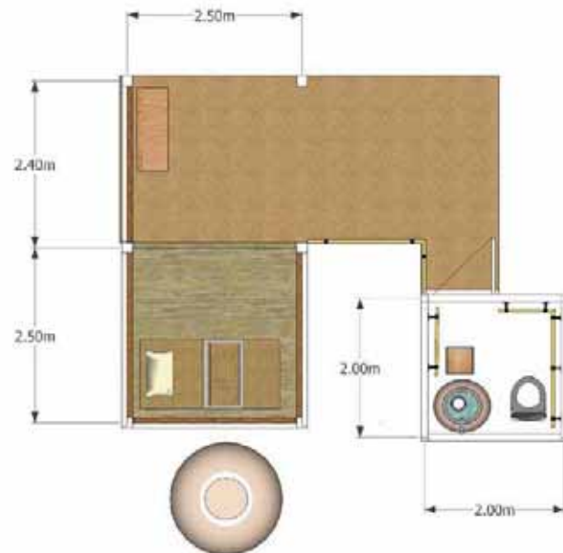
แปลนชั้น 1
