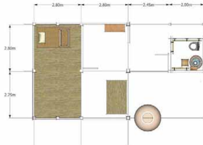
แปลนชั้น 1
