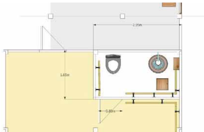
แปลนขยายห้องน้ำ
