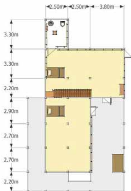
แปลนชั้น 1
