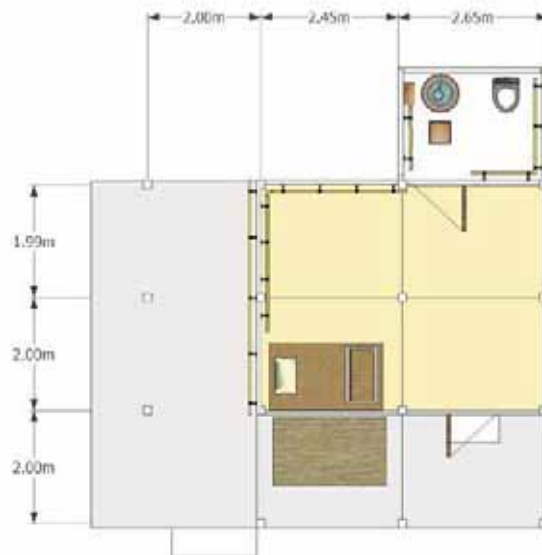
แปลนชั้น 1
