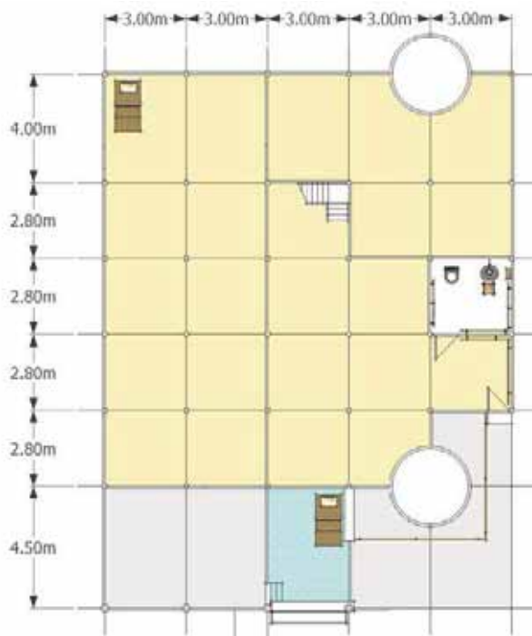
แปลนชั้น 1
