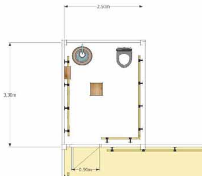
แปลนขยายห้องน้ำ
