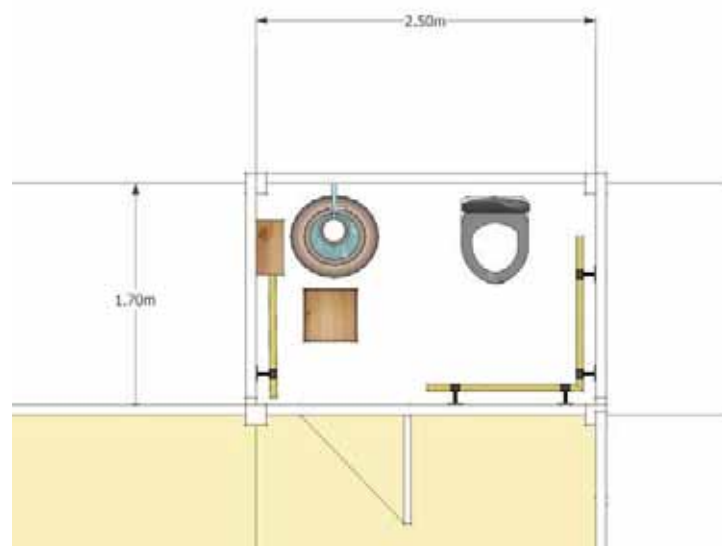
แปลนขยายห้องน้ำ
