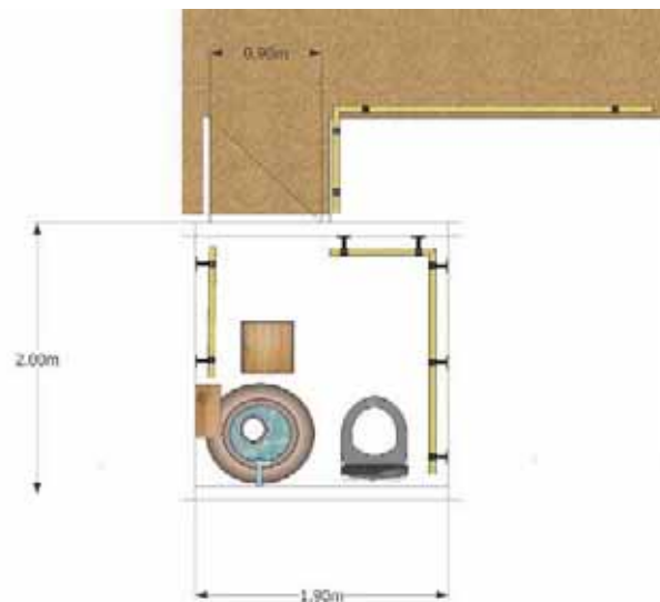
แปลนชั้น 1
