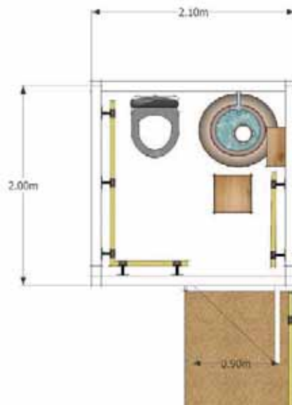
แปลนขยายห้องน้ำ
